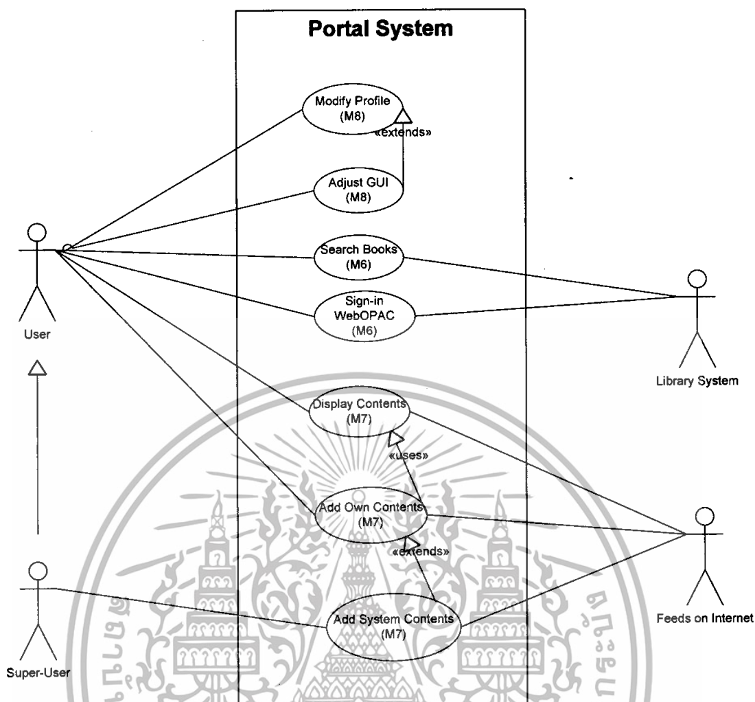
รูปที่ 3.5 Use Case Diagram ของระบบ: โมดูล 6, 7, 8
