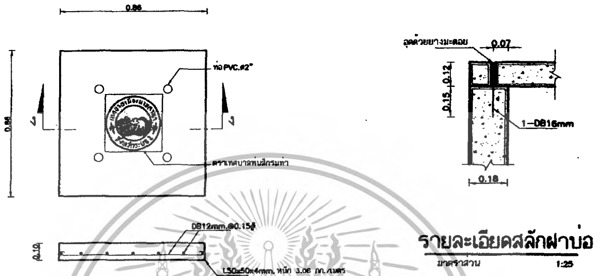
แบบขยายฝาบ่อพัก มาตรฐาน 1:25 รูปที่ จ.12 ฝาบ่อพัก
