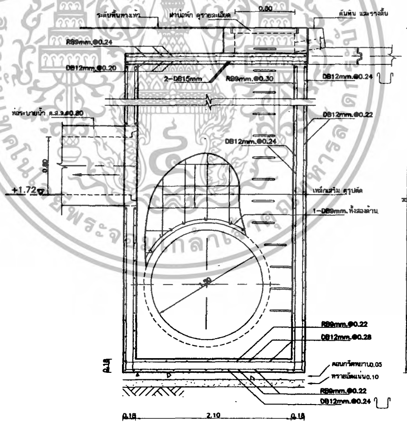
รูปตัด ก-ก มาตราส่วน 1:50
