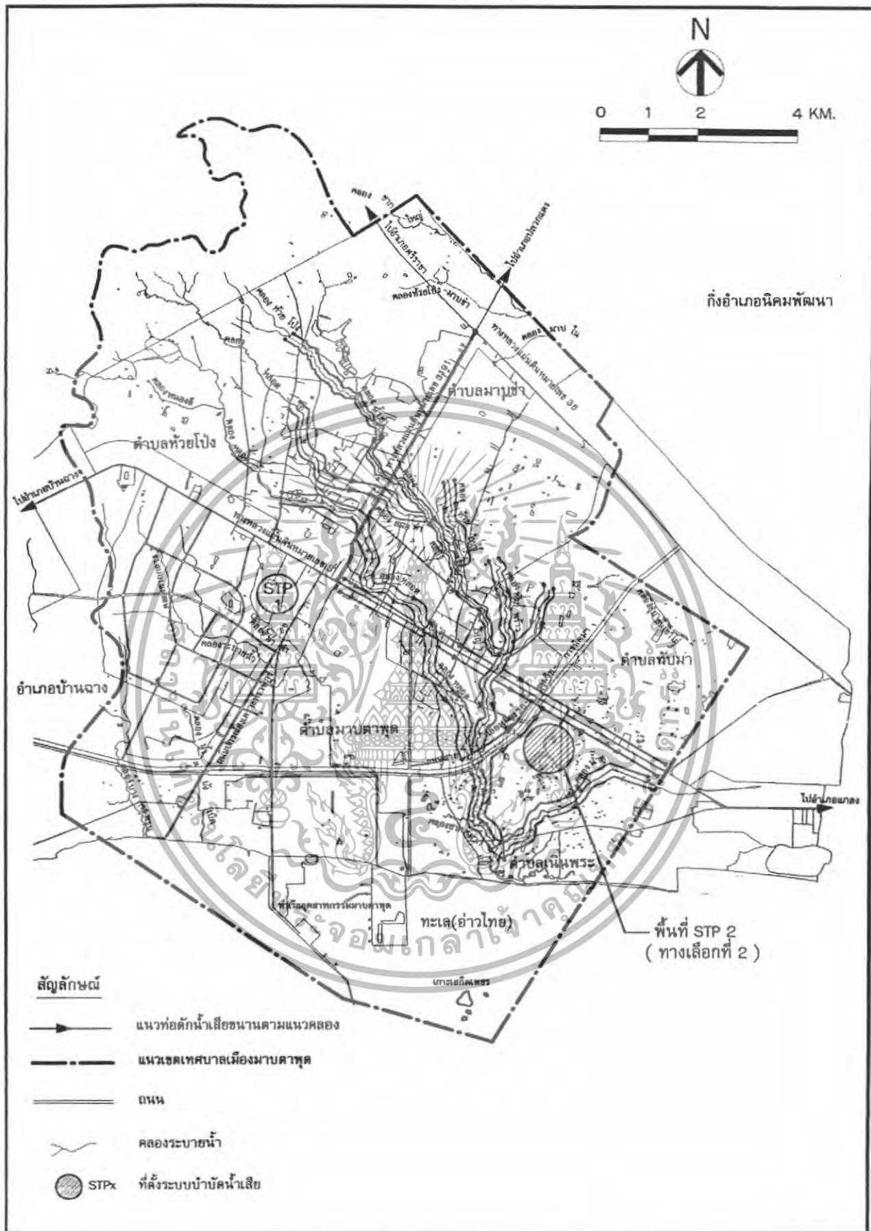
รูปที่ 3.5 แนวทางการวางท่อคักน้ำเสียนานตามแนวคลอง และที่ตั้ง STP2 (ทางเลือกที่ 2) เอกสารนี้เป็นเอกสารที่สงวนไว้สำหรับการใช้งานเพื่อการศึกษาเท่านั้น ไมออนุญาตให้นำไปใช้ประโยชน์ด้านการค้า ไม่ว่าจะกรณีใดๆทั้งสิ้น อีกทั้งห้ามมิให้ดัดแปลงเนื้อหา และต้องอ้างอิงถึงเจ้าของเอกสารทุกครั้งที่มีการนำไปใช้
