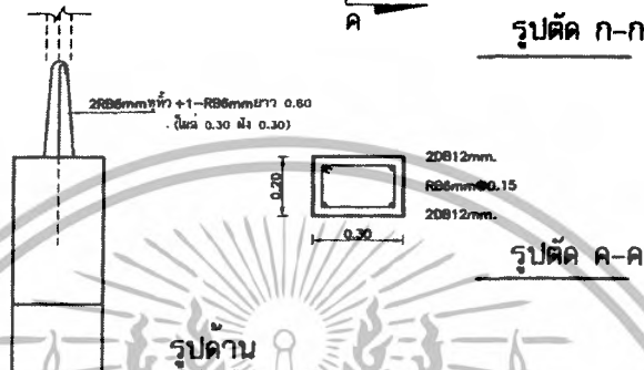
แบบขยายฐานรองรับรอยต่อท่อ มาตราส่วน 1:25
