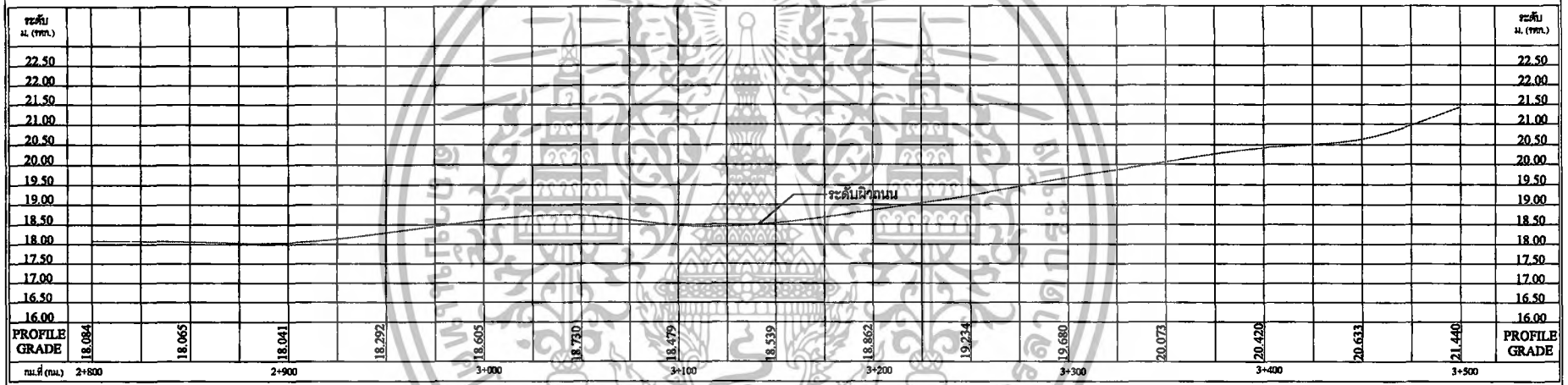
รูปที่ 4.58 รูปตัดตามยาวริมถนนเขตหิน-เขาไฟ กม.ที่ 2+800 ถึง กม.ที่ 3+500
