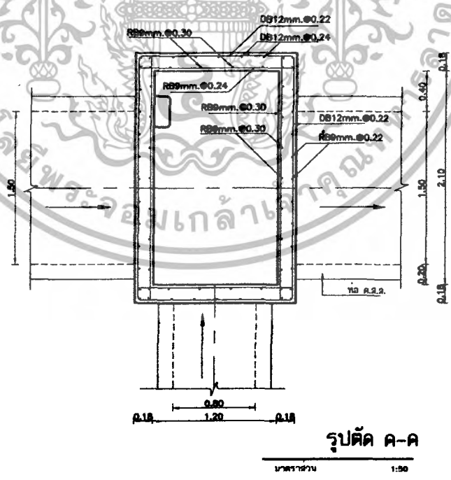
รูปที่ จ.11 รูปตัด(ค-ค)บ่อพัก
