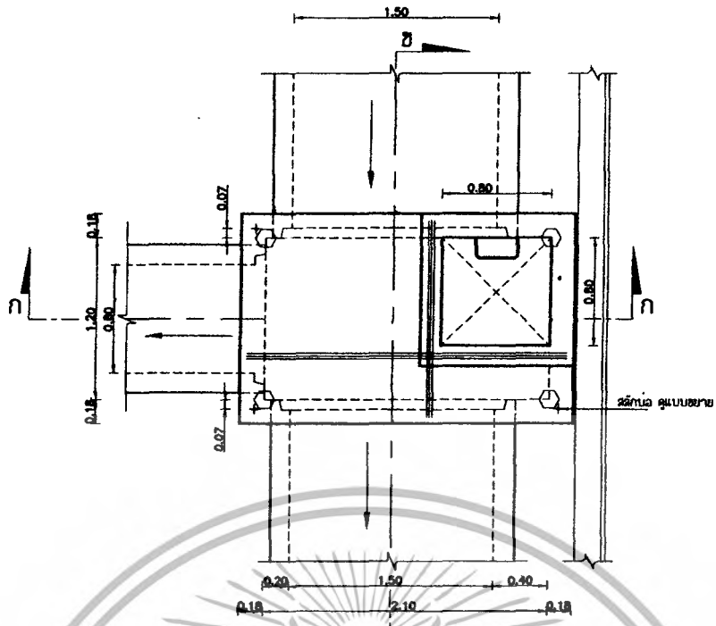
แบบ มาตราส่วน 1:50
