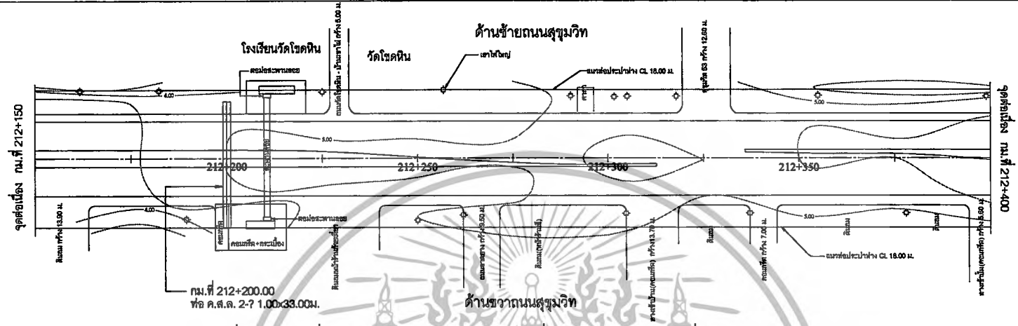
รูปที่ 4.6 แผนที่ผังค่าระดับถนนสุขุมวิท กม.ที่ 212+150 ถึง กม.ที่ 212+400
