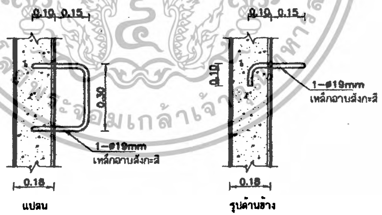
รายละเอียดบันไดเหล็ก มาตรฐาน 1:25
