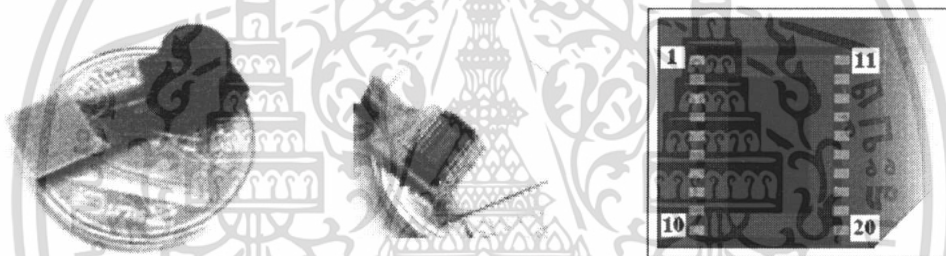
รูปที่ 3.1 โมดูลกล้องและการจัดเรียงขาของกล้อง E700
