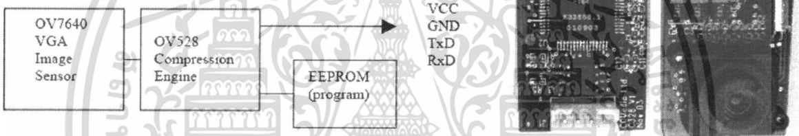
รูปที่ 3.5 บล็อกไดอะแกรมของกล้อง C328R
