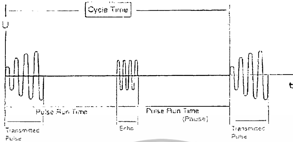
รูปที่ 2.30 อุลตราโซนิกเซ็นเซอร์, วงจรที่เปลี่ยนแปลงได้
