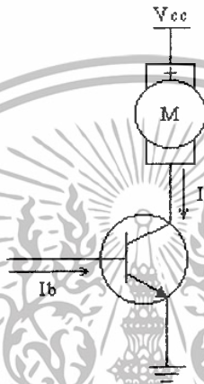
รูปที่ 2.14 วงจรสวิตช์การนำทรานซิสเตอร์ มาเป็นสวิตช์ควบคุมมอเตอร์
