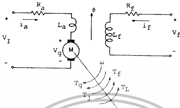
รูปที่ 2.3 แสดง โมเดลของดีซีมอเตอร์แบบฟีดแบ็คกระตุ้น
