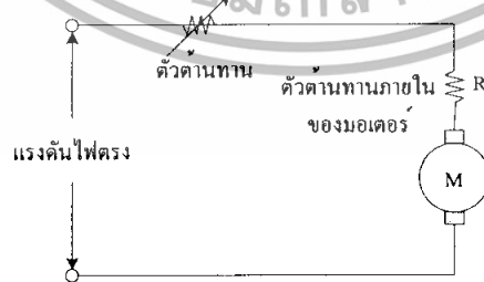
รูปที่ 2.4 วงจรควบคุมความเร็วของมอเตอร์กระแสตรงแบบใช้ตัวต้านทานอนุกรม
