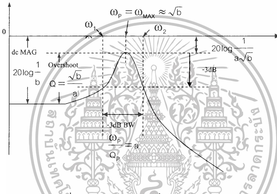
รูปที่ 2.20 การตอบสนองความถี่ของ Quadratic poles
