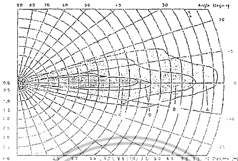
รูปที่ 2.32 อุตตราโซนิคเซ็นเซอร์, คุณลักษณะการตรวจจับ
