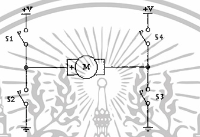
รูปที่ 2.7 วงจร H-Bridge Switching
