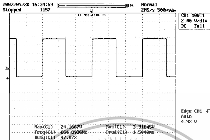
รูปที่ 6.7 แสดงการทดสอบสัญญาณที่ออกมาจาก TLP250 เมื่อที่ไมโครคอนโทรลเลอร์มี input เป็น Forward (1)
