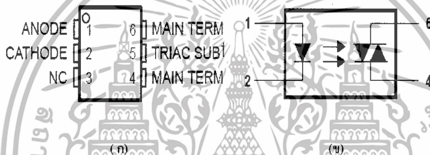
รูปที่ 3.20 ลักษณะภายนอกและวงจรภายในของ ไทรแอก
