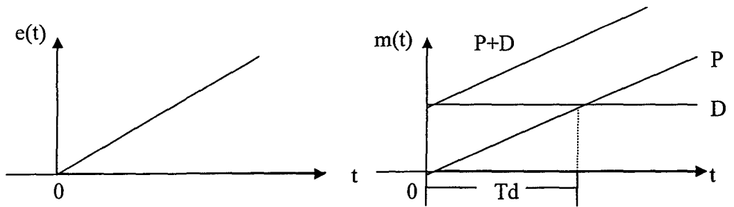
รูปที่ 2.13 การควบคุมแบบพีดี
