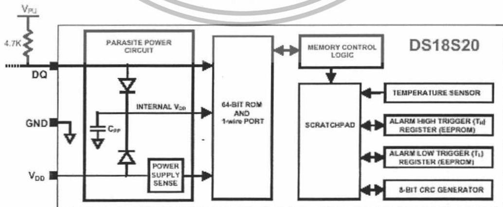
รูปที่ 2.27 โครงสร้างภายในของไอซีตรวจจับอุณหภูมิ DS18S20
