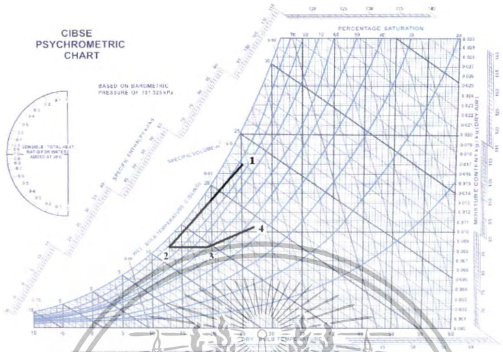
รูปที่ 3-14 แผนภูมิไซโครเมตริกแสดงกระบวนการปรับสภาวะจาก 1-4 เมื่ออากาศออกจากชุดฮีตเตอร์ที่อุณหภูมิ 19.2^{\circ}C
