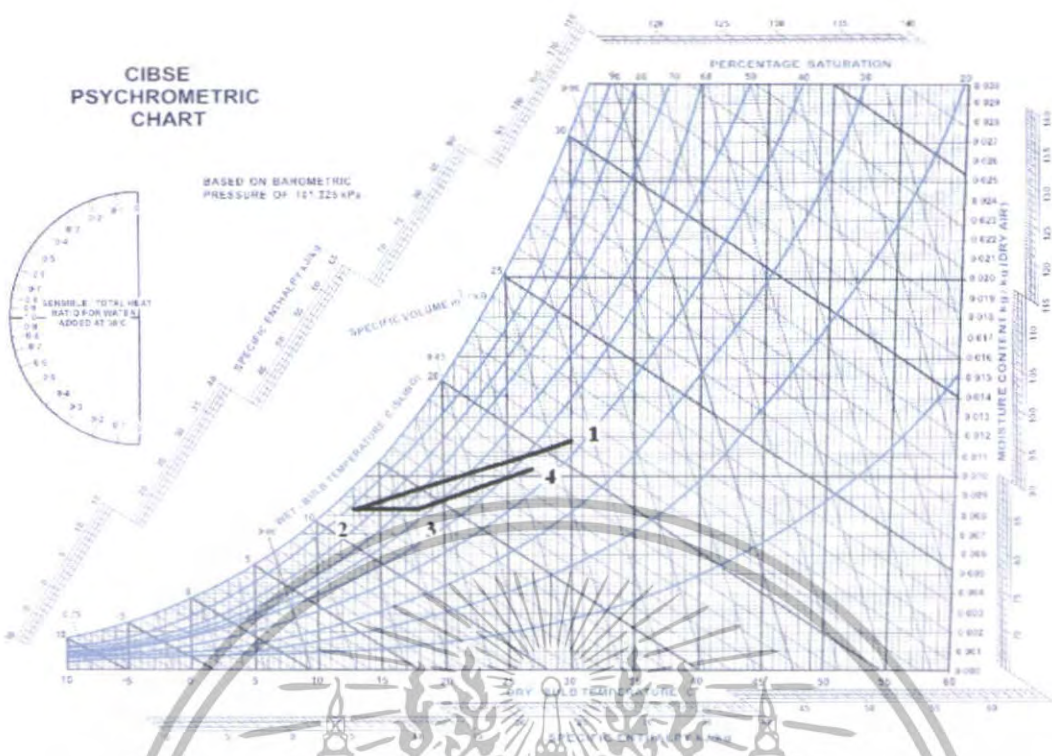
รูปที่ 3-2 แผนภูมิไซโครเมตริกแสดงกระบวนการปรับสภาวะจาก 1-4 เมื่ออากาศออกจากชุดฮีตเตอร์ที่อุณหภูมิ 18°C
