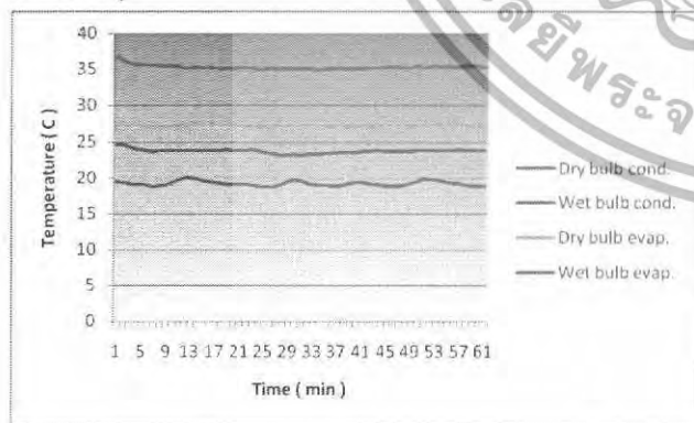
กราฟที่ 6-1 แสดงสถานะที่สมดุลระหว่างการทดลองที่ 1
