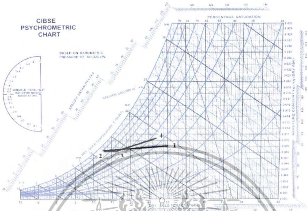
รูปที่ 3-5 แผนภูมิไซโครเมตริกแสดงกระบวนการปรับสภาวะจาก 1-4 เมื่ออากาศออกจากชุดฮีตเตอร์ที่อุณหภูมิ 16.5°C
