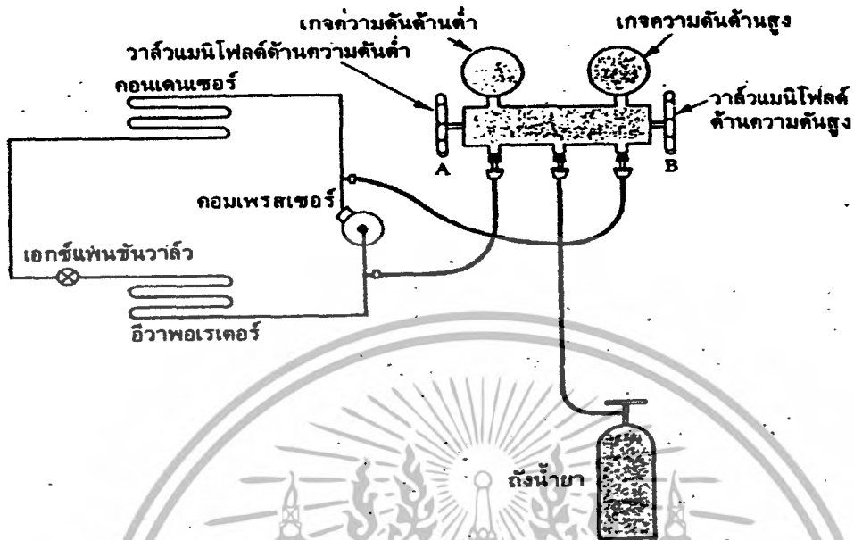
รูปที่ 4-34 การชาร์จน้ำยาในสถานะก๊าซเข้าในระบบทางด้านความดันต่ำ
