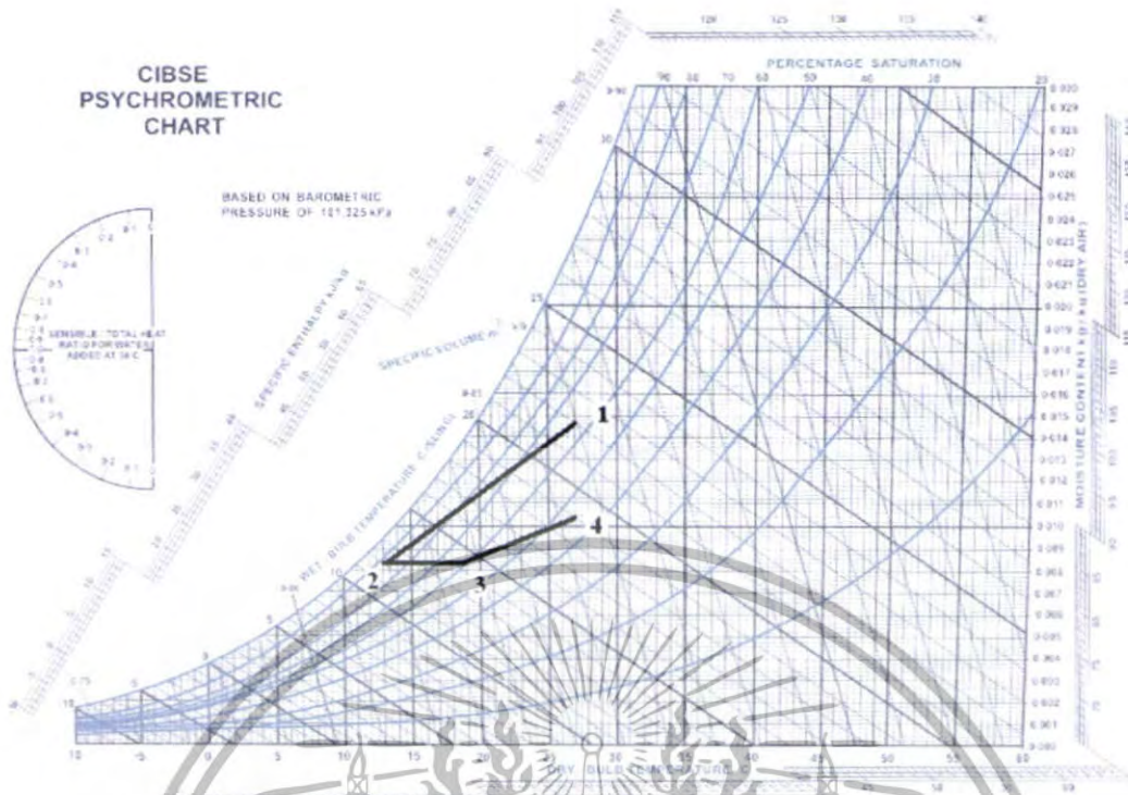
รูปที่ 3-8 แผนภูมิไซโครเมตริกแสดงกระบวนการปรับสภาวะจาก 1-4 เมื่ออากาศออกจากชุดฮีตเตอร์ ที่อุณหภูมิ 18.5°C
