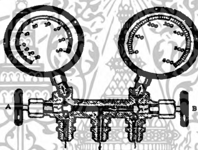
รูปที่ 4-30 วาล์ว A อยู่ในตำแหน่งปิด วาล์ว B อยู่ในตำแหน่งเปิด
