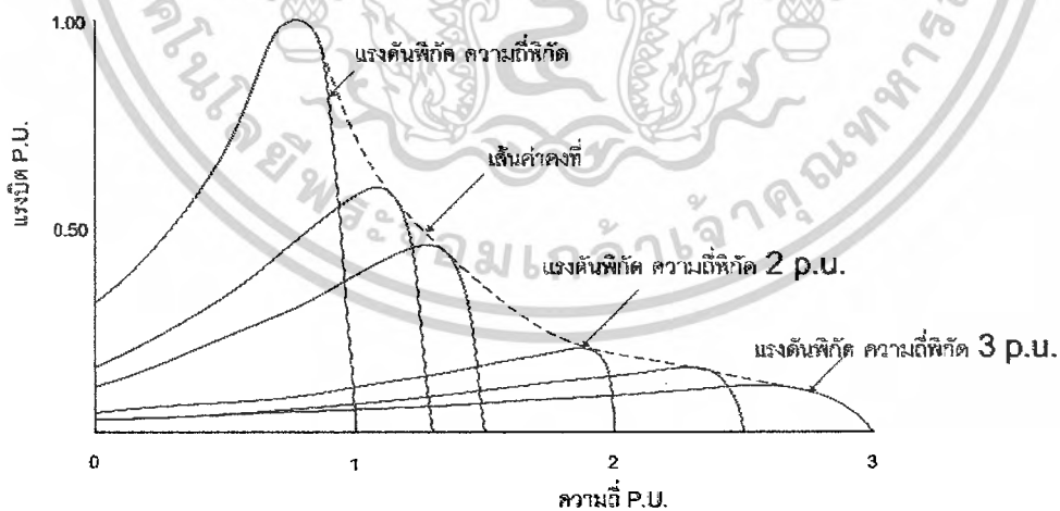
ภาพที่ 2.9 กราฟความสัมพันธ์แรงบิด - ความเร็ว เมื่อเปลี่ยนแปลงความถี่
