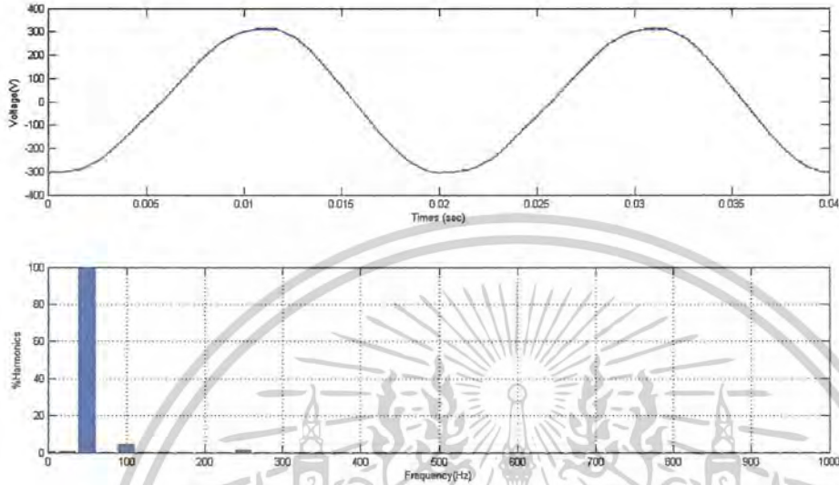
ภาพที่ 8.1 ผลรวมของความถี่มูลฐานกับความถี่ฮาร์โมนิกส์ที่มีลำดับเฟสบวก และสเปกตรัมของผลรวมความถี่มูลฐานกับความถี่ฮาร์โมนิกส์อันดับที่ 2 ที่เปอร์เซ็นต์ความเพี้ยนคิกคาไฟฟ้า 5 เปอร์เซ็นต์
