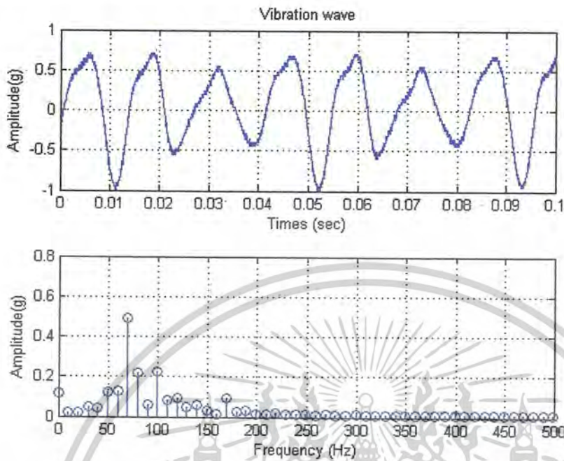
ภาพที่ 8.39 แสดงสเปกตรัมของการสั่นสะเทือนที่เกิดจากแรงดันไฟฟ้าสามเฟสไม่สมดุล
