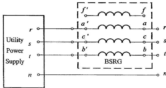
ภาพที่ 4.7 แผนภูมิการต่ออันดับ k^{\text{th}} ฮาร์โมนิกส์ศักดาไฟฟ้าลำดับเฟสลบ
