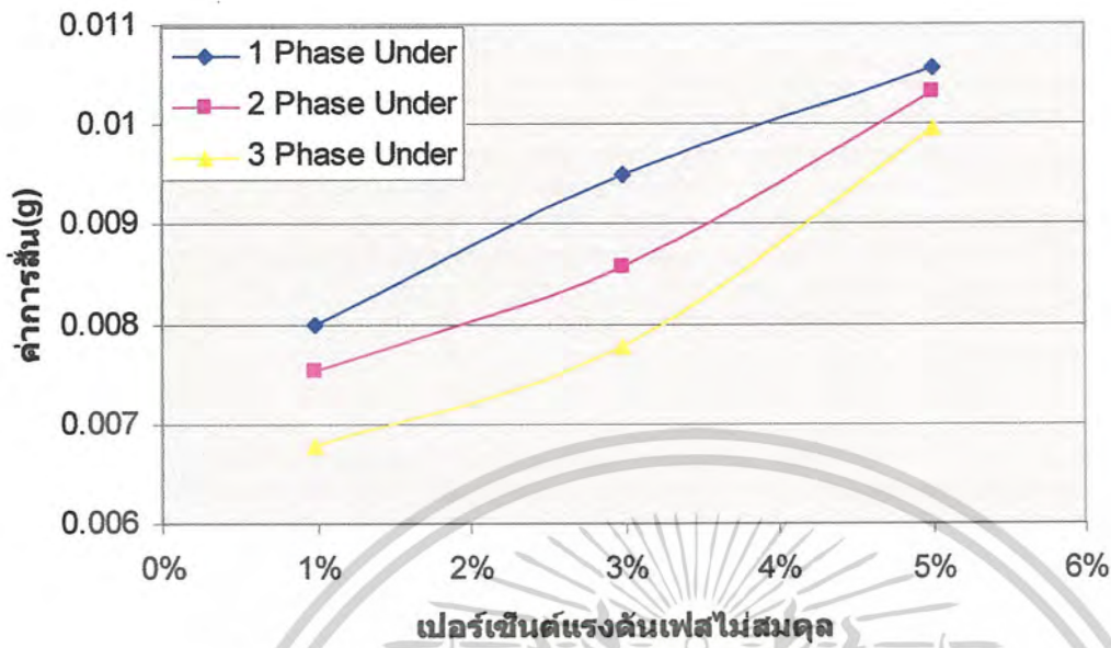
ภาพที่ 8.58 แสดงการเปรียบเทียบผลการสั่นเมื่อแรงดันสามเฟสไม่สมดุลแบบแรงดันต่ำกว่าแบบ 1 เฟส 2 เฟส และ 3 เฟส เมื่อเพิ่มเปอร์เซ็นต์ของแรงดันเฟสไม่สมดุล
