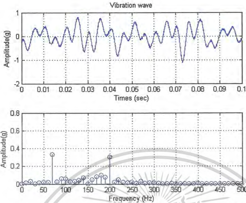
รูปที่ 8.85 แสดงสเปกตรัมของการสั่นสะเทือนเมื่อได้รับฮาร์มอนิกส์ลำดับที่ 5 ที่มีค่าความเพี้ยนตักตาไฟฟ้า 30 เปอร์เซ็นต์ และมีการเรียงลำดับเฟสในทิศทางบวก
