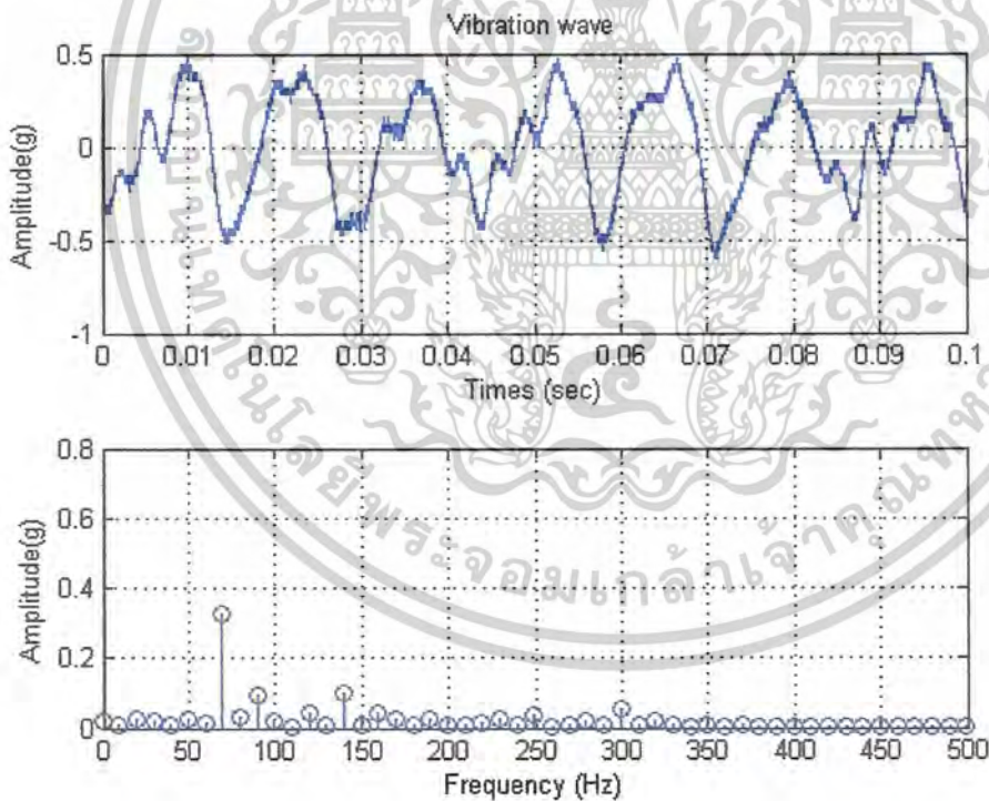
รูปที่ 8.86 แสดงสเปกตรัมของการสั่นสะเทือนเมื่อได้รับฮาร์มอนิกส์ลำดับที่ 5 ที่มีค่าความเพี้ยนตักตาไฟฟ้า 30 เปอร์เซ็นต์ และมีการเรียงลำดับเฟสในทิศทางลบ
