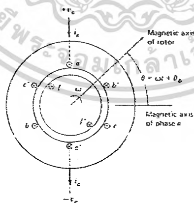
ภาพที่ 3.6 เครื่องจักรกลไฟฟ้าซึ่งโครนิสแบบขั้วนอนขาลื่น
