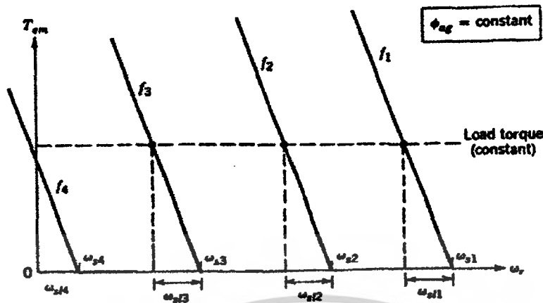
ภาพที่ 2.13 กราฟคุณลักษณะของแรงบิด - ความเร็ว ที่ค่าสลลิปต่ำ
