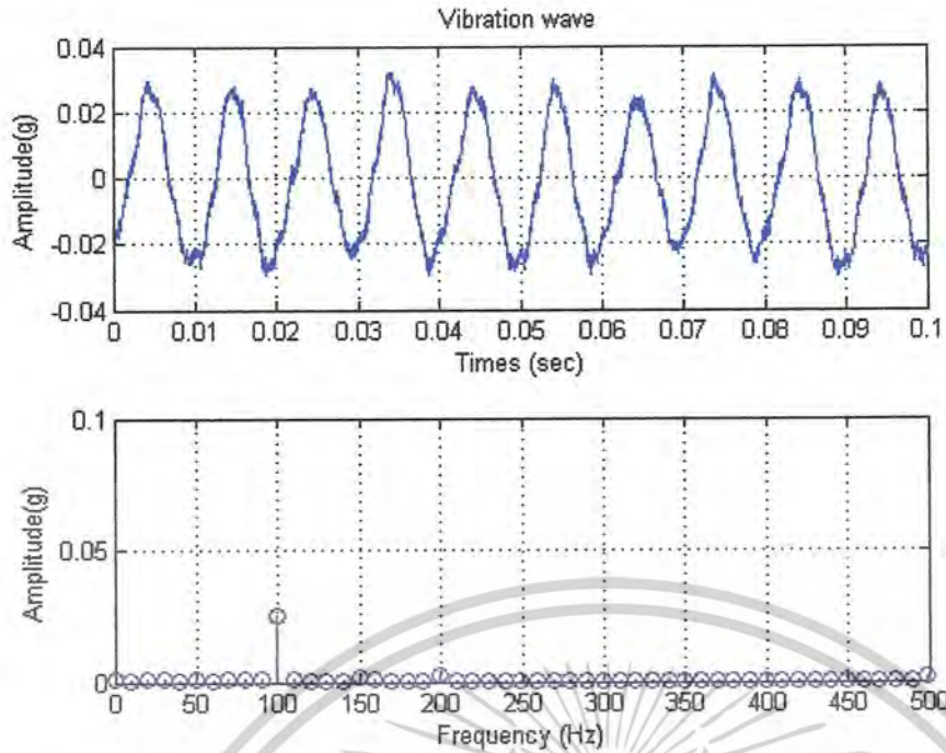
ภาพที่ 8.32 แสดงสเปกตรัมของการสั่นสะเทือนที่เกิดจากแรงดันไฟฟ้าเฟส a คงที่ 220V เฟส b 227V และเฟส c 240V (205%)
