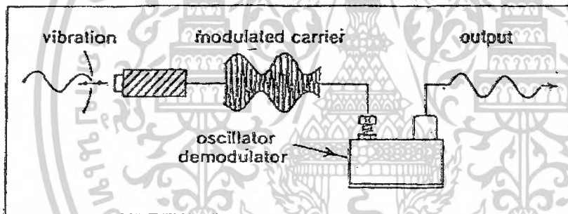
ภาพที่ ก1 การทำงานของหัวตรวจวัดประเภทระยะทาง
