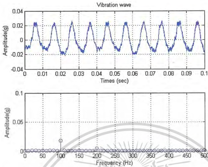
ภาพที่ 8.26 แสดงสเปกตรัมของการสั่นสะเทือนที่เกิดจากแรงดันไฟฟ้าเฟส a และ b คงที่ 220V เฟส c 236V (105%)
