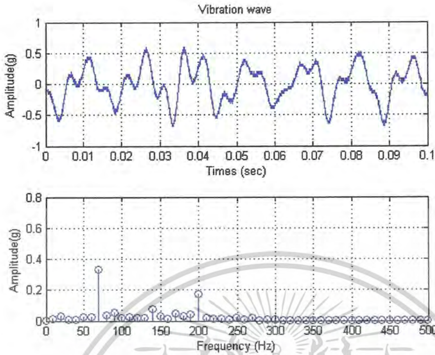
รูปที่ 8.33 แสดงสเปกตรัมของการสั่นสะเทือนเมื่อได้รับฮาร์มอนิกลำดับที่ 5 ที่มีค่าความเพี้ยนตกคาไฟฟ้า 15 เปอร์เซ็นต์ และมีการเรียงลำดับเฟสในทิศทางบวก
