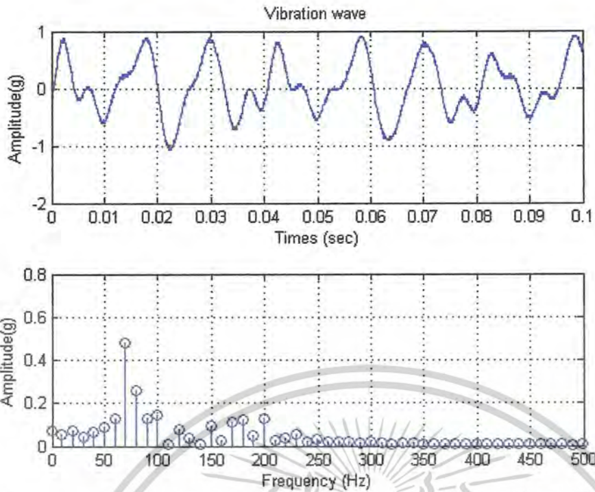
รูปที่ 8.75 แสดงสเปกตรัมของการสั่นสะเทือนเมื่อได้รับฮาร์มอนิกส์ลำดับที่ 5 ที่มีค่าความเพี้ยนศักดาไฟฟ้า 15 เปอร์เซ็นต์ และมีการเรียงลำดับเฟสในทิศทางบวก
