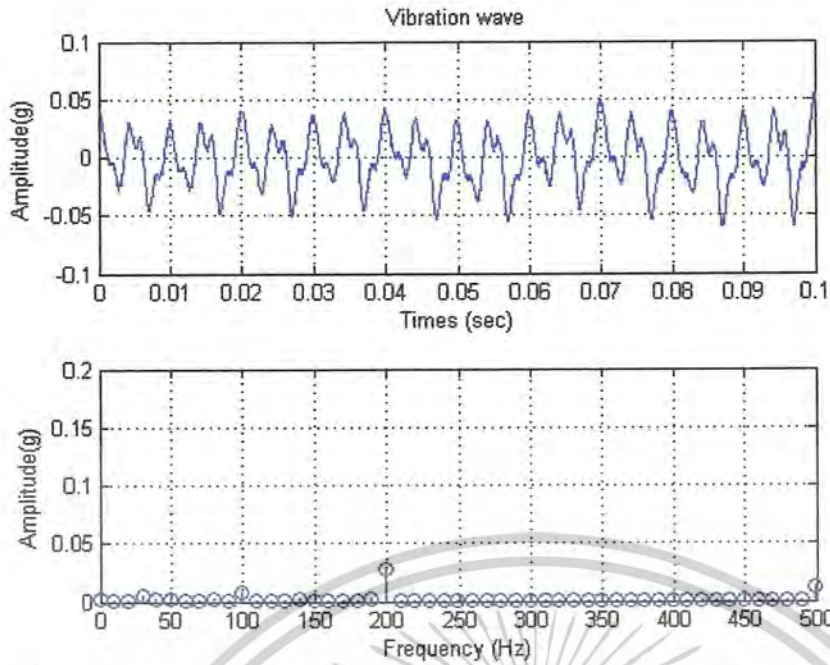
ภาพที่ 8.67 แสดงสเปกตรัมของการสั่นสะเทือนเมื่อได้รับฮาร์มอนิกส์ลำดับที่ 5 ที่มีค่าความถี่ขนาดไฟฟ้า 15 เฮอร์เซ็นต์ และมีการเรียงลำดับเฟสในทิศทางบวก
