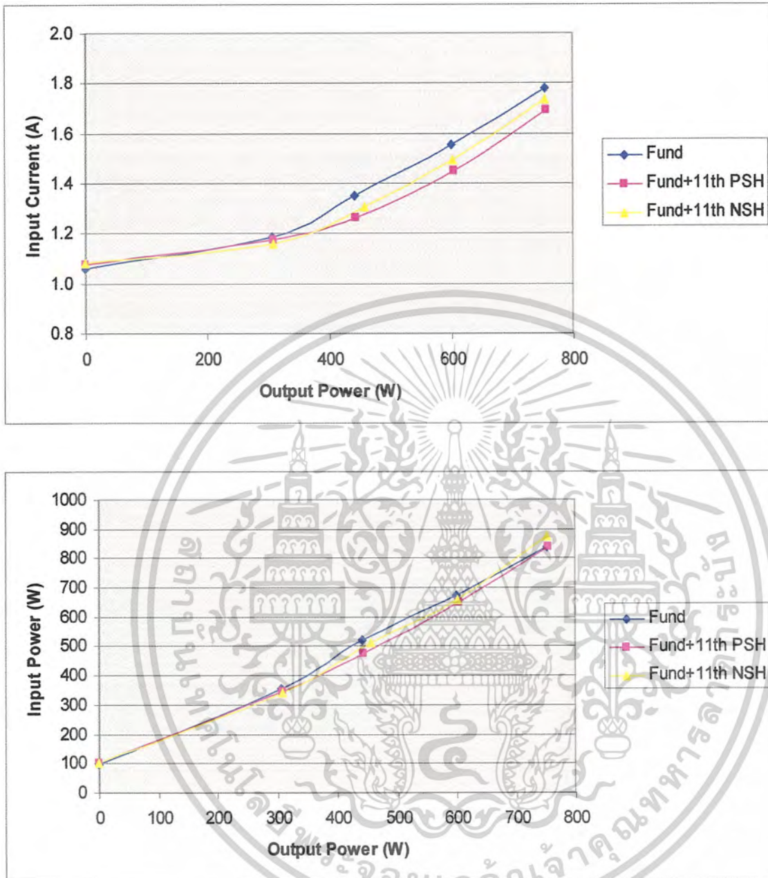
ภาพที่ 8.18 กระแสไฟฟ้าและกำลังไฟฟ้าป้อนเข้ามอเตอร์ไฟฟ้าเหนี่ยวนำขนาด 1 แรงม้า ในกรณีแหล่งจ่ายมีฮาร์โมนิกส์อันดับที่ 11 ค่าตัวประกอบความเพี้ยน ศักดาไฟฟ้า 20 เปอร์เซ็นต์
