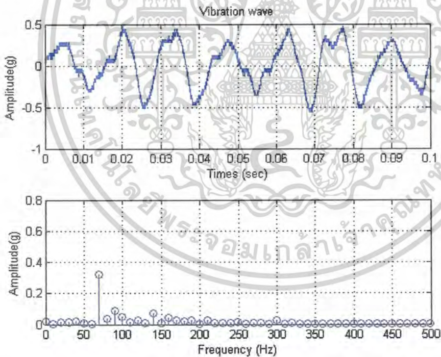
รูปที่ 8.34 แสดงสเปกตรัมของการสั่นสะเทือนเมื่อได้รับฮาร์มอนิกลำดับที่ 5 ที่มีค่าความเพี้ยนตกคาไฟฟ้า 15 เปอร์เซ็นต์ และมีการเรียงลำดับเฟสในทิศทางลบ
