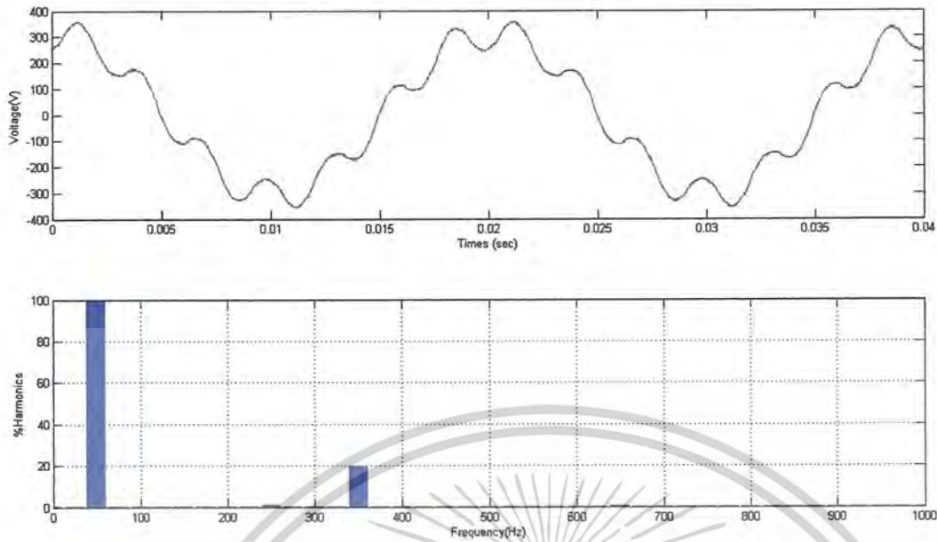
ภาพที่ 8.9 ผลรวมของความถี่มูลฐานกับความถี่ฮาร์โมนิกส์ที่มีลำดับเฟสบวก และสเปกตรัมของผลรวมความถี่มูลฐานกับความถี่ฮาร์โมนิกส์อันดับที่ 7 ที่เปอร์เซ็นต์ความเพี้ยนศักดาไฟฟ้า 20 เปอร์เซ็นต์
