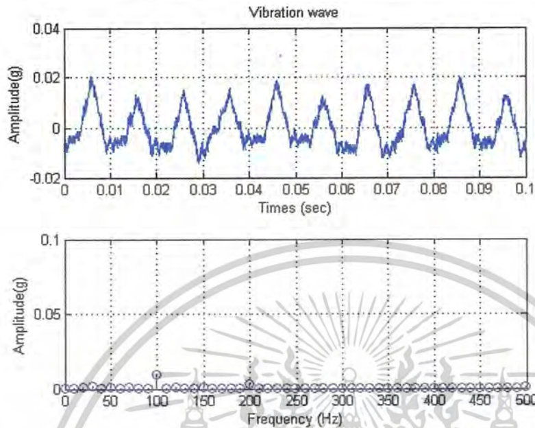
รูปที่ 8.20 แสดงสเปกตรัมของการสั่นสะเทือนที่เกิดจากแรงดันไฟฟ้าสามเฟสไม่สมดุล
