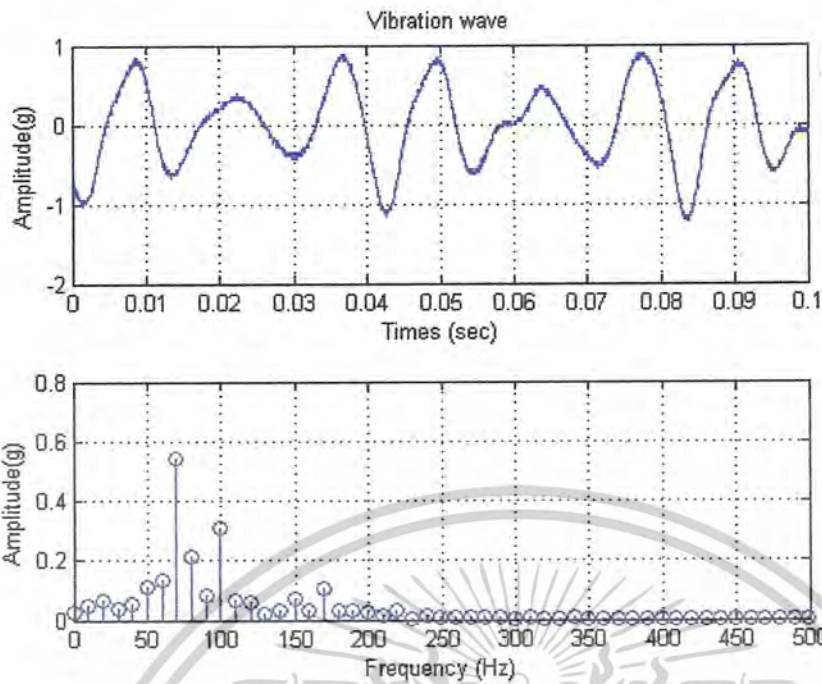
ภาพที่ 8.53 แสดงสเปกตรัมของการสั่นสะเทือนที่เกิดจากแรงดันไฟฟ้าเฟส a 218V เฟส b 213V และเฟส c 206V (3U3%)
