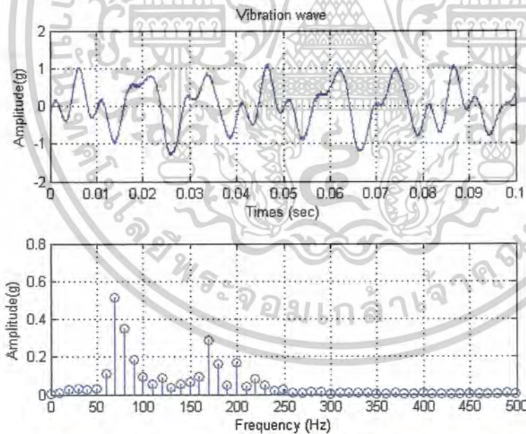
ภาพที่ 8.72 แสดงสเปกตรัมของการสั่นสะเทือนเมื่อได้รับฮาร์มอนิกส์ลำดับที่ 3 ที่มีค่าความเพี้ยนสัปดาห์ไฟฟ้า 15 เปอร์เซ็นต์ และมีการเรียงลำดับเฟสในทิศทางลบ
