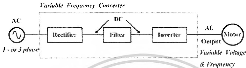
ภาพที่ 2.16 โครงสร้างพื้นฐานของระบบเครื่องปรับความเร็วรอบ
