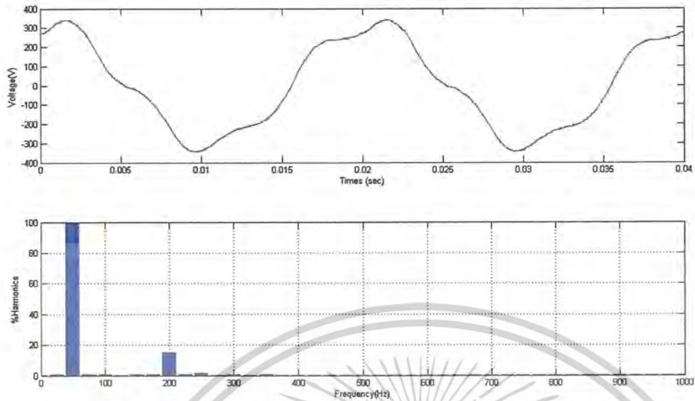
ภาพที่ 8.5 ผลรวมของความถี่มูลฐานกับความถี่ฮาร์โมนิกส์ที่มีลำดับเฟสบวก และสเปกตรัมของผลรวมความถี่มูลฐานกับความถี่ฮาร์โมนิกส์อันดับที่ 4 ที่เปอร์เซ็นต์ความเพี้ยนศักดาไฟฟ้า 15 เปอร์เซ็นต์
