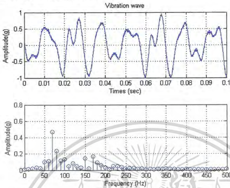
ภาพที่ 8.71 แสดงสเปกตรัมของการสั่นสะเทือนเมื่อได้รับฮาร์มอนิกส์ลำดับที่ 3 ที่มีค่าความเพี้ยนสัปดาห์ไฟฟ้า 15 เปอร์เซ็นต์ และมีการเรียงลำดับเฟสในทิศทางบวก
