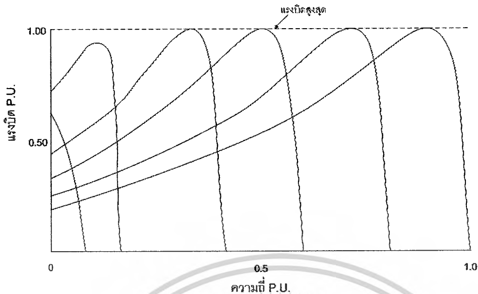
ภาพที่ 2.10 กราฟแสดงความสัมพันธ์แรงบิด – ความเร็วรอบ ที่อัตราส่วน \frac{V_s}{\omega_s} คงที่
