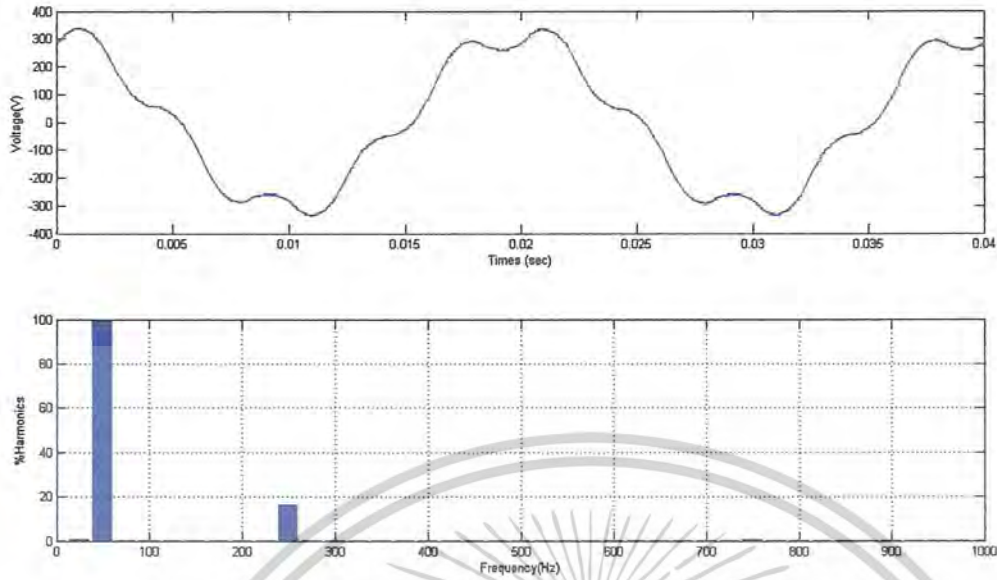
ภาพที่ 8.7 ผลรวมของความถี่มูลฐานกับความถี่ฮาร์โมนิกที่มีลำดับเฟสบวก และสเปกตรัมของผลรวมความถี่มูลฐานกับความถี่ฮาร์โมนิกอันดับที่ 5 ที่เปอร์เซ็นต์ความเพี้ยนศักดาไฟฟ้า 15 เปอร์เซ็นต์
