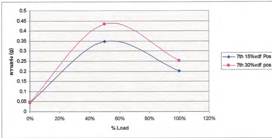
รูปที่ 8.94 การเปรียบเทียบระหว่างค่าการสันสะท้อนกับเปอร์เซ็นต์โหลดของฮาร์มอนิกอันดับที่ 7 ที่มีค่าความเพี้ยนศักดาไฟฟ้า 15 และ 30 เปอร์เซ็นต์และมีการเรียงลำดับเฟสแบบบวก
