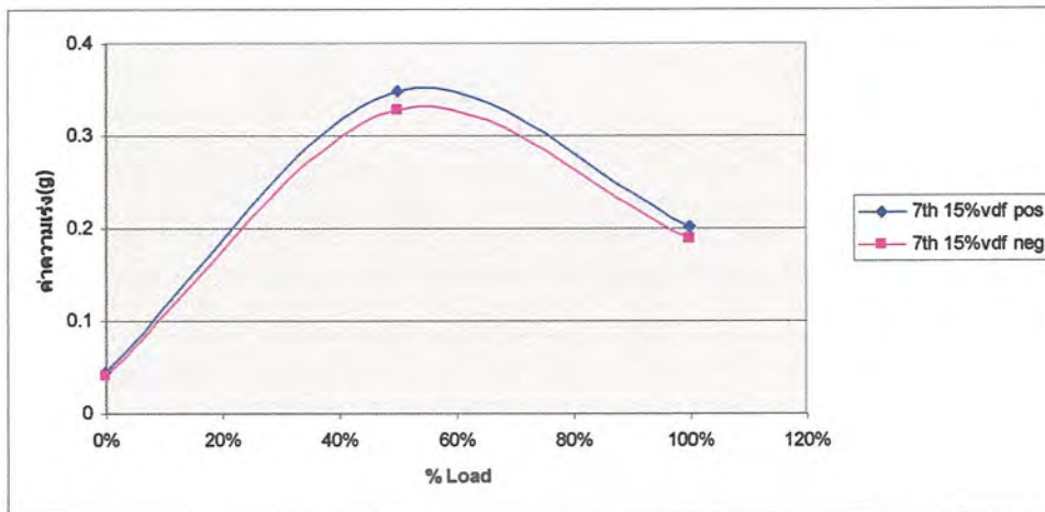
รูปที่ 8.91 การเปรียบเทียบระหว่างค่าการสั่นสะเทือนกับเปอร์เซ็นต์โหลดที่ฮาร์มอนิกส์อันดับที่ 7 ที่มีการเรียงลำดับเฟสแบบบวกและแบบลบ
