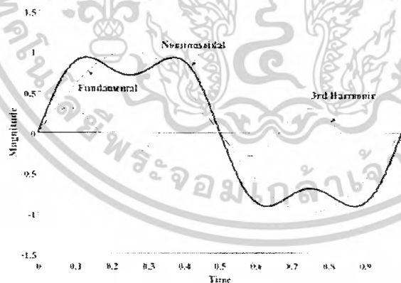
ภาพที่ 4.10 ผลของฮาร์มอนิกส์ที่มีเฟสตรงกับความถี่มูลฐาน
