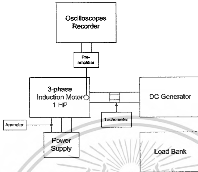
ภาพที่ 7.2 แสดงการต่ออุปกรณ์ที่ใช้ในการทดลองการสั้นสะท้อน
