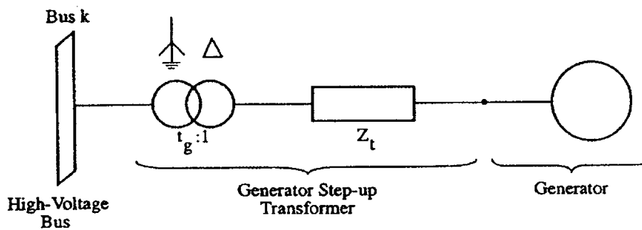
รูปที่ 2.10 แบบจำลองเครื่องกำเนิดไฟฟ้า
