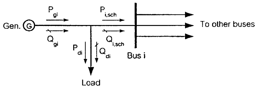
รูปที่ 2.3 แผนภาพเส้นเดียวแสดงการไหลของกำลังไฟฟ้าที่บัส i
