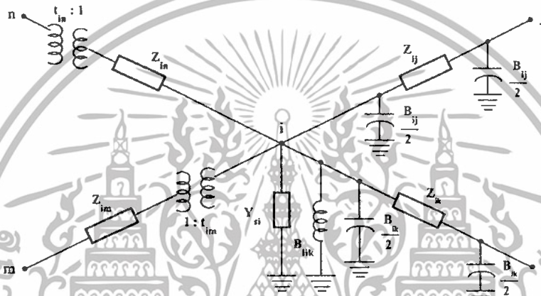
รูปที่ 2.2 วงจรสมมูลซีเควนซ์บวคของโครงข่ายระบบไฟฟ้า Node i
