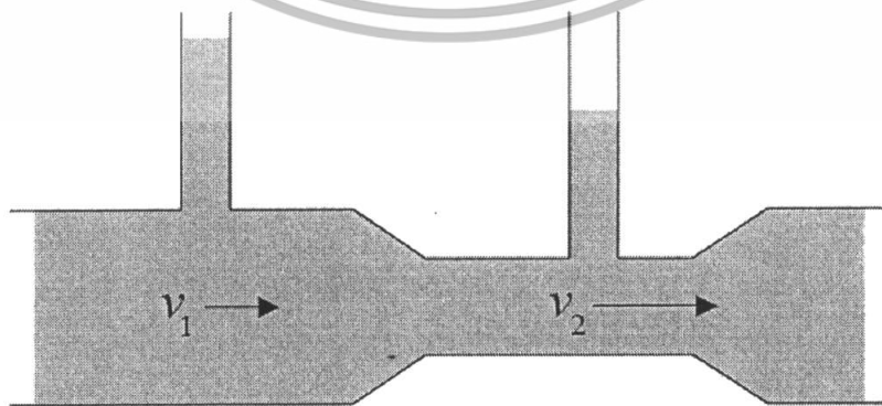
รูปที่ 2.7 มาตรการเวนจูรี
