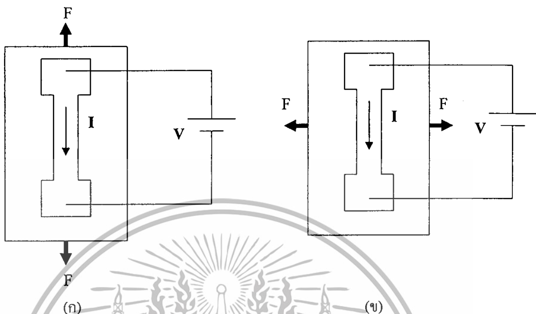
รูปที่ 2.11 ทิศทางของแรงที่มากกระทำกับวัสดุที่ประกอบด้วย(ก) แรงดึงตามยาว (ข) แรงดึงตามขวาง
