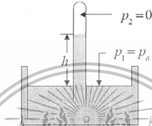
รูปที่ 2.4 บารอมิเตอร์แบบปรอท
