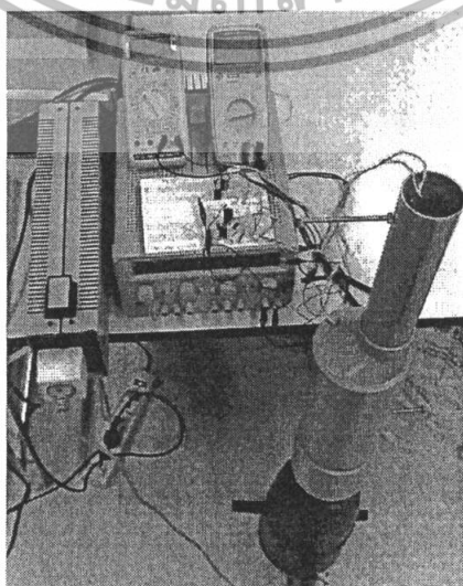
เอกสารนี้เป็นเอกสารที่สงวนไว้สำหรับการใช้งานเพื่อการศึกษาเท่านั้น ไม่อนุญาตให้นำไปใช้ประโยชน์ด้านการค้า รูปที่ 3.7 ชุดทดลองตัวตรวจวัด แบบมาตรฐานจอร์
