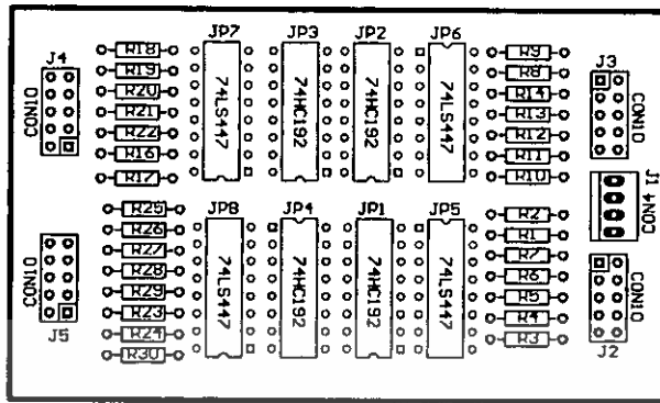
รูปที่ ข.6 ตำแหน่งการวางอุปกรณ์แผ่นวงจร
