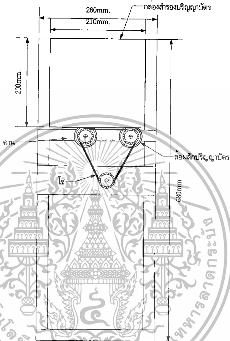
รูปที่ 3.11 ด้านข้างโครงสร้างและส่วนประกอบชุดสำรองจ่ายปริญาบัตร
