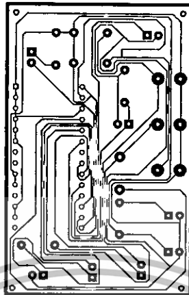
รูปที่ ๑.8 แผงวงจรพิมพ์วงจรจรรยาบทึกเสียงดิจิทัล
