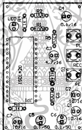
รูปที่ ๑.9 ตำแหน่งการวางอุปกรณ์แผงจรรยาบทึกเสียงดิจิทัล
