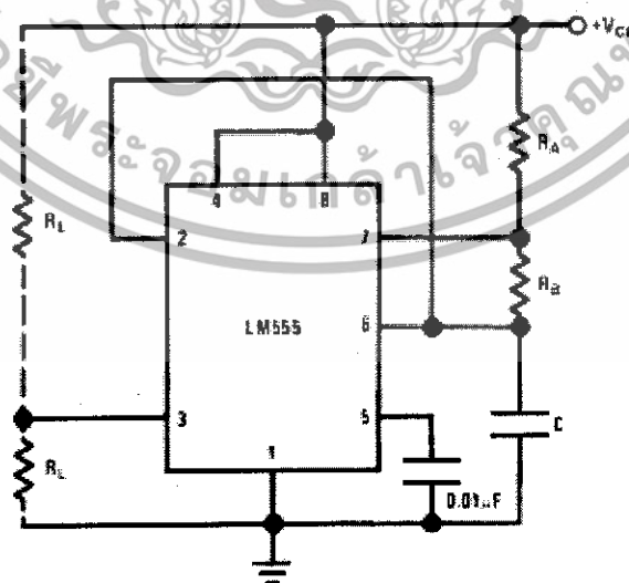
รูปที่ 3.2 แสดงวงจรที่ใช้คำนวณหาค่าความถี่ของ IC555
