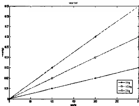
กราฟที่ 3 แสดงความสัมพันธ์ระหว่างการสึกหรอกับความเร็วรอบ (หัวกดแบบ Polypropylene และจานหมุนแบบ Polyethylene)
