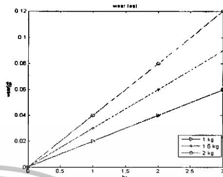
กราฟที่ 5 แสดงความสัมพันธ์ระหว่างรัศมีของการกด 35,45,55 mm น้ำหนักกด 1,1.5,2 Kg ใช้ความเร็วรอบในการทดสอบ 300 รอบ/นาที (หัวกดเป็น Polypropylene และจานหมุนเป็น Polyethylene)
