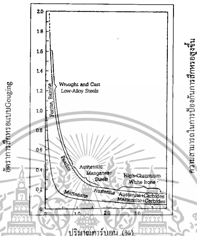
รูปที่ 2.11 แสดงความสัมพันธ์ระหว่างอัตราส่วนของการสึกหรอแบบ Gouging กับปริมาณคาร์บอนในเหล็กอัลลอย และกับความแข็งของผิวที่ผ่านการทำให้แข็งด้วยความเครียด
