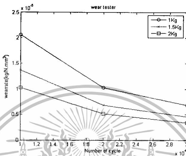
กราฟที่ 7 เปรียบเทียบอัตราการสึกหรอหัวกดแบบ Polypropylene กับ งานหมุน Polyethylene
