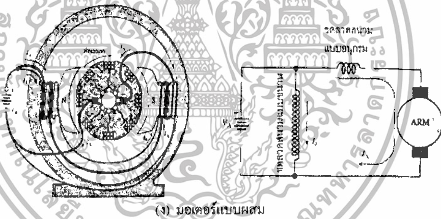
รูปที่ 2.21 แผนภูมิการพันมอเตอร์และคุณลักษณะอัตราเร็ว - ทอร์กของมอเตอร์กระแสตรง
