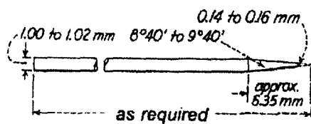
รูปที่ 3.3 แสดงขนาดของเข็มหาค่าการทดลอง
