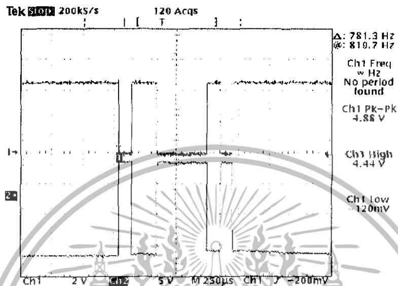
รูปที่ 4.4 แสดงการเปรียบเทียบการแปลงระดับสัญญาณ ของวงจรเชื่อมต่อกับพอร์ตอนุกรมของคอมพิวเตอร์
