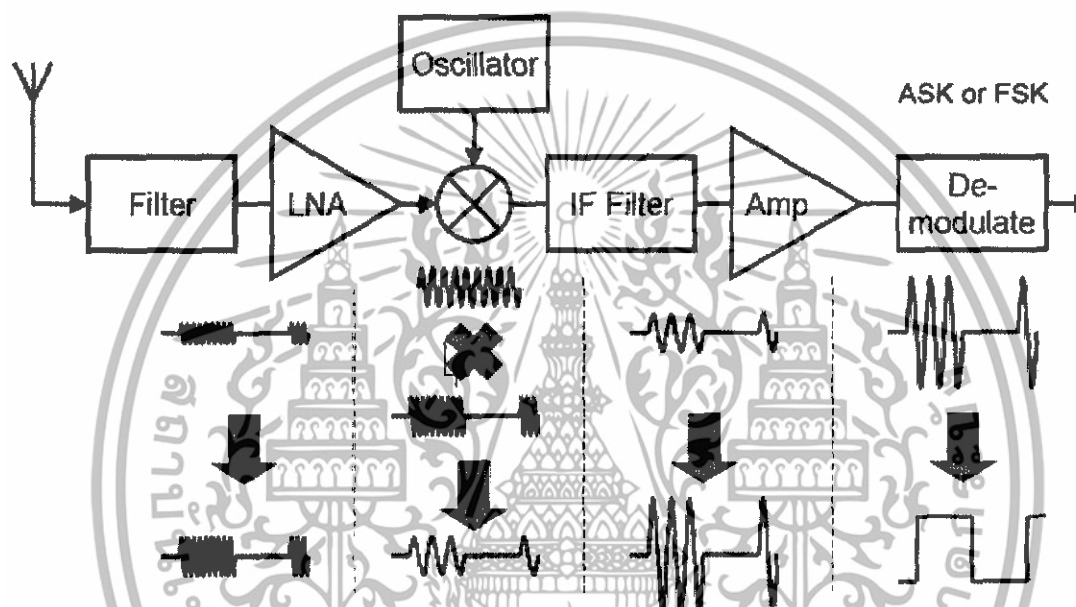
รูปที่ 2.15 บล็อกไดอะแกรมของ ไอซี rRXD0420
