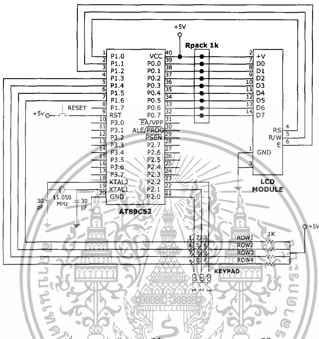
รูปที่ 3.5 วงจรรับข้อมูลจากคีย์แพดและแสดงผลทางจอแอลซีดี
