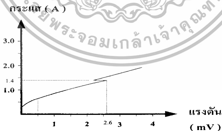
รูปที่ 3.15 กราฟความสัมพันธ์ระหว่างกระแสกับแรงดัน ไฟฟ้าที่สนามแม่เหล็กค่าต่างๆ ที่อุณหภูมิกำลัง 950 องศาเซลเซียส
