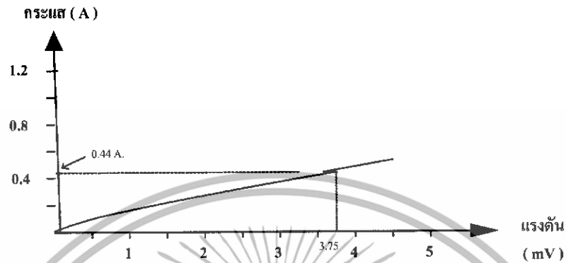
รูปที่ 3.18 กราฟความสัมพันธ์ระหว่างกระแสกับแรงดันไฟฟ้าที่สนามแม่เหล็กค่าต่างๆ ที่อุณหภูมิกาวา 970 องศาเซลเซียส
