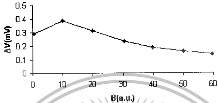
รูปที่ 3.16 กราฟแสดงความสัมพันธ์ระหว่างสนามแม่เหล็กกับขนาดการเปลี่ยนแปลงแรงดันขณะที่เกิดความต้านทานเชิงลบ ที่อุณหภูมิการเผา 950 องศาเซลเซียส
