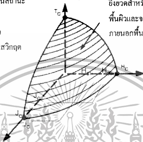
รูปที่ 1.3 ความสัมพันธ์ของสถานะการนำไฟฟ้ายิ่งยวดที่ขึ้นอยู่กับอุณหภูมิ, สนามแม่เหล็ก และความหนาแน่นกระแส
