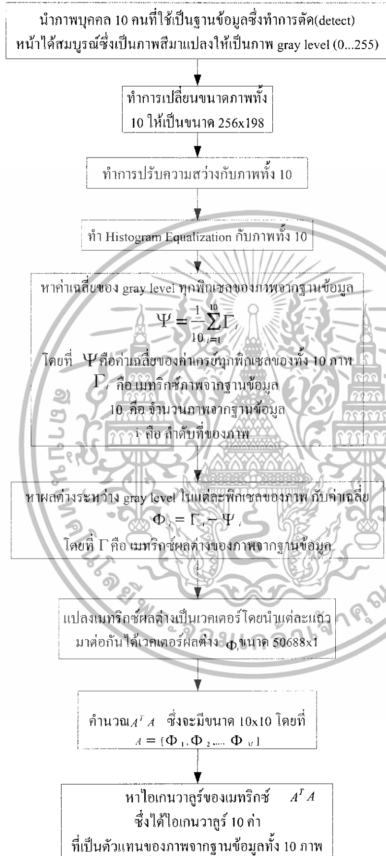
รูปที่ 3.6 แสดงการหาไอเกนวาเลจของภาพ
