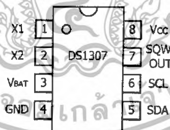
รูปที่ 3.7 การจัดขาของไอซี DS 1307 ไอซีสร้างฐานเวลาจริง (RTC)
