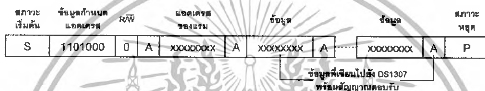
รูปที่ 3.10 รูปแบบของข้อมูลสำหรับติดต่อกับ DS 1307 ในโหมดการเขียนข้อมูล
