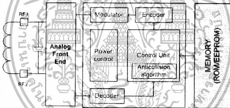
รูปที่ 5.3 แสดงบล็อกโคะแกรมของ Passive Tag
