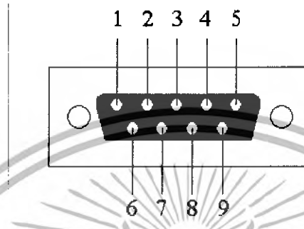
รูปที่ 4.1 คอนเน็คเตอร์อนุกรม 9 ขาหรือแบบ DB-9
