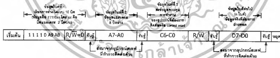
รูปที่ 3.6 รูปแบบของข้อมูลอนุกรมที่ใช้ติดต่อกับอุปกรณ์บัส I 2 C เมื่อใช้การอ้างถึงแบบ 10 บิต
