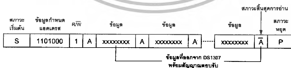
รูปที่ 3.11 รูปแบบของข้อมูลสำหรับติดต่อกับ DS 1307 ในโหมดการอ่านข้อมูล
