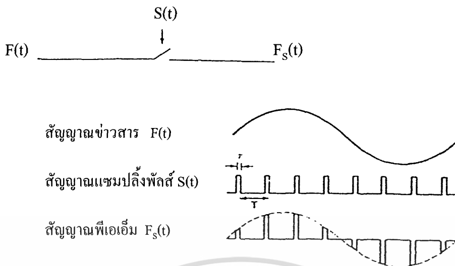
รูปที่ 2.7 ระบบการซักรหัสสัญญาณและสัญญาณ
