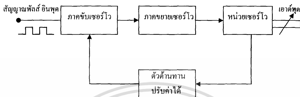
รูปที่ 2.17 การทำงานของเซอร์โว
