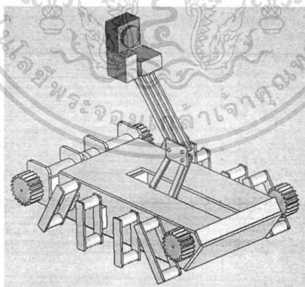
รูปที่ 3.24 การประกอบเฟืองขับเคลื่อนและเฟืองช่วยขับเคลื่อนกับ โครงสร้างหลัก
