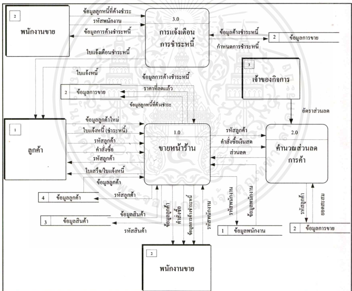
ภาพที่ 5 ผังแสดงการไหลเวียนของข้อมูลระดับที่ 0 (Data Flow Diagram Level 0)
