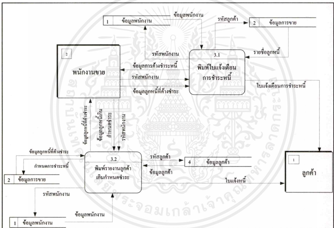
ภาพที่ 7 ผังแสดงการไหลเวียนของข้อมูลระดับที่ 1(3.0 กระบวนการแจ้งเตือนการชำระหนี้)
