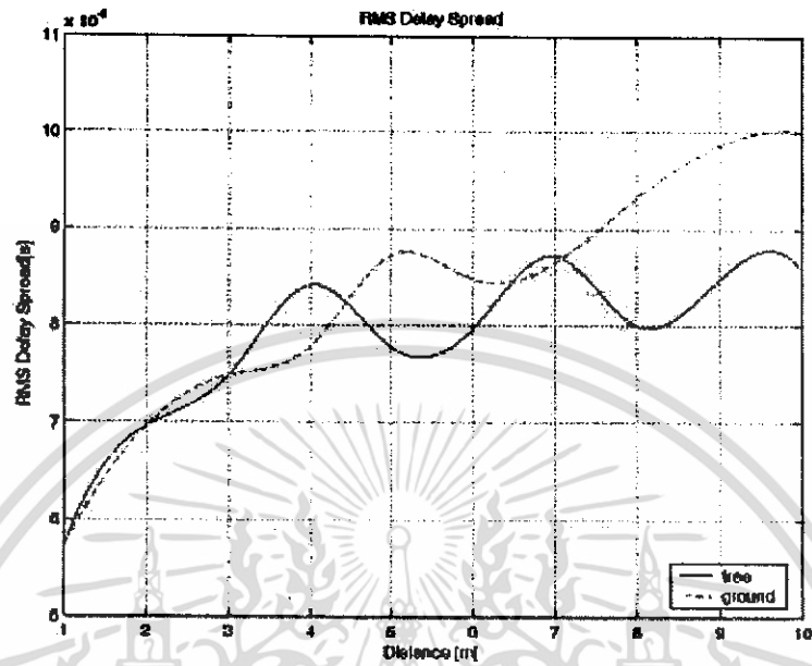
รูปที่ 4.15a การเปรียบเทียบ RMS Delay Spread ของ Free Space กับ Ground Reflection
