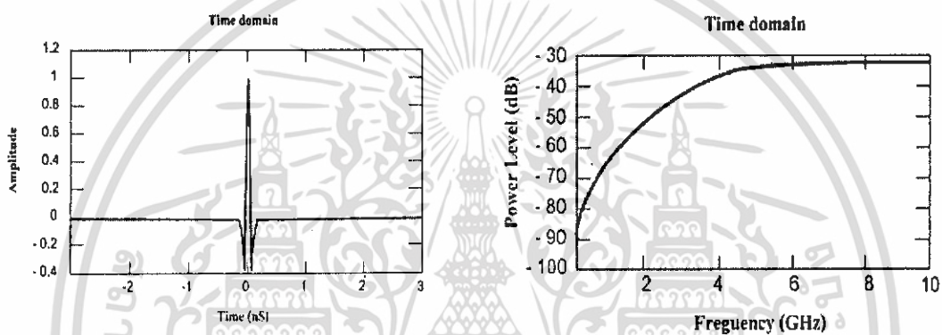
รูปที่ 2.8 รูปสัญญาณพัลส์แบบเกาส์เขียนทับเล็ททั้งใน โดเมนเวลาและ โดเมนความถี่
