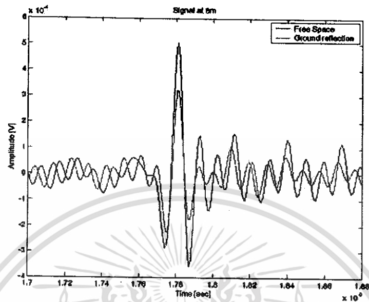
รูปที่ 4.18c การเปรียบเทียบสัญญาณ Free Space กับ Ground Reflection ทางด้านรับที่ ระยะทาง 8 เมตร
