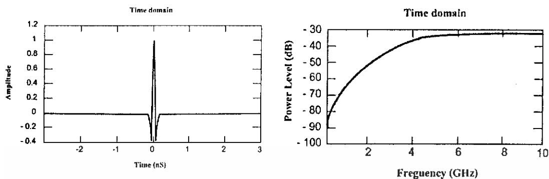
รูปที่ 2.2 ลักษณะของสัญญาณพัลส์ใน โดเมนเวลาและแถบกำลังงานของสัญญาณในเมนความถี่
