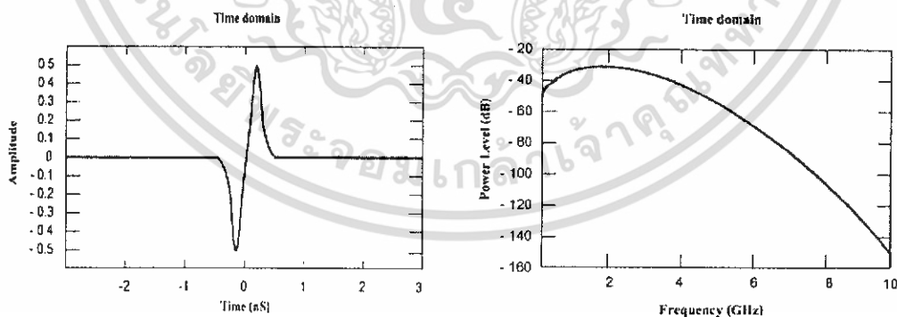
รูปที่ 2.7 รูปสัญญาณพัลส์แบบเกาส์เซียน โมนอไซเคิลทั้งใน โดเมนเวลาและ โดเมนความถี่
