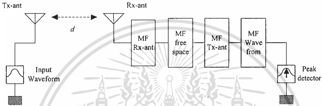
รูปที่ 2.19 บล็อกไดอแกรมของระบบการส่งสัญญาณที่ได้มีการเพิ่มเติมจากสูตรของฟรีต (Friis' transmission) เพื่อนำมาใช้กับระบบอุลตราไวด์แบนด์
