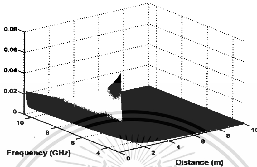
รูปที่ 4.3 ฟังก์ชันถ่ายโอนของอัตราการขยายเชิงวิถี (Transfer function of free space)
