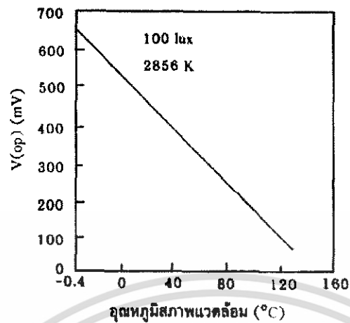
รูปที่ 11 ความสัมพันธ์ระหว่างแรงดันวงจรเปิดในโฟโตไดโอดชนิดซิลิคอนและอุณหภูมิสภาพแวดล้อม
