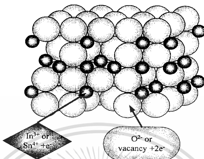
รูปที่ 2.2 แสดง โครงสร้างอะตอมของอินเดียมออกไซด์ (In 2 O 3 ) ถูกเจือด้วยดีบุก (Sn)
