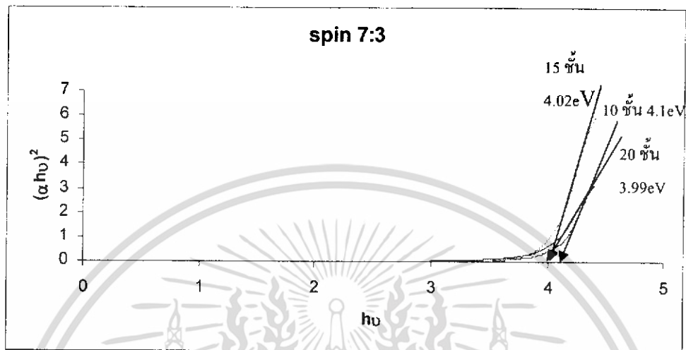
รูปที่ 4.15 กราฟแสดงความสัมพันธ์ระหว่างค่า (\alpha h\nu)^2 กับค่าพลังงานโฟตอนซึ่งก็คือค่าแถบพลังงานต้องห้ามของวิธีหมุนเคลือบที่อัตราส่วน In:Sn เป็น 7:3
