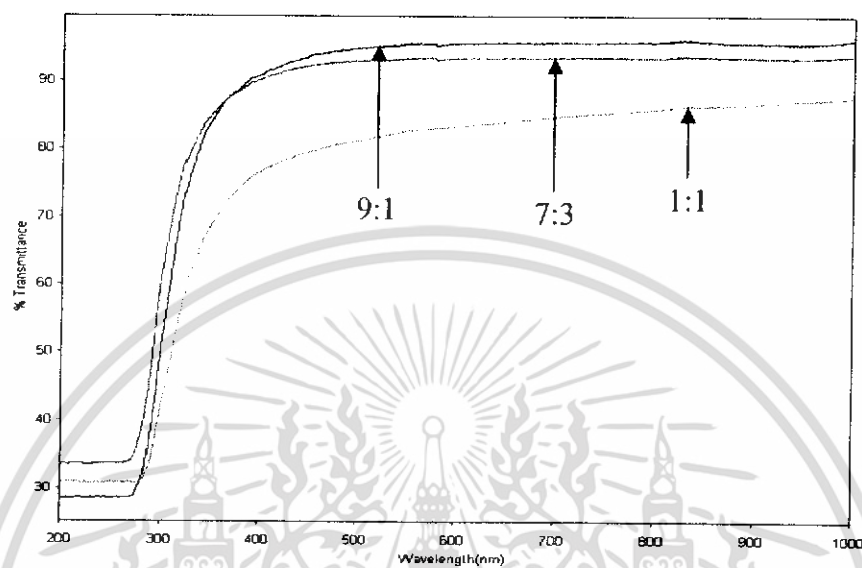
รูปที่ 4.6 กราฟแสดงความสัมพันธ์ระหว่างค่าการส่องผ่านกับความยาวคลื่นของฟิล์มบาง ITO ที่ปลูกโดยวิธีหมุนเคลือบความหนา 10 ชั้น
