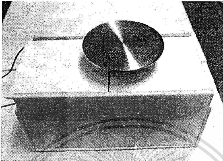
รูปที่ 3.5 เครื่องหมุนเคลือบ
