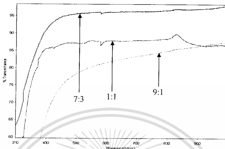
รูปที่ 4.5 กราฟแสดงความสัมพันธ์ระหว่างค่าการส่งผ่านกับความยาวคลื่นของฟิล์มบาง ITO ที่ปลูกโดยวิธีจุ่มเคลือบความหนา 30 ชั้น
