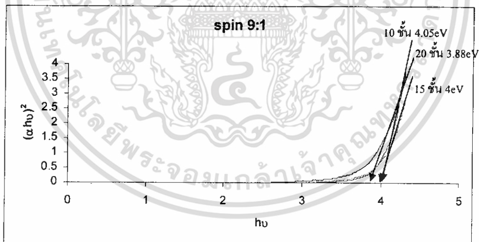
รูปที่ 4.16 กราฟแสดงความสัมพันธ์ระหว่างค่า (\alpha h\nu)^2 กับค่าพลังงานโฟตอนซึ่งก็คือค่าแถบพลังงานต้องห้ามของวิธีหมุนเคลือบที่อัตราส่วน In:Sn เป็น 9:1
