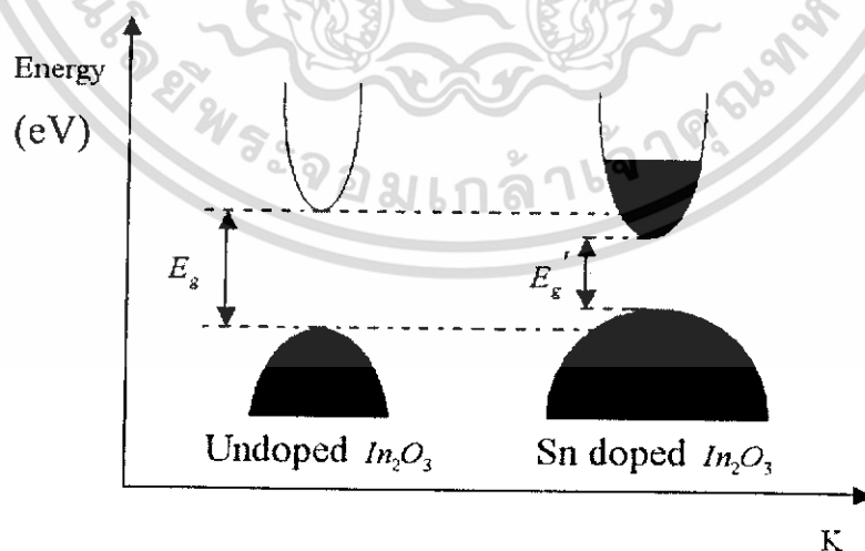
รูปที่ 2.3 แสดง โครงสร้างของแถบพลังงานที่มีลักษณะเป็นพาราโบลาของ In 2 O 3
