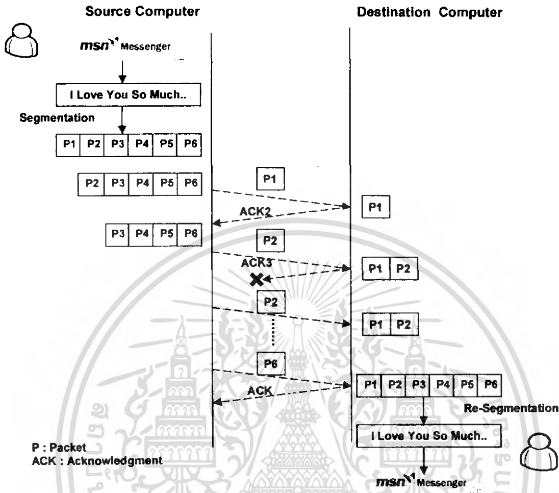
รูปที่ 2.32 การติดต่อสื่อสารผ่านโปรโตคอลที่ซีพีอาร์พีปลายทางยังไม่ได้รับการตอบรับ [9]
