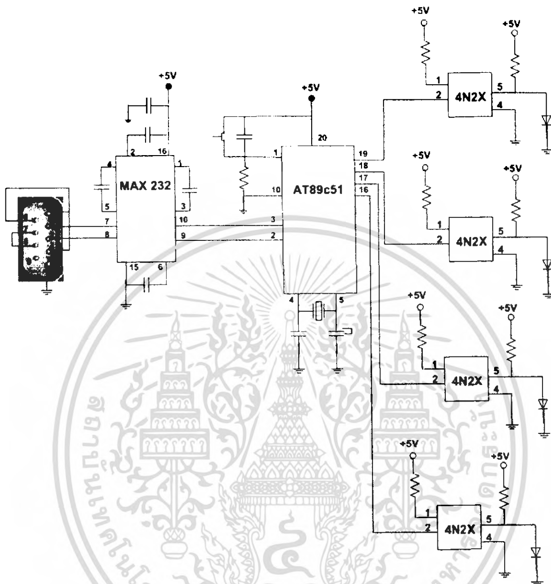
รูปที่ 3.2 วงจรส่วนควบคุมรถคลอง
