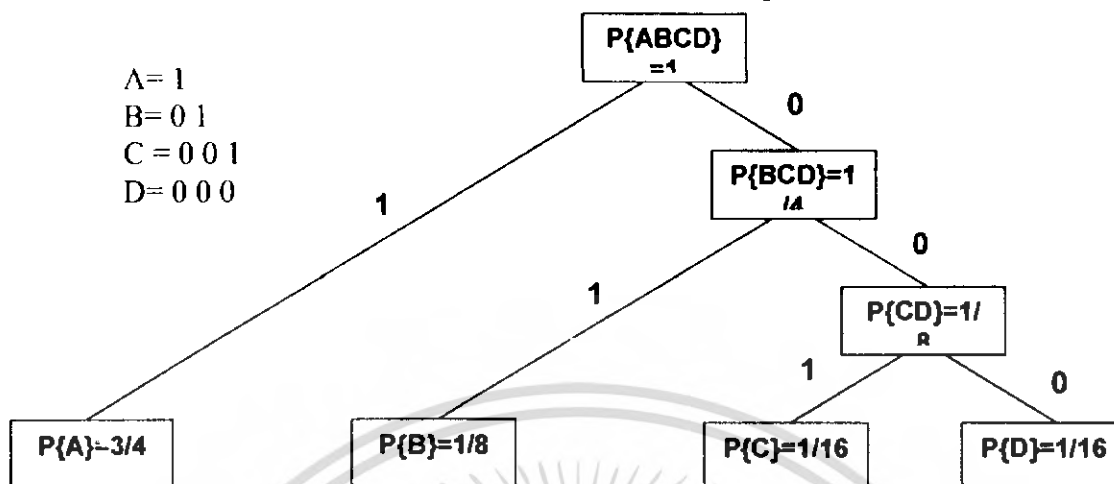
รูปที่ 2.17 ขั้นตอนการเข้ารหัสฮัฟแมน (Huffman Coding)
