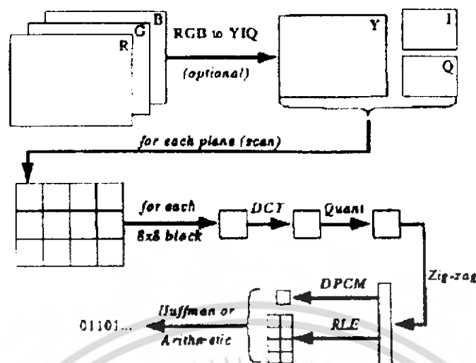
รูปที่ 2.23 รายละเอียดขั้นตอนการบีบอัดข้อมูลภาพนิ่งเจเพ็ก [11]
