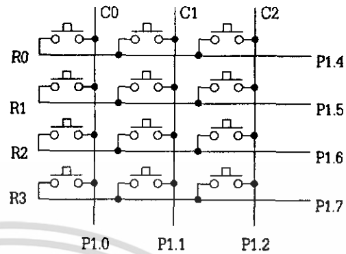
ข. การต่อสวิตช์ใช้งานแบบเมทริกซ์
