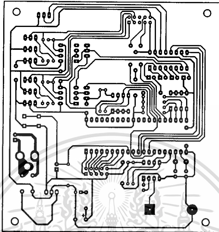
รูปที่ ๒.2 แผงวงจรพิมพ์วงจรควบคุมหลัก
