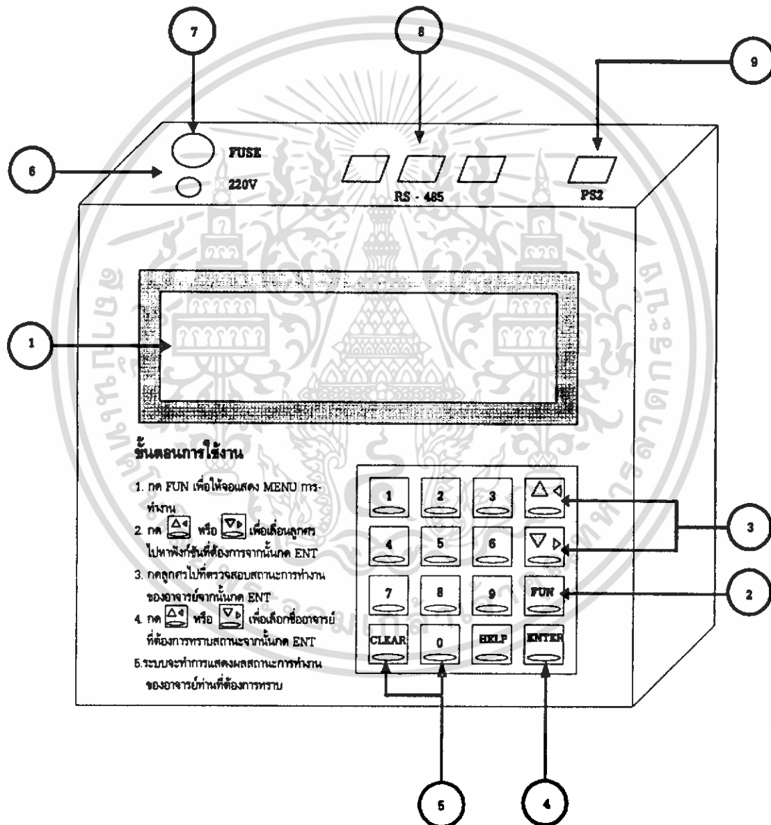
รูปที่ ๑.1 ส่วนประกอบและปุ่มควบคุมของแผงแสดงผลสถานะการทำงานของอาจารย์
