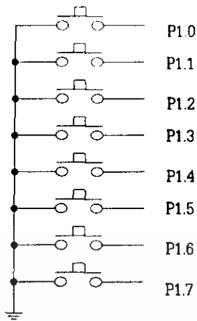
ก. การต่อสวิตช์ใช้งานแบบเดี่ยว
