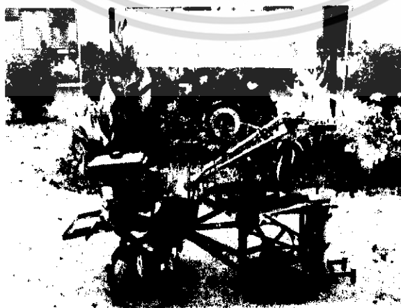
เอกสารรูปที่ 3.32 เครื่องยักกล้าที่สร้างเสร็จสมบูรณ์และนำมาติดตั้งเข้ากับรถไถเดินตามขนาด 5 แรงม้า ไม่ว่ากรณีใดๆทั้งสิ้น อีกทั้งห้ามมิให้ดัดแปลงเนื้อหา และต้องอ้างอิงถึงเจ้าของเอกสารทุกครั้งที่มีการนำไปใช้
