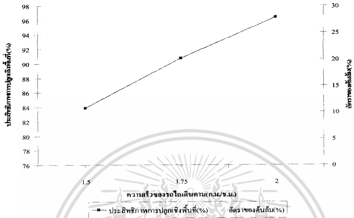
รูปที่ 4.22 กราฟแสดงความสัมพันธ์ระหว่าง ความเร็วของรถไถเดินตาม กับ ประสิทธิภาพการปลุกเชิงพื้นที่ และอัตราของต้นล้ม
