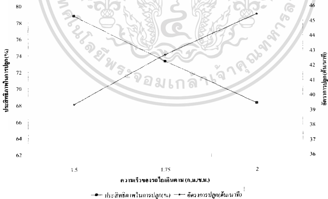
รูปที่ 4.15 กราฟแสดงความสัมพันธ์ระหว่าง ความเร็วของรถไถเดินตาม กับ ประสิทธิภาพในการปลูก และอัตราการปลูก
