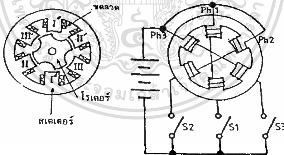
รูปที่ 2.9 แสดงภาพหน้าตัดและการพันขดลวดของสเต็ปมอเตอร์ 3 เฟส
