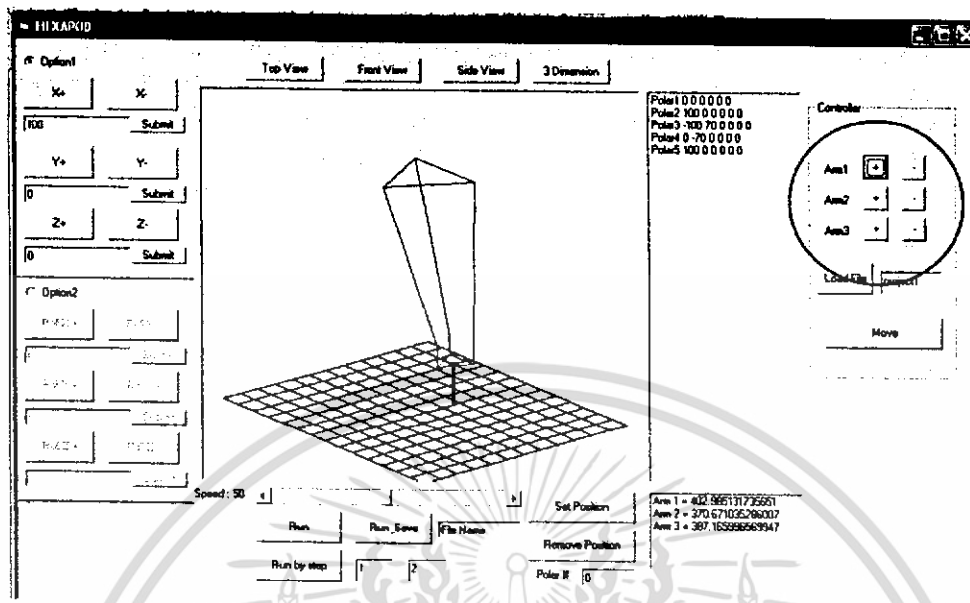
รูปที่ 4.21 แสดงการใช้คำสั่ง Arm1
