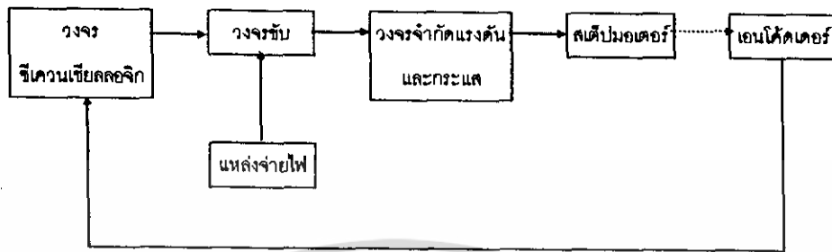
รูปที่ 2.20 แสดงบล็อกไดอะแกรมของระบบควบคุมสเต็ปมอเตอร์
