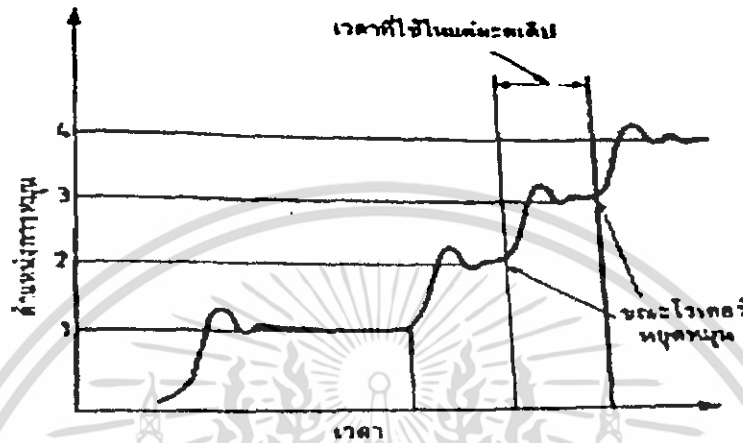
รูปที่ 2.15 กราฟแสดงการหมุนในโหมดการทำงานแบบหมุนเป็นสเต็ป
