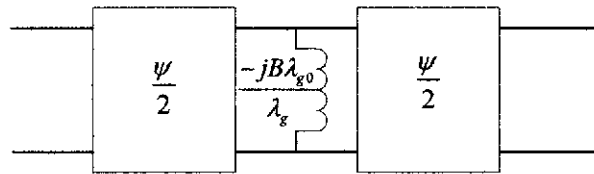
รูปที่ 2.13 วงจรสมมูลของฉากรัดที่วางในท่อนำคลื่น
