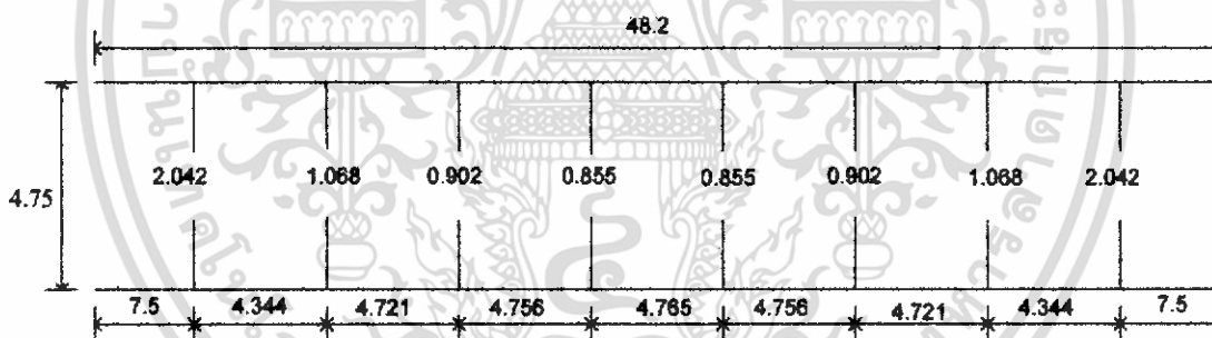
รูปที่ 4.1 ขนาดระยะห่างต่างๆ ภายในท่อทองเหลืองที่มีความถี่ตัดที่ 4.35-4.45 GHz หน่วยเป็น cm.
