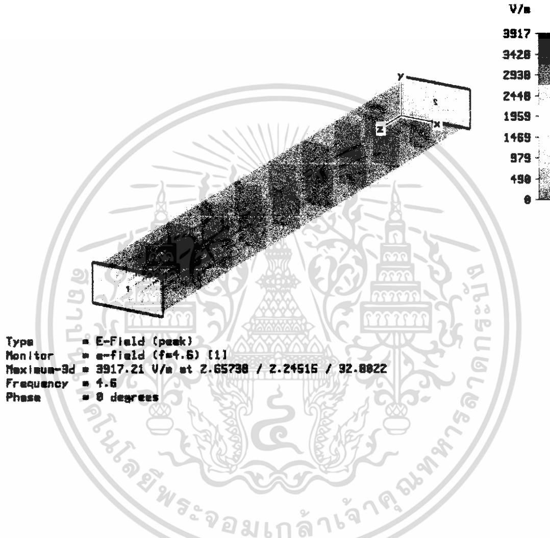
รูปที่ 4.25 ลักษณะของสนามไฟฟ้าที่ถูกกลดทอนจึงไม่มีการส่งผ่านที่ความถี่ 4.6 GHz
