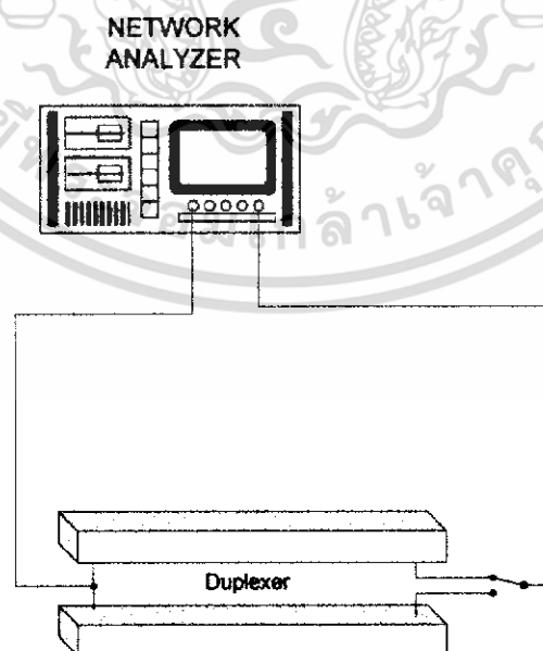
รูปที่ 5.11 การต่ออุปกรณ์การทดสอบ Insertion Loss, Return Loss, Impedance ของดูเพล็กซ์เซอร์ เอกสารนี้เป็นเอกสารที่สงวนไว้สำหรับการใช้งานเพื่อการศึกษาเท่านั้น ไม่อนุญาตให้นำไปใช้ประโยชน์ด้านการค้า ไม่ว่ากรณีใดๆทั้งสิ้น อีกทั้งห้ามมิให้ดัดแปลงเนื้อหา และต้องอ้างอิงถึงเจ้าของเอกสารทุกครั้งที่มีการนำไปใช้
