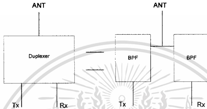
รูปที่ 3.1 แสดงการนำพาสแบนด์สองตัวมาเชื่อมต่อกันเป็นคูเพล็กซ์เซอร์
