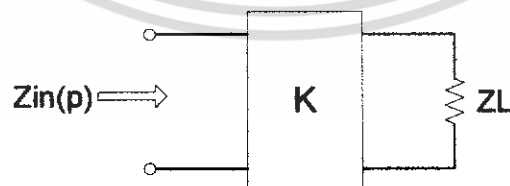
รูปที่ 2.11 รูปแบบทวิพอร์ตอิมพีแดนซ์อินเวอร์เตอร์
