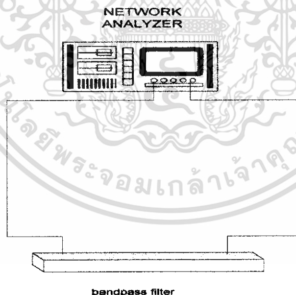
รูปที่ 5.1 การต่ออุปกรณ์การทดสอบ Insertion Loss, Return Loss, Impedance ของฟิลเตอร์
