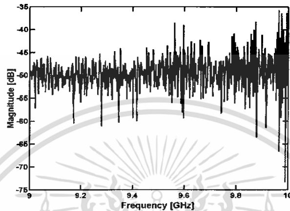
รูปที่ 4.46 ค่าแมคนิจูดของช่องสัญญาณความถี่ที่ย่านความถี่ 9 – 10 GHz ที่ระยะห่างระหว่างสายอากาศส่งและสายอากาศรับ 1 เมตร
