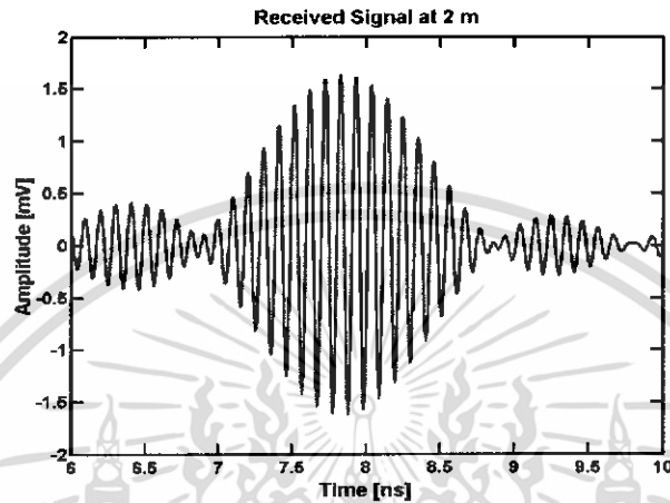
รูปที่ 4.90 สัญญาณทางด้านการรับในรูปโดเมนเวลา
