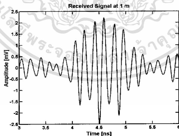
รูปที่ 4.127 สัญญาณทางด้านรับในรูปโดเมนเวลา
