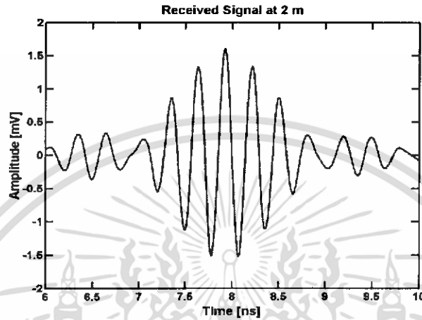
รูปที่ 4.60 สัญญาณทางด้านการรับในรูปโดเมนเวลา
