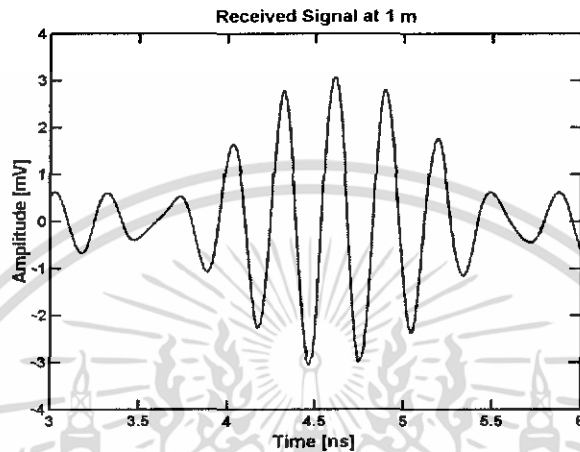
รูปที่ 4.20 สัญญาณทางด้่านรับในรูปโดเมนเวลา
