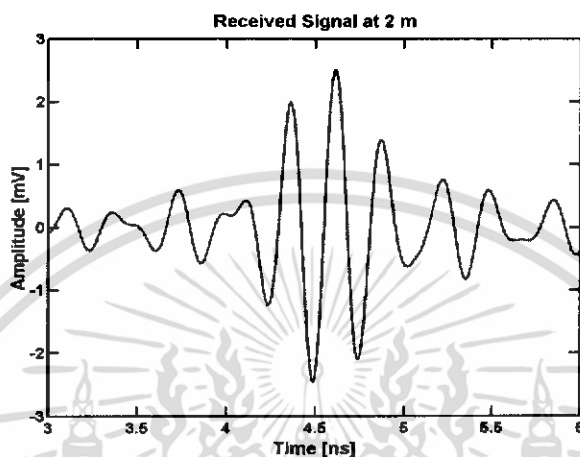
รูปที่ 4.102 สัญญาณทางด้านการรับในรูปโดเมนเวลา
