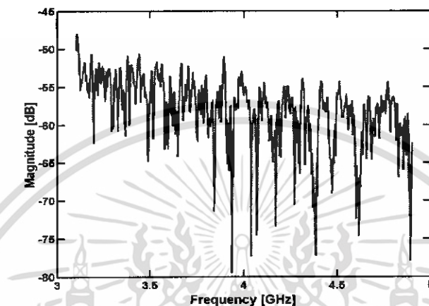
รูปที่ 4.118 ค่าแมกนิจูดของช่องสัญญาณความถี่ที่ย่านความถี่ 3.1-4.9 GHz ที่ระยะห่างระหว่างสายอากาศส่งและสายอากาศรับ 2 เมตร
