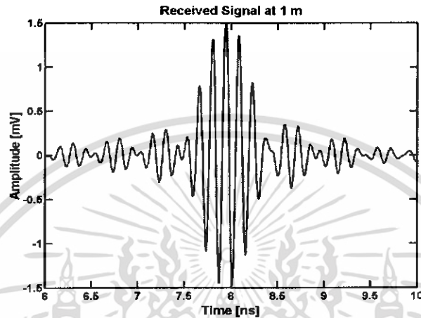
รูปที่ 4.132 สัญญาณทางด้านการรับในรูปโดเมนเวลา
