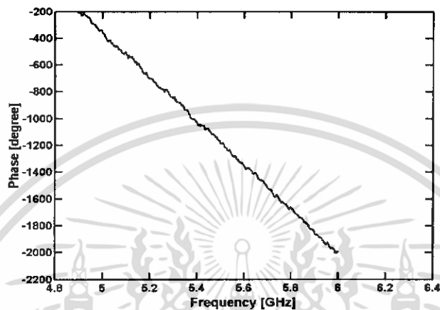
รูปที่ 4.104 ค่าเฟสของช่องสัญญาณความถี่ที่ย่านความถี่ 4.9 - 6 GHz ที่ระยะห่างระหว่างสายอากาศส่งและสายอากาศรับ 1 เมตร
