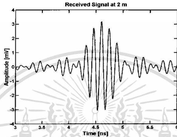
รูปที่ 4.112 สัญญาณทางค่านรับในรูปโดเมนเวลา
