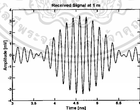
รูปที่ 4.35 สัญญาณทางต้านรับในรูปโดเมนเวลา
