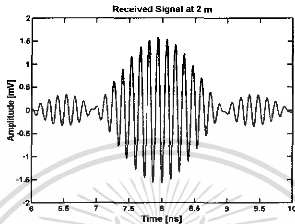
รูปที่ 4.80 สัญญาณทางด้านรับในรูปโดเมนเวลา
