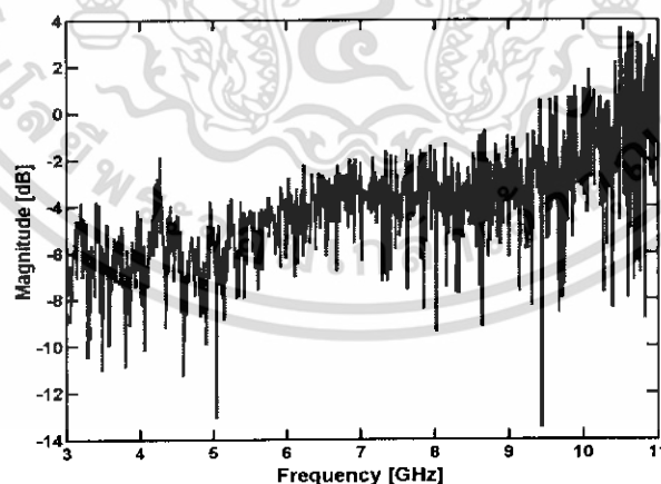
รูปที่ 4.13 ค่าแมคนิจูดของสายอากาศที่ย่านความถี่ 3 – 11 GHz ที่ระยะห่างระหว่างสายอากาศส่งและสายอากาศรับ 2 เมตร
