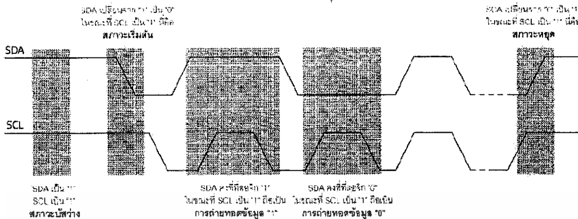
รูปที่ 3.13 ไคอะแกรมเวลาแสดงสถานะต่างๆบนระบบบัส I 2 C
