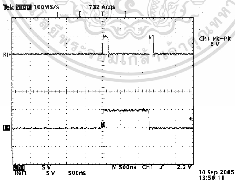
รูปที่ 4.18 สัญญาณที่ได้จากวงจร D- Flip Flop 1 หรือวงจรตรวจับเวลา
