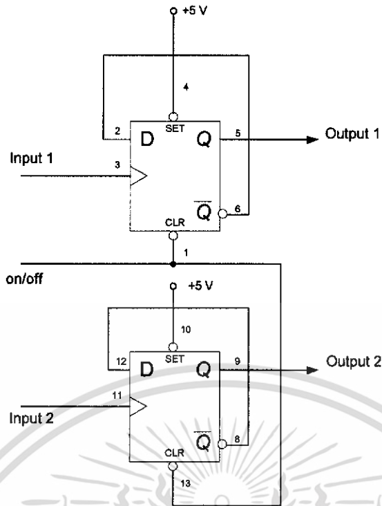
รูปที่ 4.17 วงจรตรวจับเวลาและวงจรตรวจสอบสถานะ
