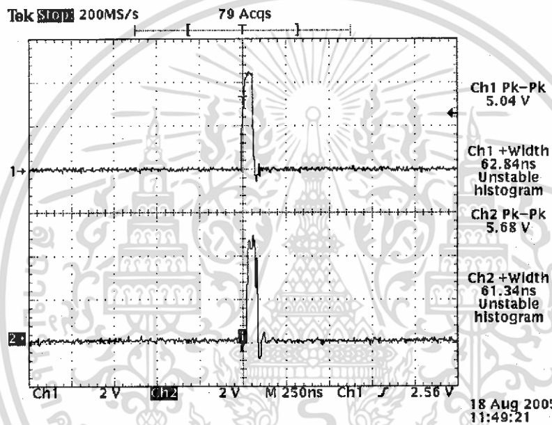
รูปที่ 4.8 ตัวอย่างสัญญาณจากวงจรเลือกสัญญาณเมื่อ A=0 , B=0
