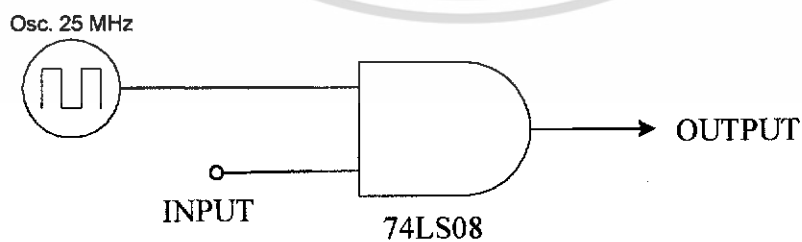
รูปที่ 4.20 วงจรคูณสัญญาณ และวงจรผลิตสัญญาณความถี่ 25 MHz
