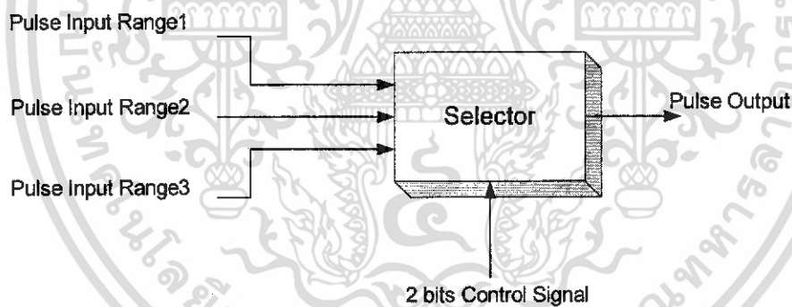
รูปที่ 3.2 บล็อกโคจรของวงจรเลือกสัญญาณ
