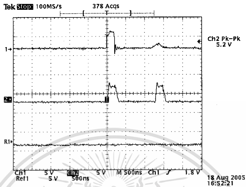
รูปที่ 4.12 สัญญาณที่ได้จากวงจรตรวจจับพัลส์ เปรียบเทียบกับสัญญาณอินพุต เมื่อทำการเปิดปลายสาย
