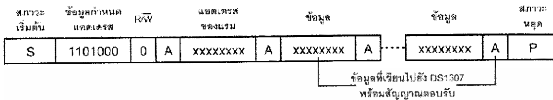
รูปที่ 3.24 รูปแบบข้อมูลสำหรับติดต่อกับ DS1307 ในโหมดการเขียนข้อมูล
