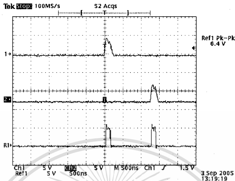
รูปที่ 4.16 สัญญาณที่ได้จากวงจรรวมสัญญาณ เปรียบเทียบกับสัญญาณอินพุต เมื่อทำการตัดวงจรที่ปลายสาย
