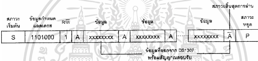
รูปที่ 3.25 รูปแบบข้อมูลสำหรับติดต่อกับ DS1307 ในโหมดการอ่านข้อมูล
