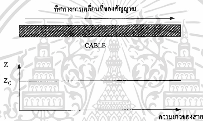
รูปที่ 2.13 การเคลื่อนที่ของสัญญาณพัลส์ในสายดี
