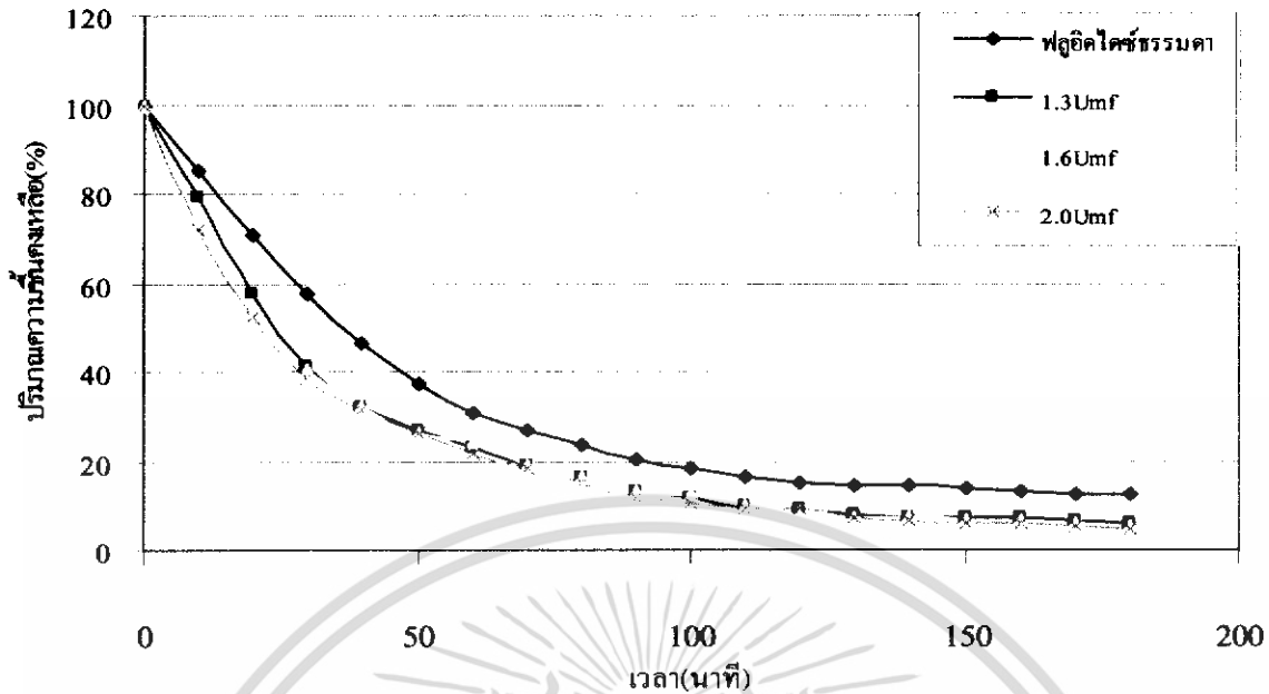
รูปที่ 5.13 แสดงการเปรียบเทียบปริมาณความชื้นกับเวลา ของหอยทดลองฟลูอิดไดซ์เบดแบบธรรมดา กับหอยทดลองฟลูอิดไดซ์เบดแบบลมหมุนและฝิวคลื่น จำนวนฝิวคลื่น 8 ลูก
