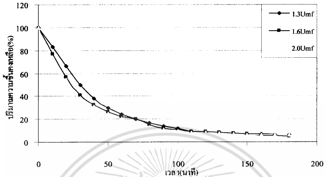
รูปที่ 5.6 กราฟเปรียบเทียบระหว่างปริมาณความเข้มข้นกับเวลา ของหอยทกกรองผิวคัตเส้น 4 ลูก ขนาด (0.3,0.4,0.5,0.6) เท่าของขนาดเส้นผ่านศูนย์กลางหอย แผ่นกระจายลมแบบใบพัด ที่ความเร็วต่างๆ
