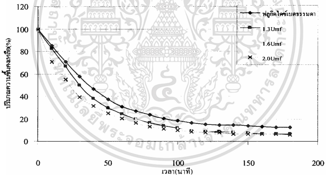
รูปที่ 5.14 แสดงการเปรียบเทียบปริมาณความชื้นกับเวลา ของหอยทดลองฟลูอิดไดซ์เบดแบบธรรมดา กับหอยทดลองฟลูอิดไดซ์เบดแบบลมหมุนและฝิวคลื่น จำนวนฝิวคลื่น 4 ลูก
