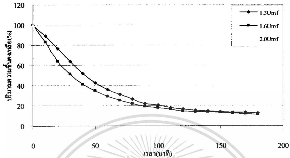
รูปที่ 5.2 กราฟเปรียบเทียบระหว่างปริมาณความชื้นกับเวลา ของหอตดลองแบบผิวกลั่น 8 ลูก ขนาด (0.3,0.35,0.4,0.45,0.5,0.55,0.6,0.65) เท่าของขนาดเส้นผ่านศูนย์กลางห่อ แผ่นกระจายลมธรรมชาติ ที่ความเร็วต่างๆ
