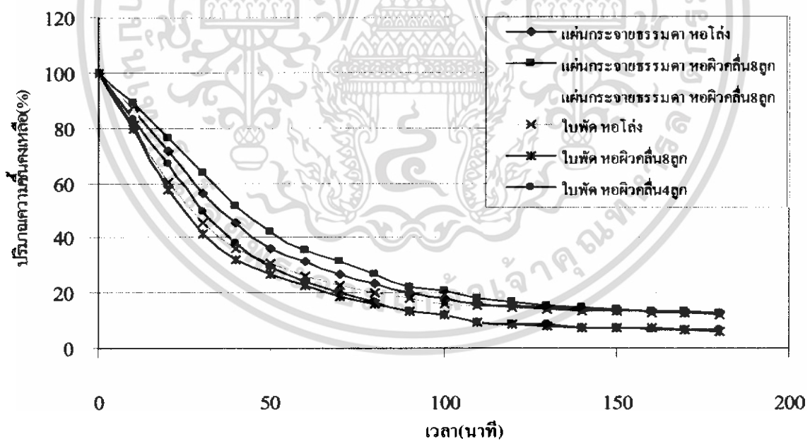
รูปที่ 5.7 กราฟเปรียบเทียบระหว่างปริมาณความเข้มข้นกับเวลา ของหอยทกกรองลักษณะต่างๆ ที่ความเร็วลม 1.3 Umf
