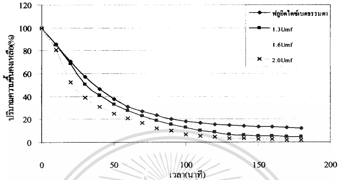
รูปที่ 5.11 แสดงการเปรียบเทียบปริมาณความชื้นกับเวลา ของหอตลอดฟลูอิดโค้เบคแบบธรรมดา กับหอตลอดฟลูอิดโค้เบคแบบผิวคลื่น จำนวนผิวคลื่น 4 ลูก
