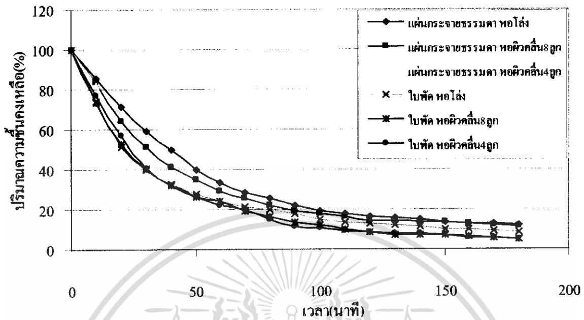
รูปที่ 5.8 กราฟเปรียบเทียบระหว่างปริมาณความชื้นกับเวลา ของหอตลอดลักษณะต่างๆ ที่ความเร็วลม 1.6 Umf
