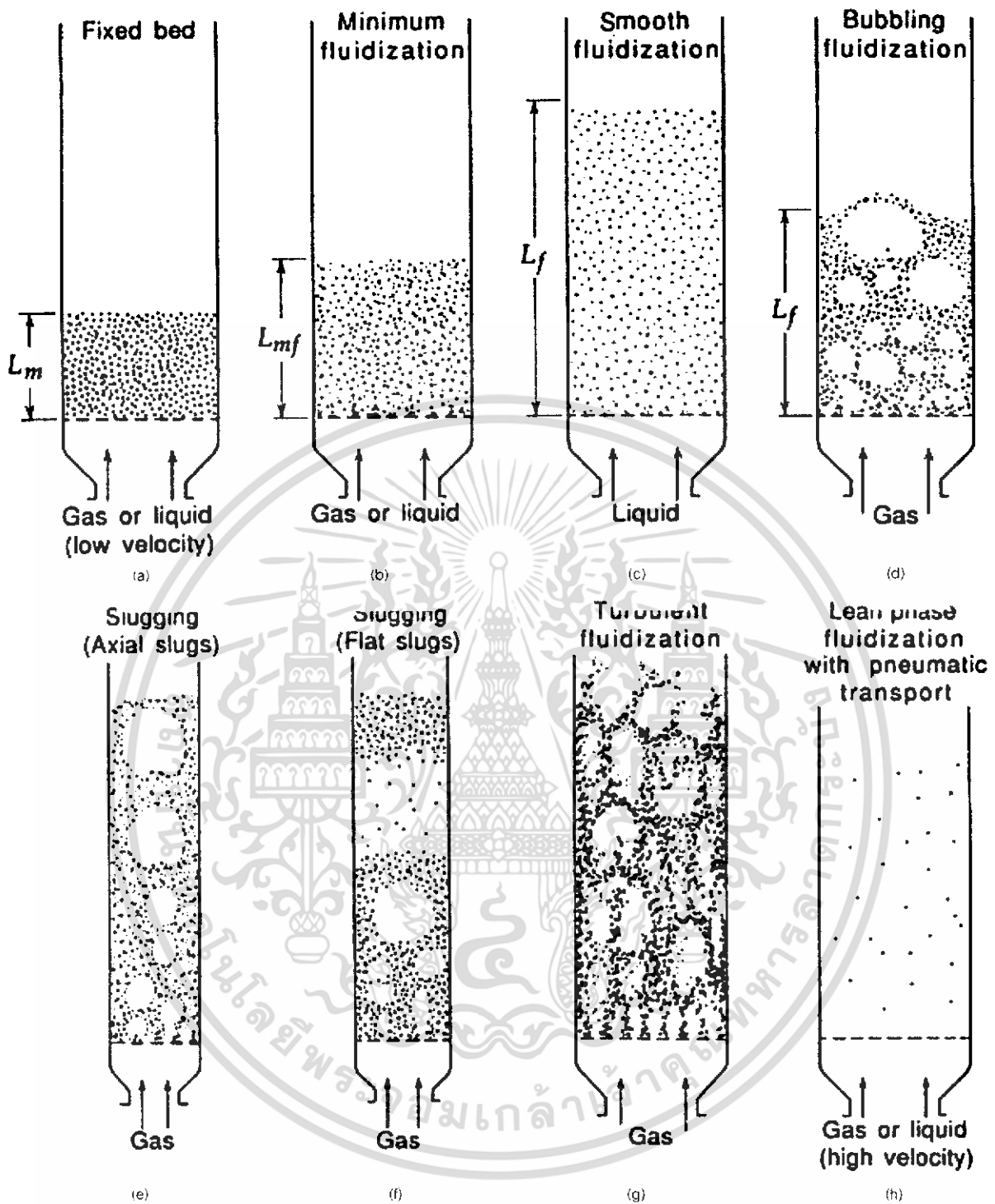
รูปที่ 3.2 พฤติกรรมการเกิดฟลูอิดไดเซชัน [Daizo Kunii, 1991]
