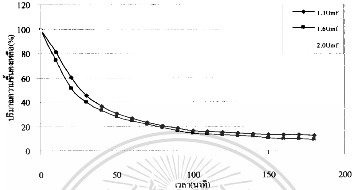
รูปที่ 5.4 กราฟเปรียบเทียบระหว่างปริมาณความชื้นกับเวลา ของหอยทอคลองแบบโล่งแผ่นกระจายลมแบบไบพัด ที่ความเร็วต่างๆ
