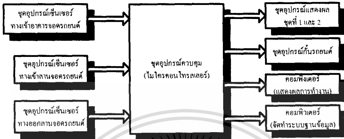
รูปที่ 3.2 ระบบการทำงานของอุปกรณ์ในส่วนของตำแหน่งทางเข้าของอาคารจอร์ถยนต์ และในส่วนของตำแหน่งทางเข้าและทางออกของลานจอร์ถยนต์
