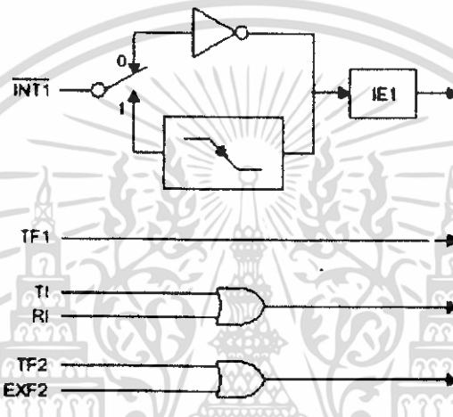
รูปที่ 2.12 โครงสร้างระบบอินเทอร์รัปต์ของ 8051
