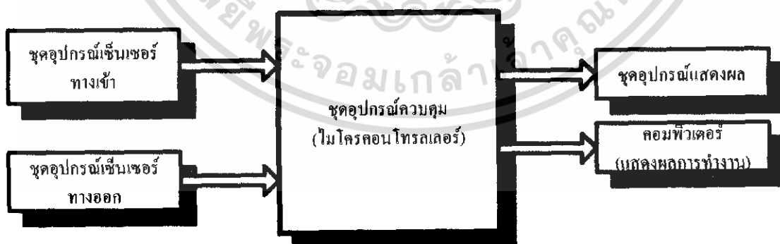
รูปที่ 3.3 ระบบการทำงานของอุปกรณ์ในส่วนของตำแหน่งทางเข้าและทางออกของแต่ละแถวหรือช่องทางจอร์ถยนต์
