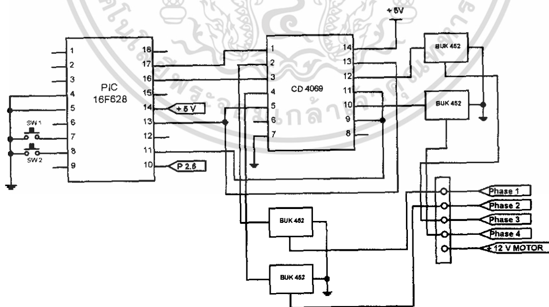
วงจรมอเตอร์ควบคุมการปิด-เปิดกันรยยนต์
