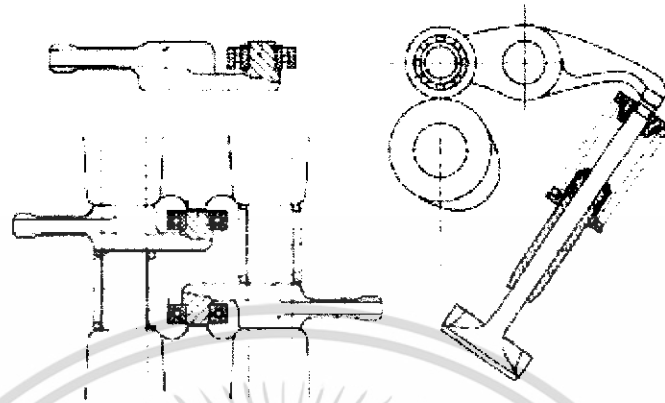
รูปที่ 3.2 ส่วนประกอบของกระดิ่งกวางตัวแบบติดตั้งโรลเลอร์ของ Tokuo
