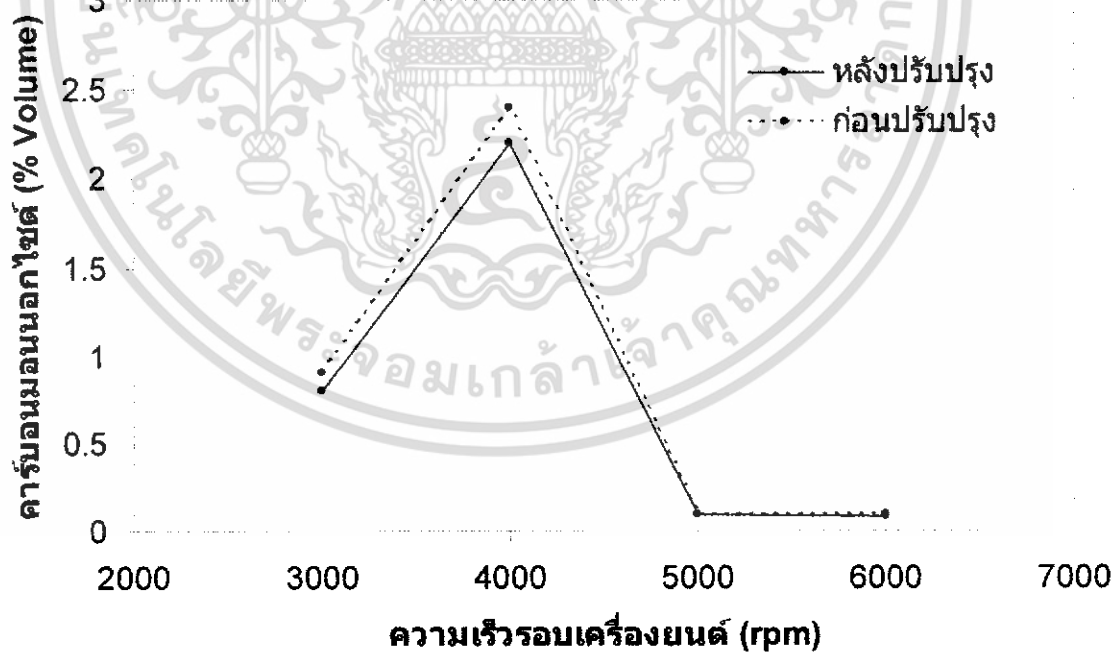
รูปที่ 5.11 ร้อยละ โดยปริมาตรของคาร์บอนมอนอกไซด์ที่ความเร็วรอบเครื่องต่างๆ ที่ภาวะ 500 kPa
