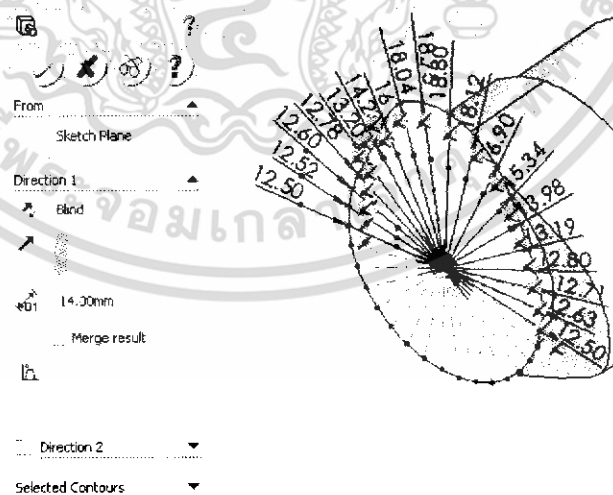
รูปที่ 5ก การทำเส้นร่างของลูกเบี้ยวสำหรับระบบไอดี
