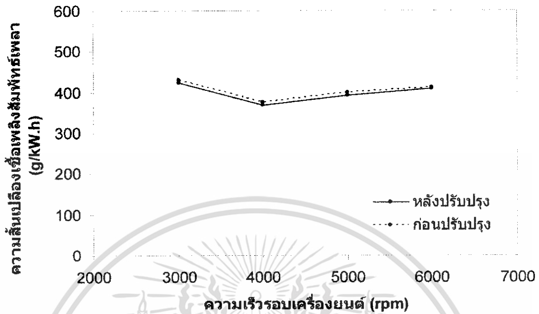
รูปที่ 5.2 ความสิ้นเปลืองเชื้อเพลิงสัมพัทธ์เพลลาที่ความเร็วรอบเครื่องต่างๆ ที่ภาวะ 300 kPa
