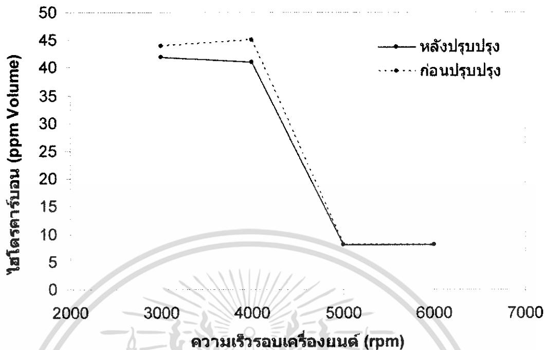
รูปที่ 5.6 ส่วนในล้านส่วนของปริมาณของไฮโดรคาร์บอนที่ความเร็วรอบเครื่องต่างๆ ที่ภาวะ 200 kPa
