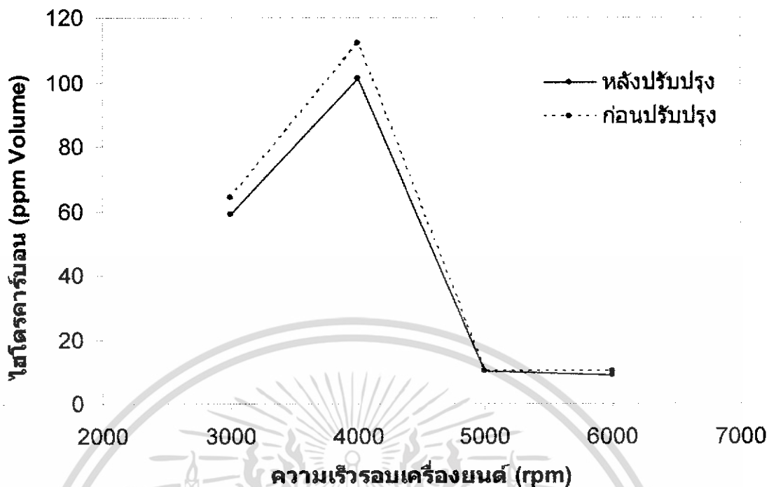
รูปที่ 5.10 ส่วนในล้านส่วนของปริมาตรของไฮโดรคาร์บอนที่ความเร็วรอบเครื่องต่างๆ ที่ภาวะ 400 kPa
