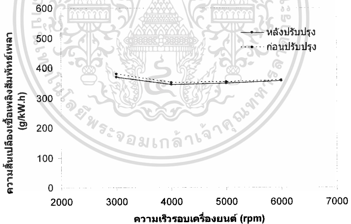
รูปที่ 5.3 ความสิ้นเปลืองเชื้อเพลิงสัมพัทธ์เพลลาที่ความเร็วรอบเครื่องต่างๆ ที่ภาวะ 400 kPa
