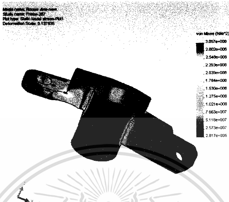
รูปที่ 22ก การวิเคราะห์ความเค้นสมมูลโดยใช้ COSMOSWorks ในจังหวะที่เกิดแรงกระทำสูงสุด
