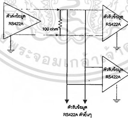
รูปที่ 5.10 โครงสร้างการสื่อสารข้อมูลแบบอนุกรมตามมาตรฐาน RS-422A
