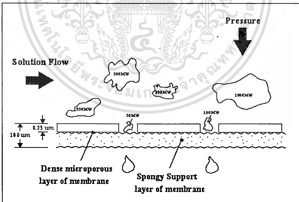
รูปที่ 2.6 กลไกการกำจัดสารอินทรีย์ของระบบออสโมซิสย้อนกลับ
