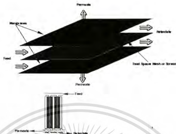
รูปที่ 3.1 RO-Plate and Frame Module
