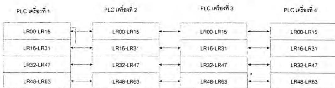
รูปที่ 5.18 การแบ่งพื้นที่สำหรับ PC Link System
