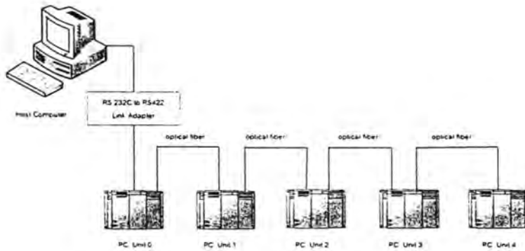
รูปที่ 5.16 การต่อแบบ Serial Link
