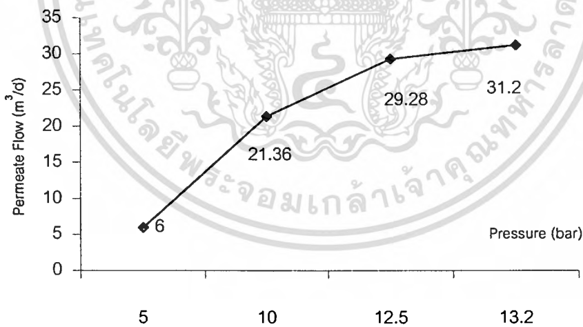
รูปที่ 2.3 ผลของแรงดันที่มีต่อปริมาณน้ำสะอาดที่ผลิตได้
