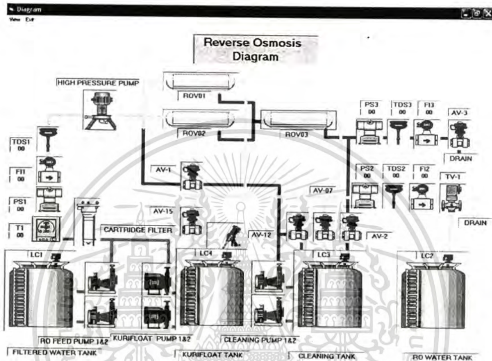
รูปที่ 8.3 แสดงหน้าจอควบคุมระบบออสโมซิสย้อนกลับที่ใช้ในโรงงานโรงแป้งน้ำเสีย
