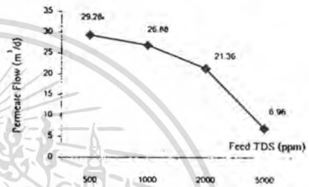
รูปที่ 4 ผลของความเข้มข้นของสารละลายต่อปริมาณน้ำ สะอาดที่ผลิตได้
