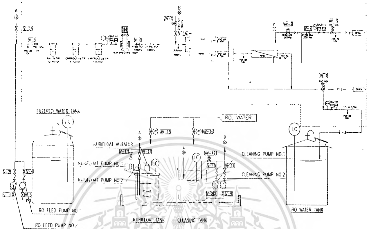
รูปที่ 6.4 ระบบออสโมซิสย้อนกลับแบบที่ได้มีการพัฒนาขึ้น
