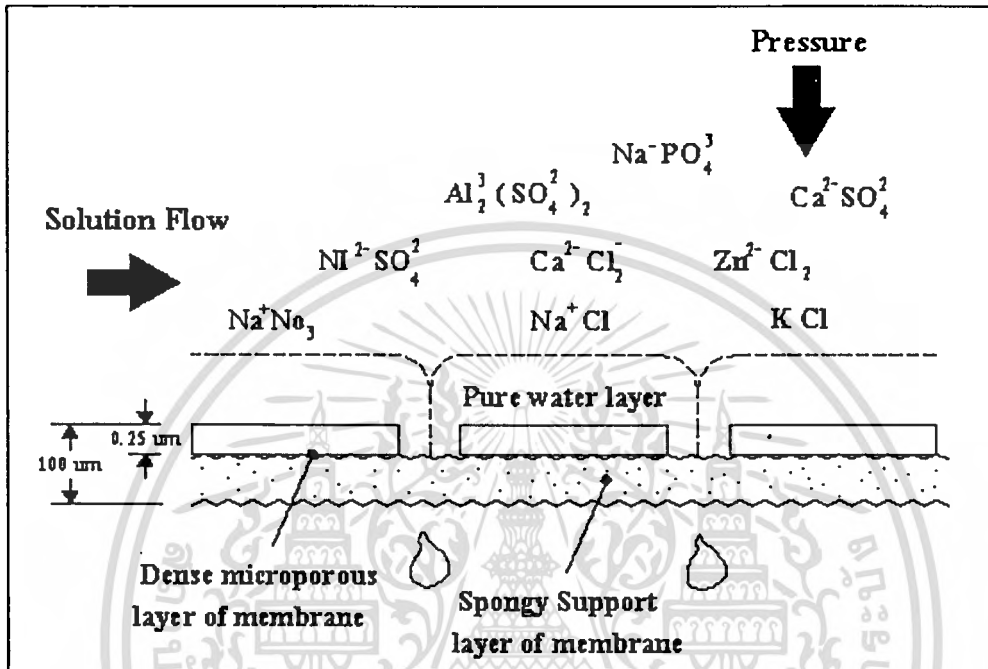
รูปที่ 2.5 กลไกการกำจัดเกลือแร่ของระบบออสโมซิสย้อนกลับ
