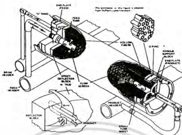
รูปที่ 3.4 RO-Hollow Fiber Module
