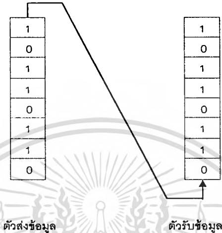
รูปที่ 5.6 การสื่อสารข้อมูลแบบอนุกรม
