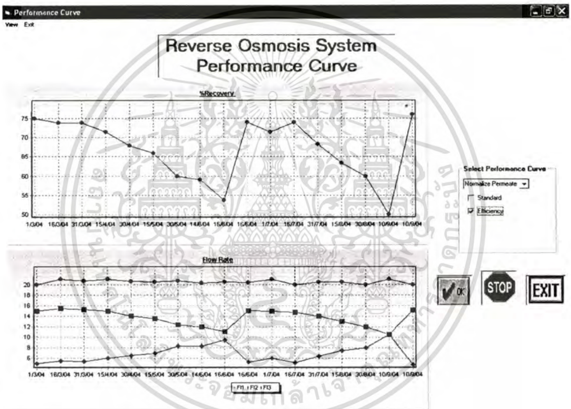
รูปที่ 8.6 แนวโน้ม Recovery (%R)
