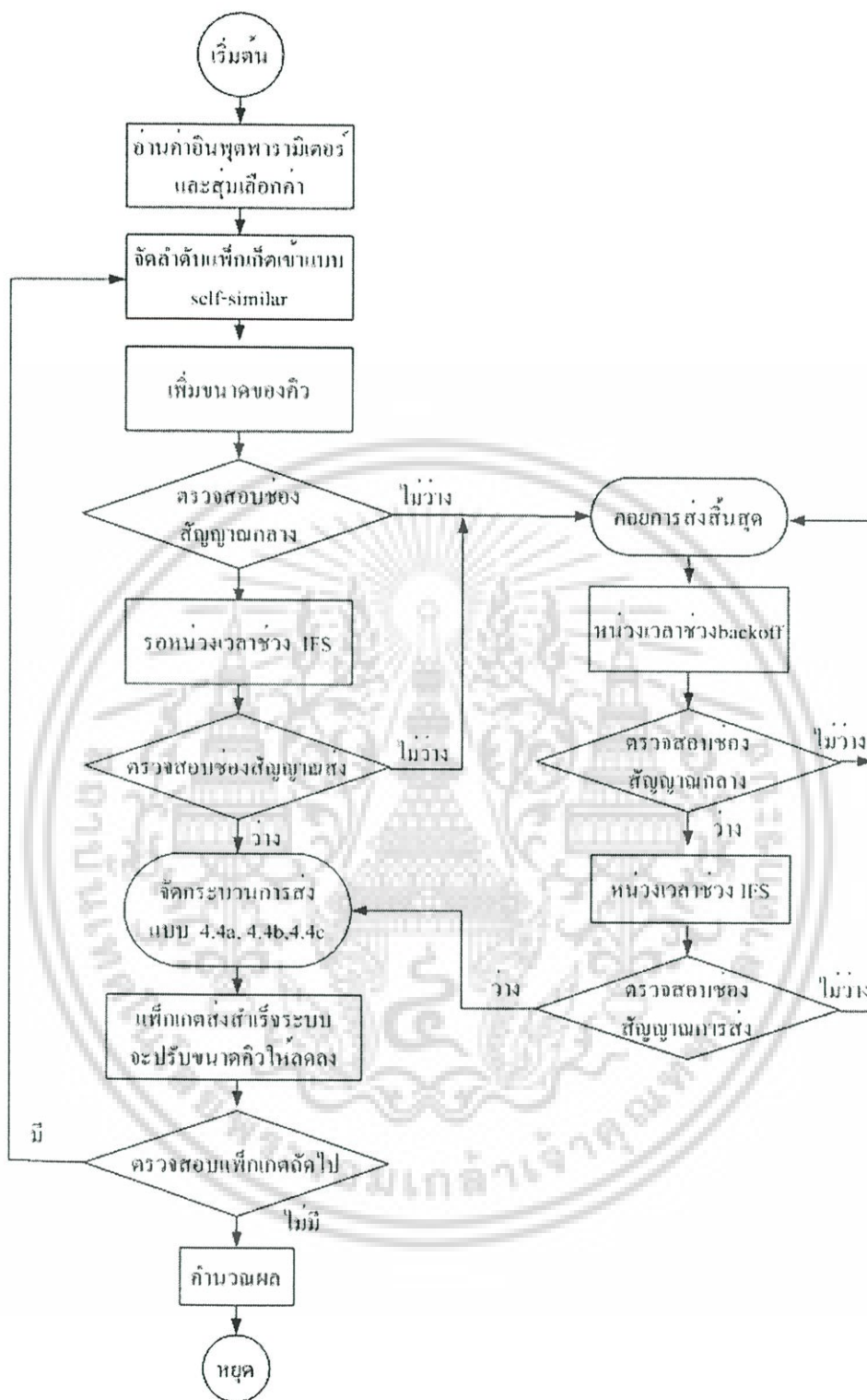
รูปที่ 4.6 โฟลวชาร์ตแสดงการจำลองแบบ CSMA/CA เมื่อมีรูปแบบการรับ-ส่งข้อมูลที่แตกต่างกัน ตามรูปแบบ 4.4a, 4.4b และ 4.4c
