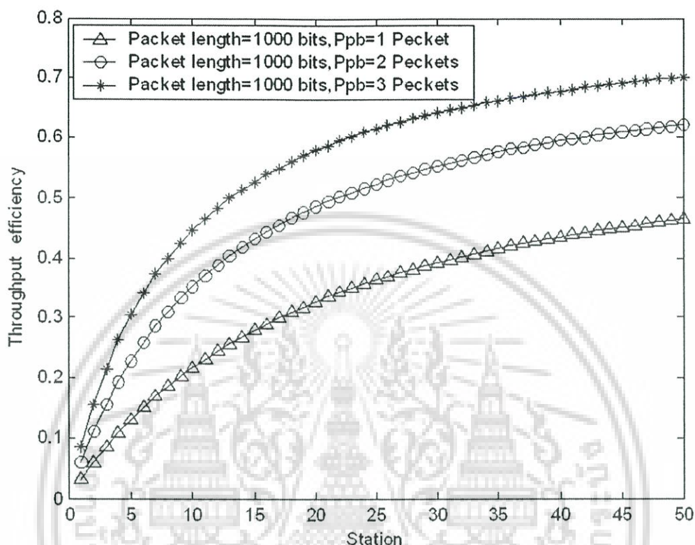
รูปที่ 5.10 จำลองระบบที่มีกราฟฟิกแบบบัวซองโดยความยาวแพ็กเก็ตคงที่ที่ 1000 บิต
