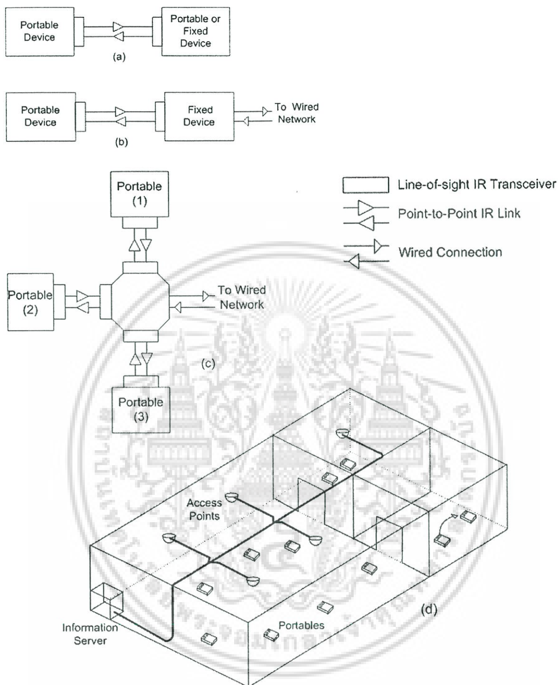
รูปที่ 2.2 แสดงชนิดของการสื่อสารระบบอินฟราเรด a) การสื่อสารแบบ Point-to-Point ในรูปแบบ LOS (หรือเป็นแบบ Point-to-Multipoint) b) การสื่อสารอินฟราเรดแบบ Point-to-Point โดยผ่าน Fixed Device จะทำการเชื่อมต่อกับโครงข่าย c) การติดต่อระหว่างผู้ใช้หลายคนพร้อมกันด้วยอุปกรณ์ Hub ซึ่งการเชื่อมต่อเป็นแบบ Point-to-Point และ อีกด้านเป็นการเชื่อมต่อกับโครงข่ายที่ใช้สาย d) คือรูปแบบของ LAN ที่มีการเข้าแบบหลายทางเพื่อติดต่อกับผู้ใช้หลายคนผ่านโครงข่ายแบบมีสาย, การติดต่อระหว่างผู้ใช้กับ
