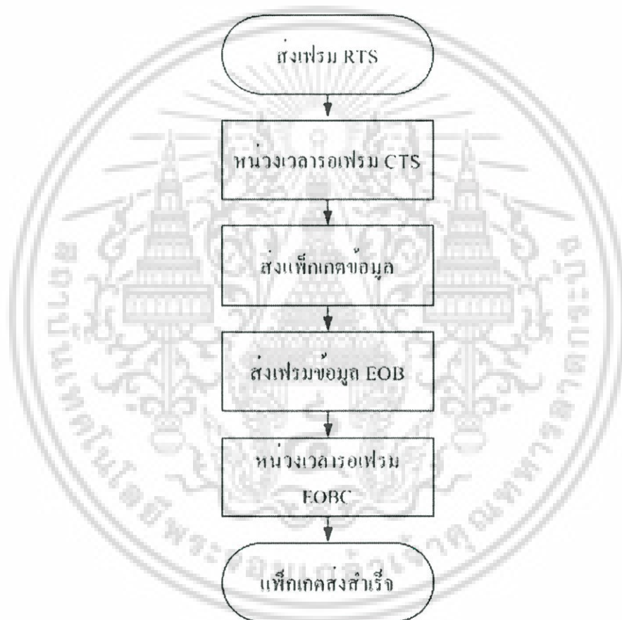
รูปที่ 4.10 โฟลว์ชาร์ตการ รับ-ส่ง ข้อมูลทั้งหมดโดยมีการตรวจสอบข้อมูลเพียงครั้งเดียว ด้วยการรอแพ็กเก็ต EOBC ในขั้นตอนสุดท้ายดังรูปที่ 4.4b
