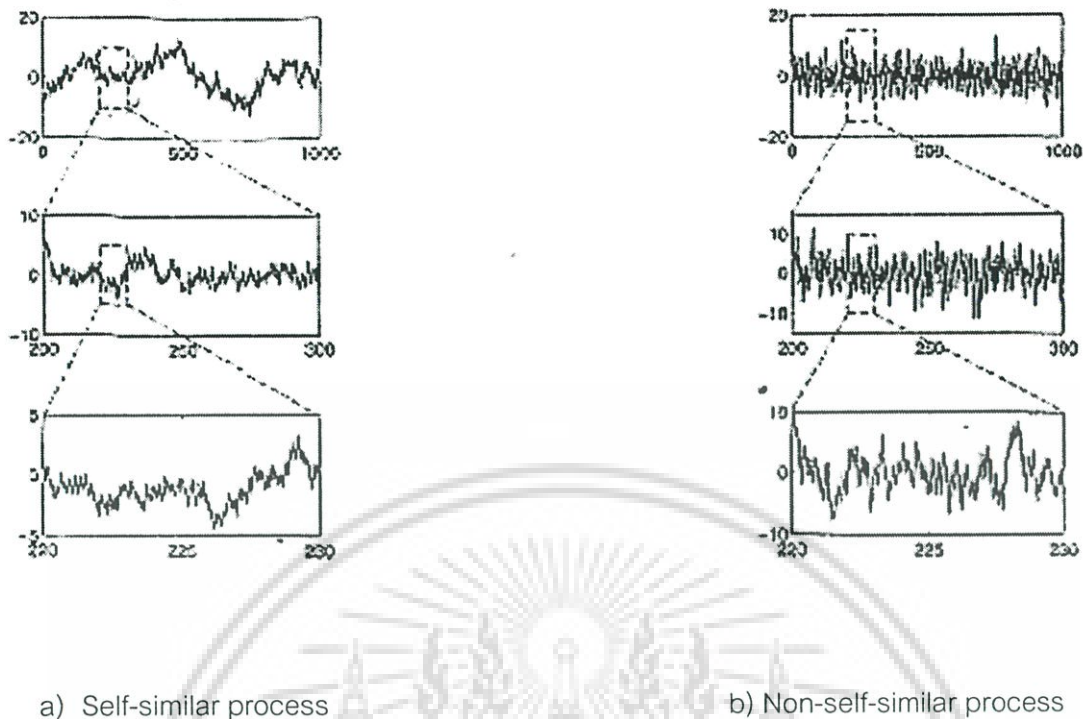
รูปที่ 3.3 ภาพเปรียบเทียบผลข้อมูลที่ผ่านมาเข้ามาในระบบเมื่อทำการขยายสเกลระหว่างกราฟฟิก ข้อมูลที่เป็น Self-similar และกราฟฟิกข้อมูลที่เป็น Non-self-similar
