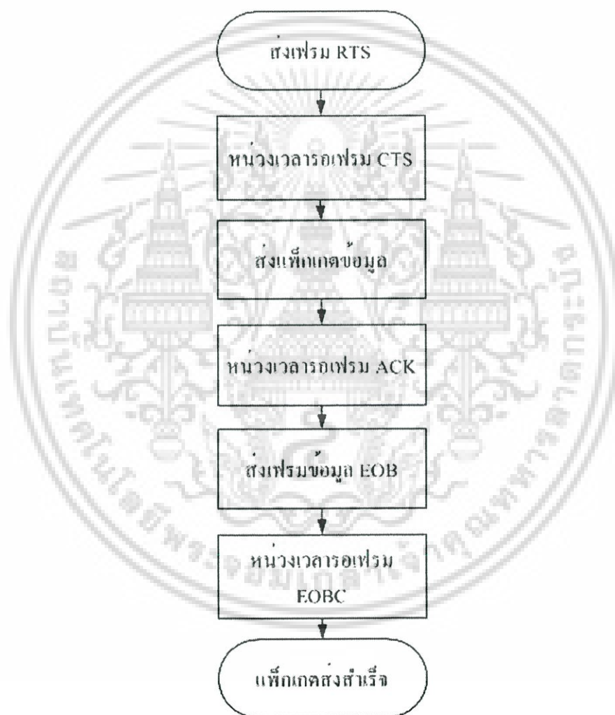
รูปที่ 4.8 โฟลว์ชาร์ตการ รับ-ส่ง ข้อมูลเมื่อมีการตรวจสอบการส่งข้อมูลที่ส่งด้วยแพ็กเก็ต ACK ดังขั้นตอนของรูปที่ 4.4a
