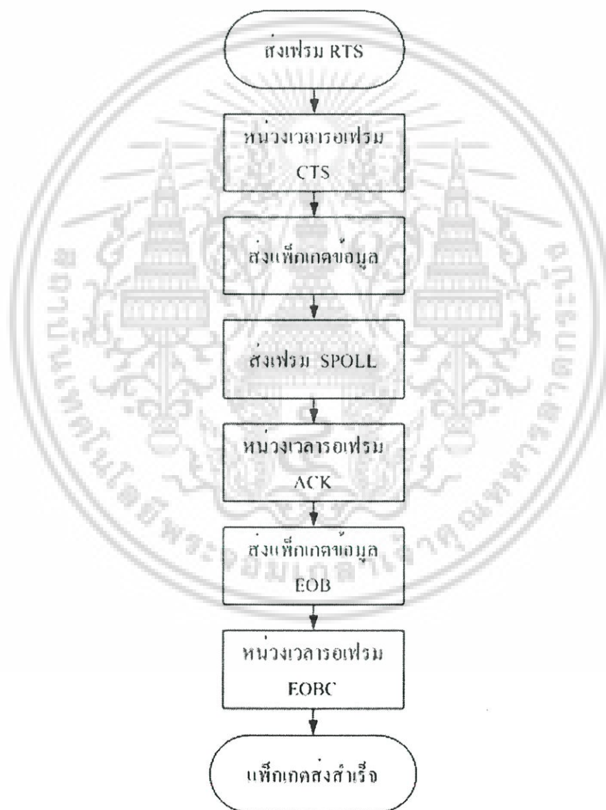
รูปที่ 4.12 โฟลว์ชาร์ตการ รับ-ส่ง ข้อมูลทั้งหมดโดยมีการตรวจสอบข้อมูลเพียงทุกครั้งที่มีการส่งข้อมูลด้วยการส่งแพ็กเก็ต SPOLL ดังแสดงในรูปที่ 4.4c
