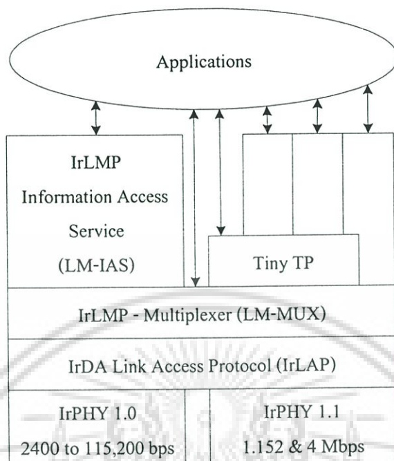
รูปที่ 2.3 แบบจำลองโพรโตคอล IrDA
