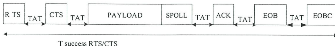
รูปที่ 4.11 แบบจำลองรูปแบบการรับ-ส่ง ข้อมูล ตามรูปที่ 4.4c
