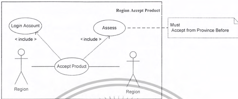
รูปที่ 3.6 ยูสเคส ไดอะแกรมสำหรับการยอมรับผลิตภัณฑ์ระดับภาค ( Region Accept )
