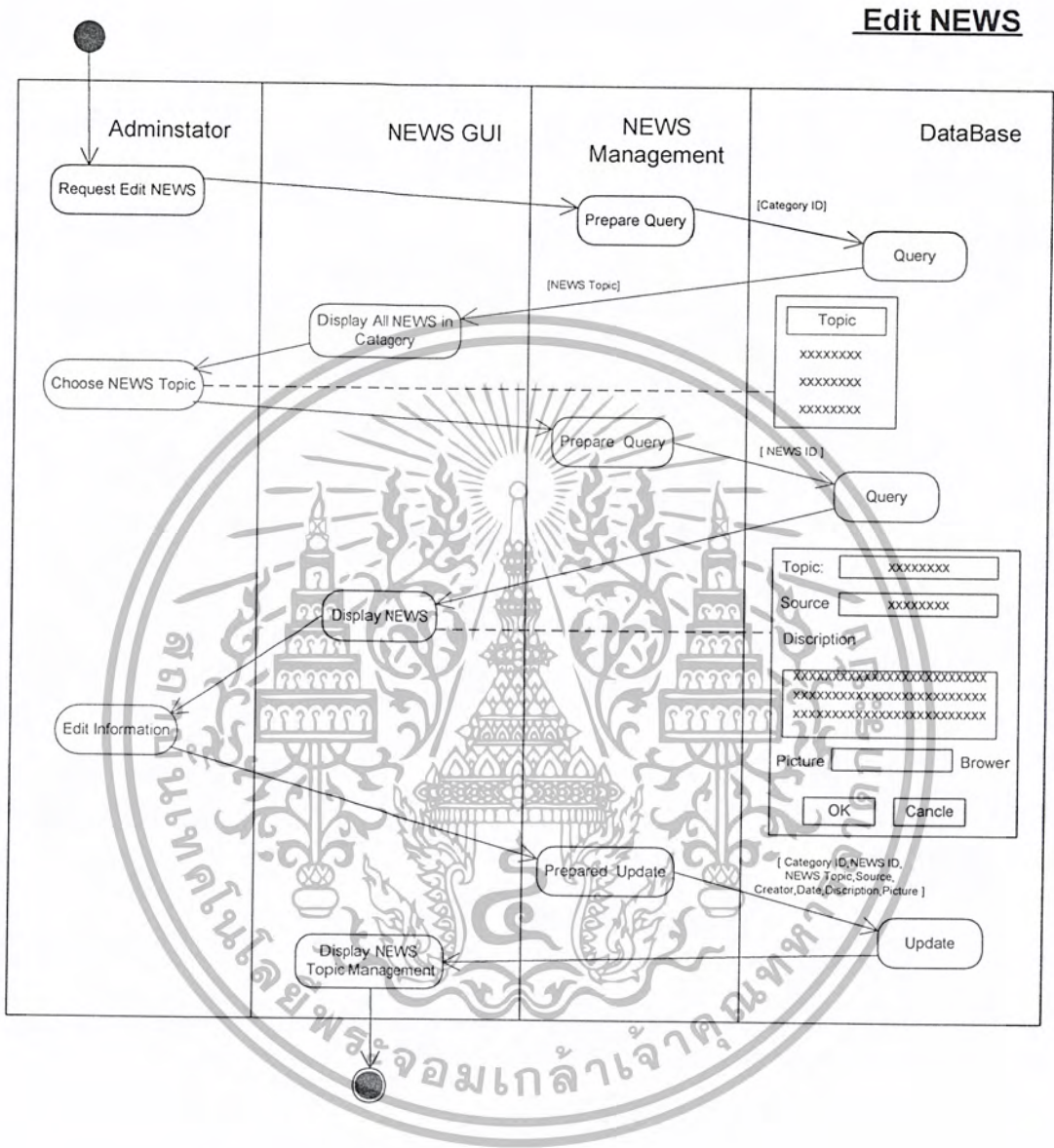
รูปที่ 3.33 แอกทิวิตี้ไดอะแกรมสำหรับแก้ไขข่าวสาร (Edit NEWS)
