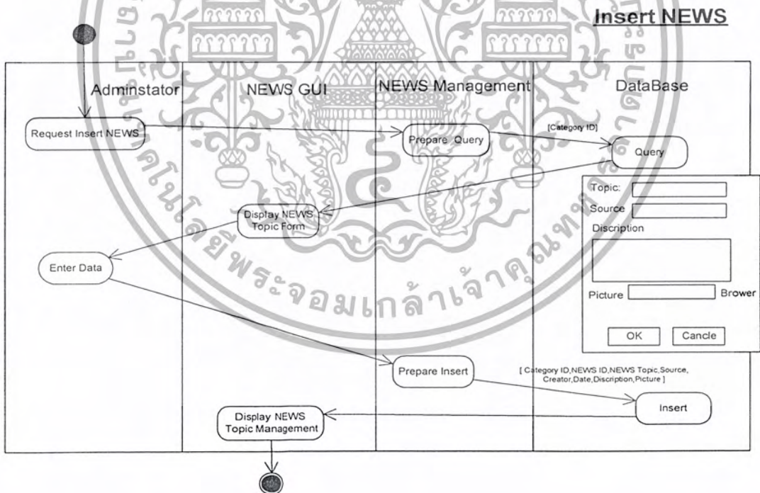
รูปที่ 3.32 แอทวิตตี้ไดอะแกรมสำหรับเพิ่มข่าวสาร ( Insert NEWS )
