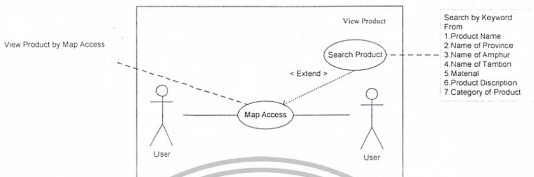
รูปที่ 3.8 ยูสเคสไดอะแกรมสำหรับบริการดูรายละเอียดของผลิตภัณฑ์ ( View Product )
