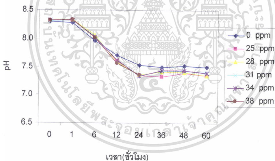
ภาพที่ 5 การเปลี่ยนแปลงค่าความเป็นกรดเป็นด่าง ในระหว่างการทดลองหาความเป็นพิษ เฉียบพลันของ benzocaine ต่อปลาสดภายในระยะเวลา 60 ชั่วโมง
