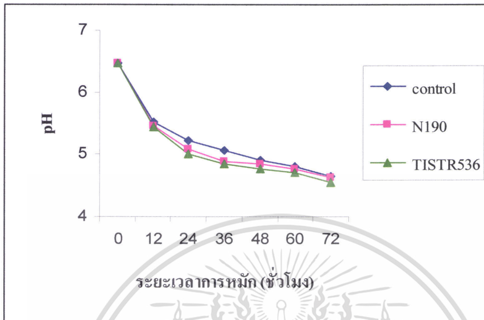
รูปที่ 3 กราฟเปรียบเทียบแนวโน้มการลดลงของค่าพีเอชในตัวอย่างเหวม ในระยะเวลาการหมักเหวม ที่ชั่วโมงต่างๆ
