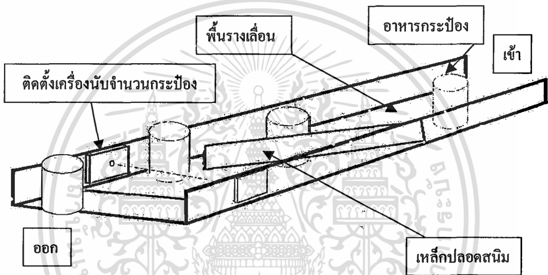
ภาพที่ 8 ตำแหน่งที่ควรติดตั้งเครื่องนับกระป๋อง
