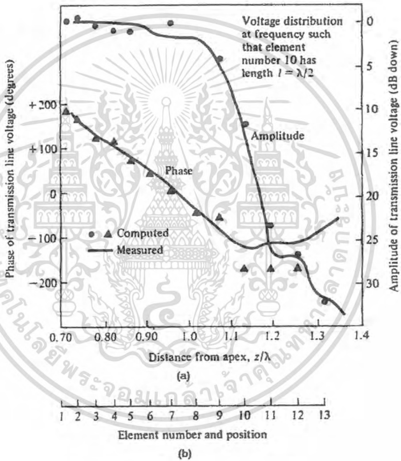
รูปที่ 2.7 (a) แรงดันในแนวนอนของตัวพีคเคอร์ของสายอากาศสายคาบลือก (b) ตำแหน่งขององค์ประกอบที่สัมพันธ์กัน
