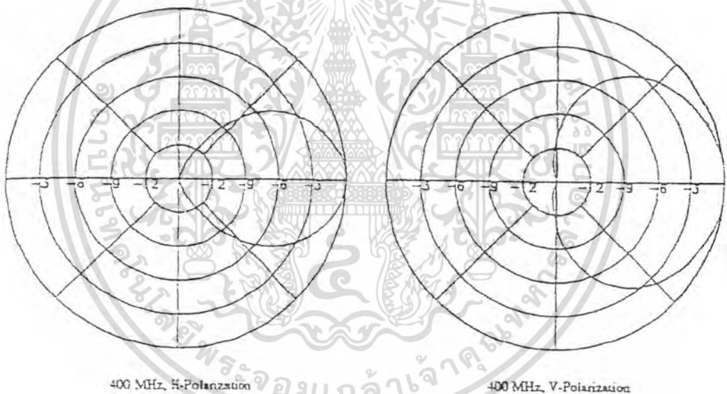
รูปที่ 2.9 แบบรูปการกระจายคลื่นของสายอากาศสายคาบถ็อก
