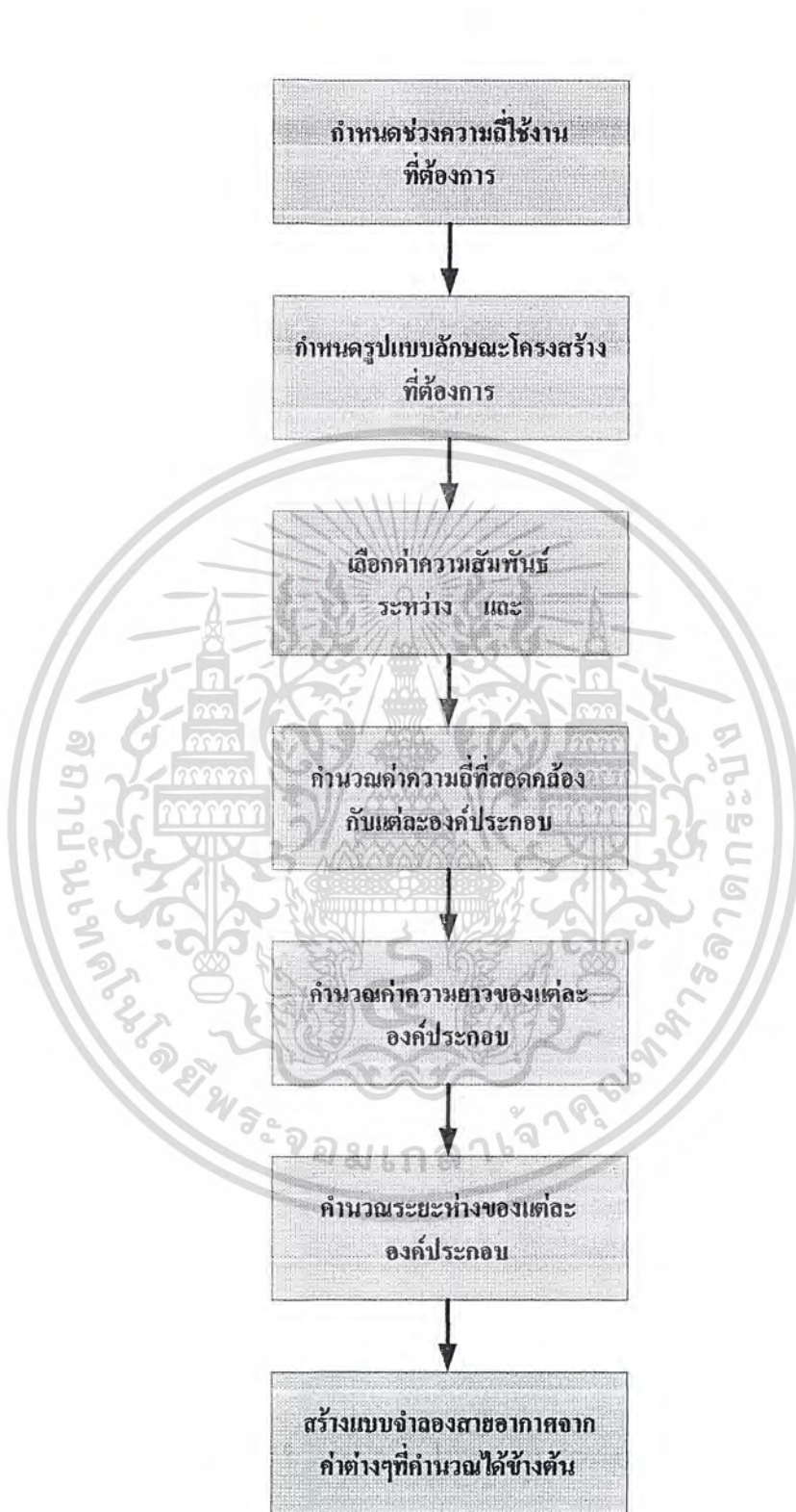
รูปที่ 3.1 แผนผังแสดงขั้นตอนการออกแบบสายอากาศสายคาบสลับบนวัสดุฐานรองไดอิเล็กตริก
