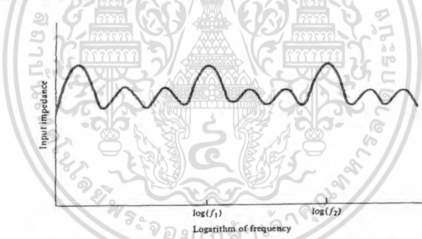
รูปที่ 2.2 การเปลี่ยนแปลงค่าอินพุทอิมพีแดนซ์ของสายอากาศแบบรายคาบล็อก ซึ่งเป็นฟังก์ชันลอการิทึมของความถี่
