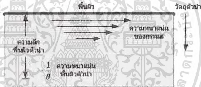
รูปที่ 2.11 แสดงการลดลงของความหนาแน่นกระแสเนื่องจากสกินเอฟเฟกต์
