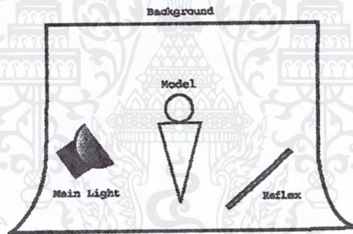
รูปที่ 2.9 แผนผังไฟหนึ่งดวง
