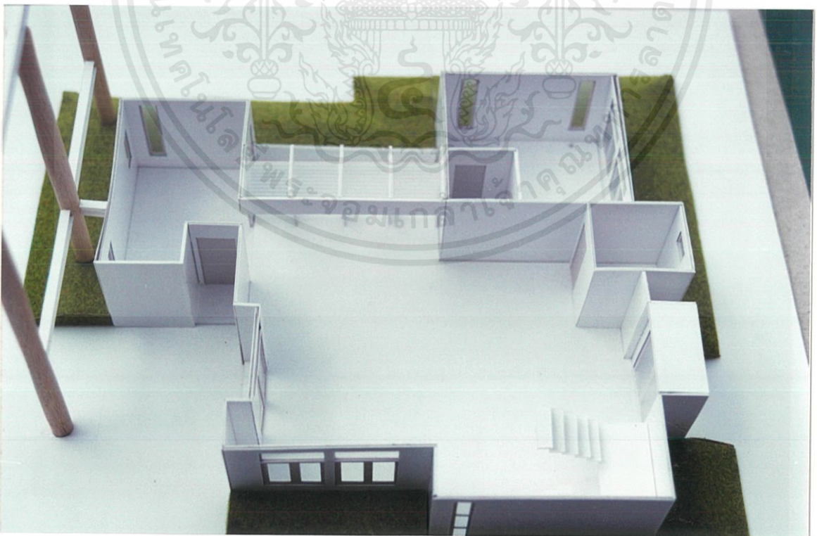
รูปที่ 4.76 แสดงหุ่นจำลองพื้นที่ชั้น 1 ส่วนเอนกประสงค์ภายในบ้านพักอาศัยกลุ่ม Loop house เอกสารนี้เป็นเอกสารที่สงวนไว้สำหรับการใช้งานเพื่อการศึกษาเท่านั้น ไม่อนุญาตให้นำไปใช้ประโยชน์ด้านการค้า ไม่ว่ากรณีใดๆ ทั้งสิ้น อีกทั้งห้ามมิให้ตัดแปลงเนื้อหาและต้องอ้างอิงถึงเจ้าของเอกสารทุกครั้งที่มีการนำไปใช้
