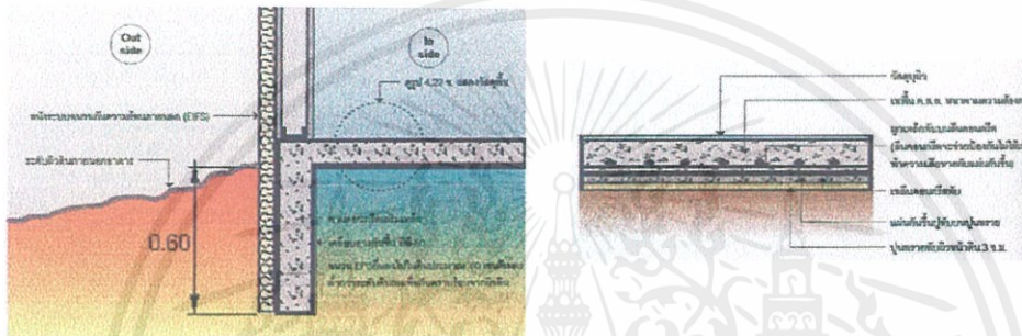
รูปที่ 3.12 ลักษณะการป้องกันความชื้นจากผิวดินเข้าสู่ภายใน
