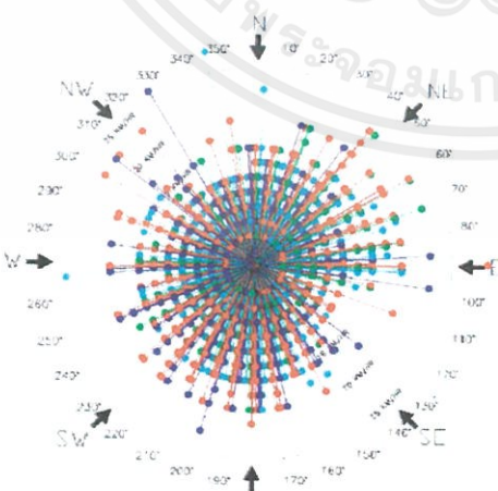
รูปที่ 2.2 แสดงทิศทางลมในประเทศไทย
