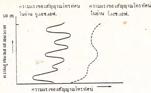
(ก) สำหรับโทรทัศน์ในย่านยู.เอช.เอฟ. ความแรงของสัญญาณโทรทัศน์จะขึ้นอยู่กับความสูงของเสาอากาศ ส่วนโทรทัศน์ในย่านวี.เอช.เอฟ. ความแรงของสัญญาณโทรทัศน์จะขึ้นอยู่กับความสูงของเสาอากาศเหมือนกัน แต่จะไม่มีการเปลี่ยนแปลงมาก
