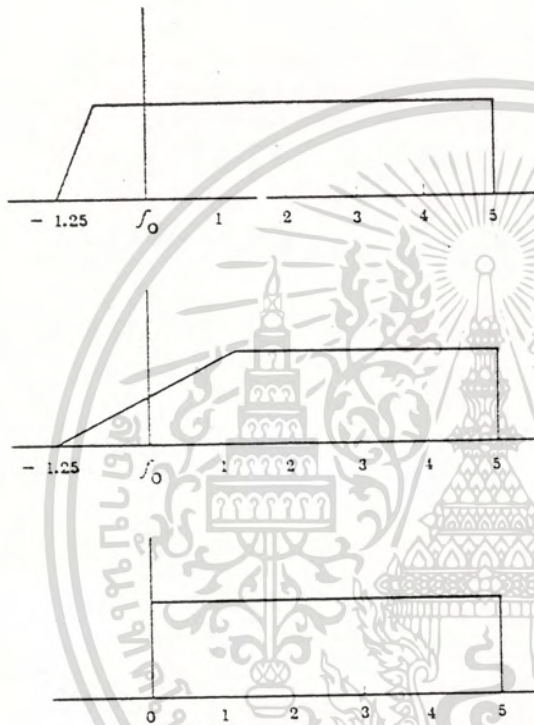
รูปที่ 2-2-2 หลักการใช้ในเครื่องส่งและเครื่องรับโทรทัศน์ ในระบบ vestigial sideband transmission.
