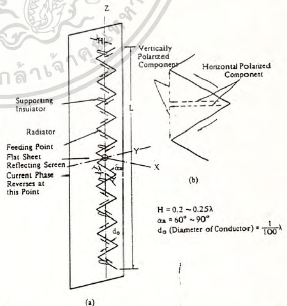
Fig. 3.28 Zig-Zag Antenna
