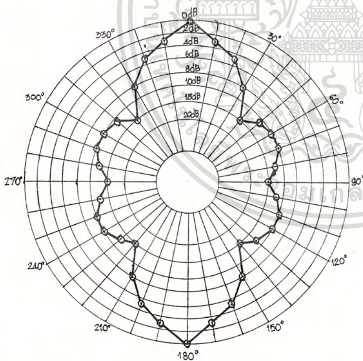
รูป 4-6 Pattern Loop Antenna
