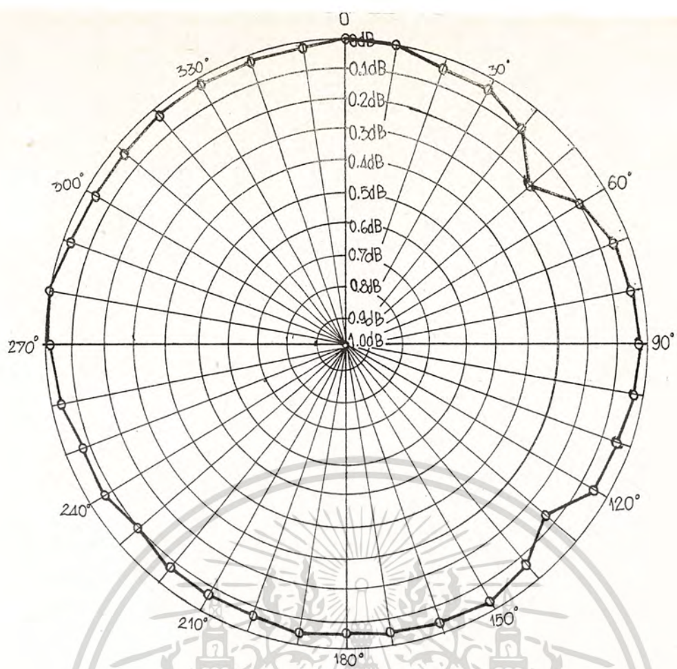
รูป 4-6 Pattern Loop Antenna
