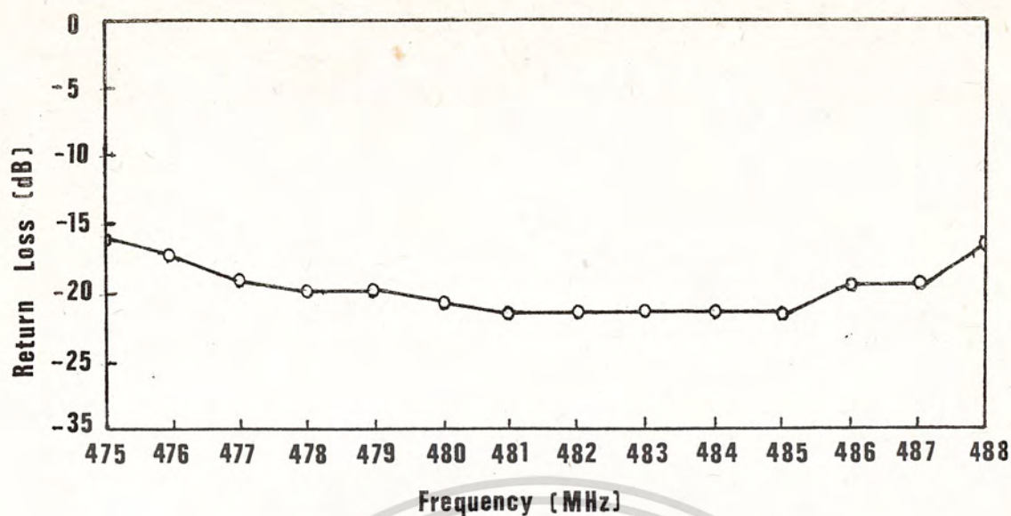
รูป 4-2 กราฟความสัมพันธ์ระหว่างความถี่ต่าง ๆ กับ Return Loss
