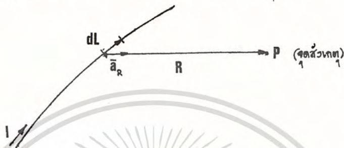
รูปที่ 2-3-1 แสดงหลักการของบิโอต์ซาวาร์ต
