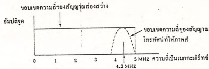
รูปที่ 2-2-1 ขอบเขตความดีของสัญญาณส่องสว่าง และของสัญญาณโทรทัศน์ที่ให้ภาพสี.
