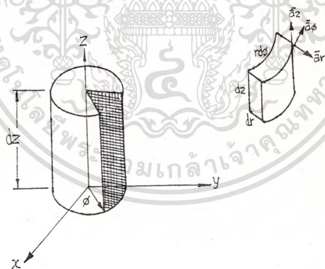
รูปที่ 2-3-2 กระแสไหลผ่านเส้นลวดยาวมาก
