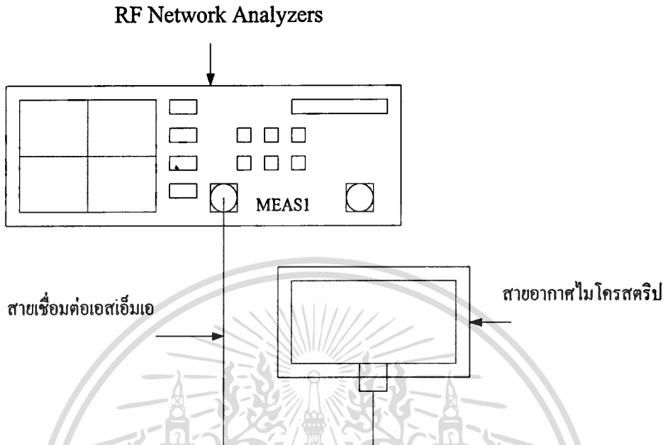
รูปที่ 5 การต่อสายอากาศไมโครสตริปกับเครื่องมือวัด
