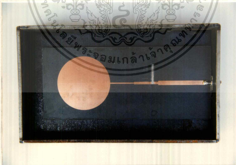
รูปที่ ก.12 สายอากาศไมโครสตริปแบบวงกลมที่มีสารตัวกลางเป็นดูรอยด์ที่ใส่ควาวิตี
