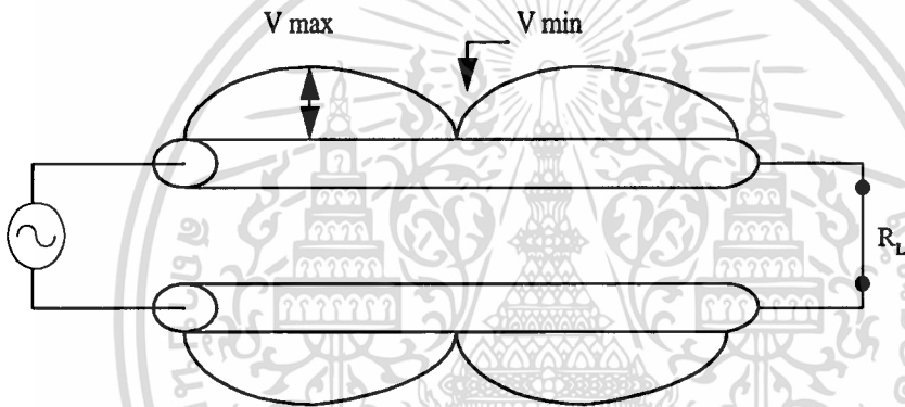
รูปที่ 2.10 จุดแรงดันสูงสุดและต่ำสุดของคลื่นนิ่ง
