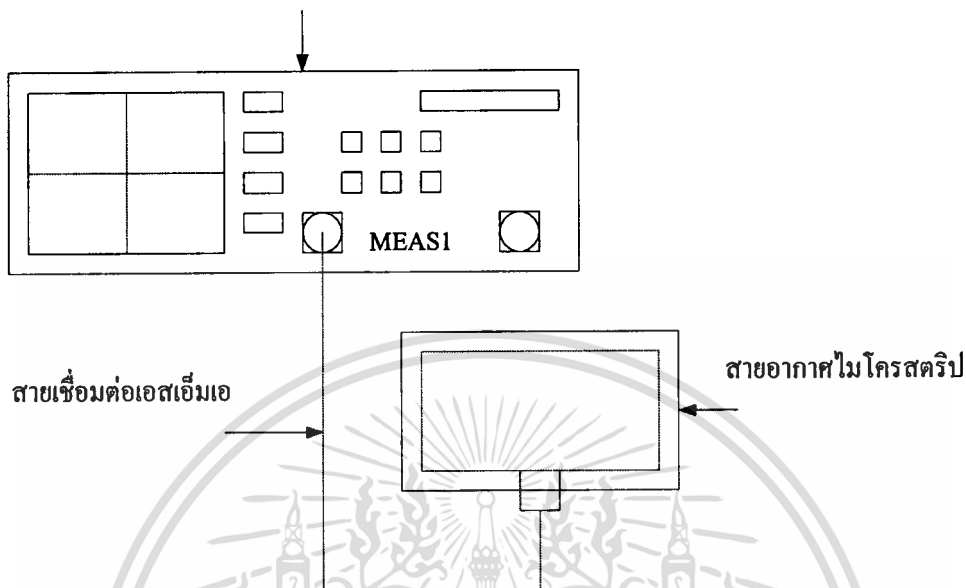
รูปที่ 2 การต่อสายอากาศไมโครสตริปกับเครื่องมือวัด
