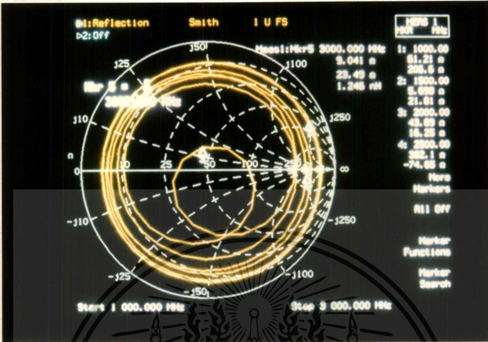
รูปที่ 4.11 แผนภาพสมิตชาร์ตค่าอิมพีแดนซ์ของสายอากาศไมโครสตริปแบบวงกลมที่มีสารตัวกลางเป็นอีพ็อกซี
