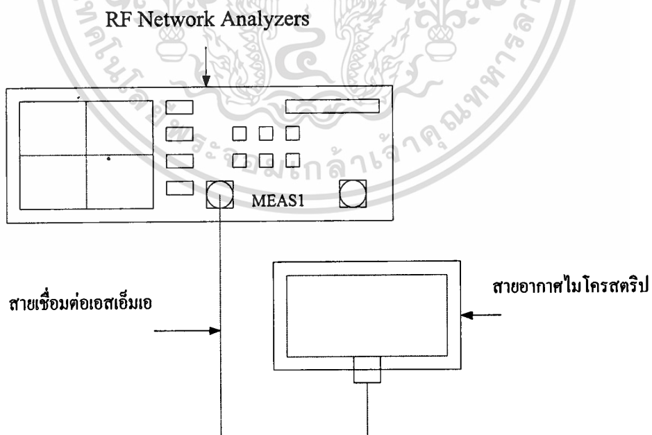
รูปที่ 20 การต่อสายอากาศไมโครสตริปกับเครื่องมือวัด
