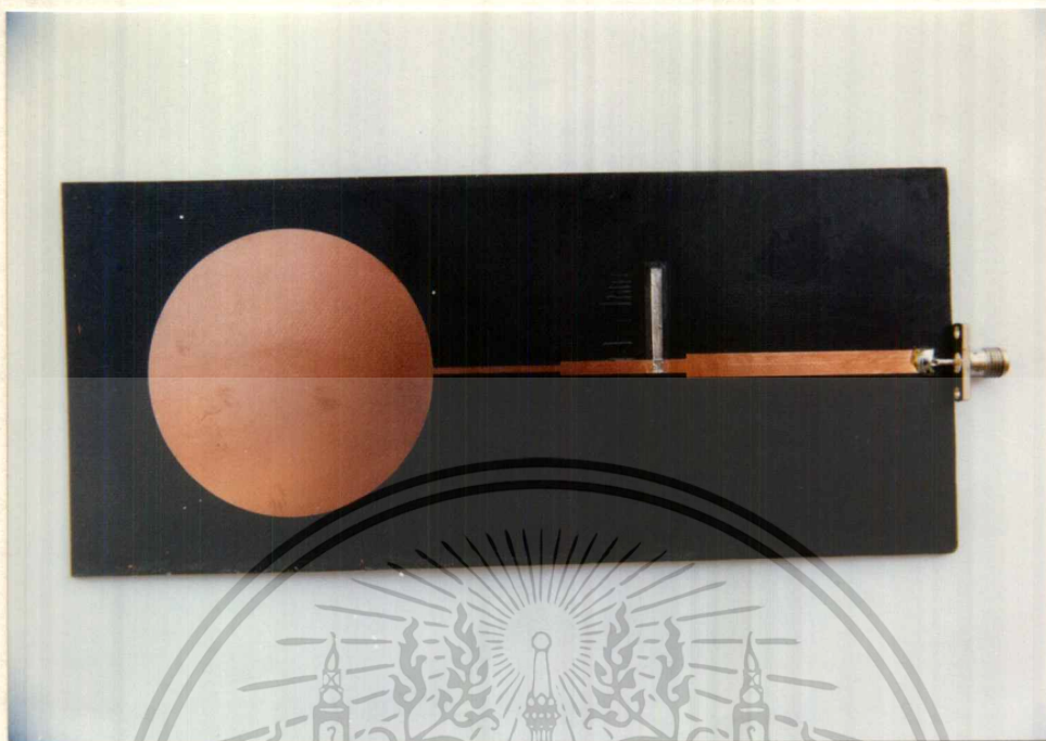
รูปที่ ก.11 สายอากาศไมโครสตริปแบบวงกลมที่มีสารตัวกลางเป็นดูรอยด์ที่ยังไม่ใส่ควาวิตี
