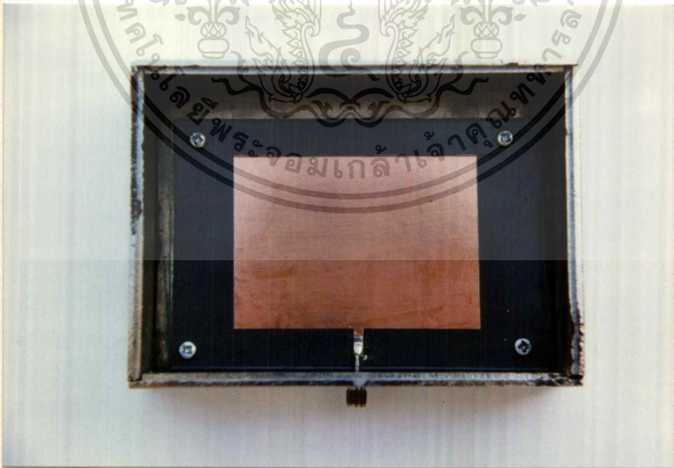
รูปที่ ก.8 สายอากาศไมโครสตริปแบบสี่เหลี่ยมที่มีสารตัวกลางเป็นฉนวนที่ใส่ค่าวิดี
