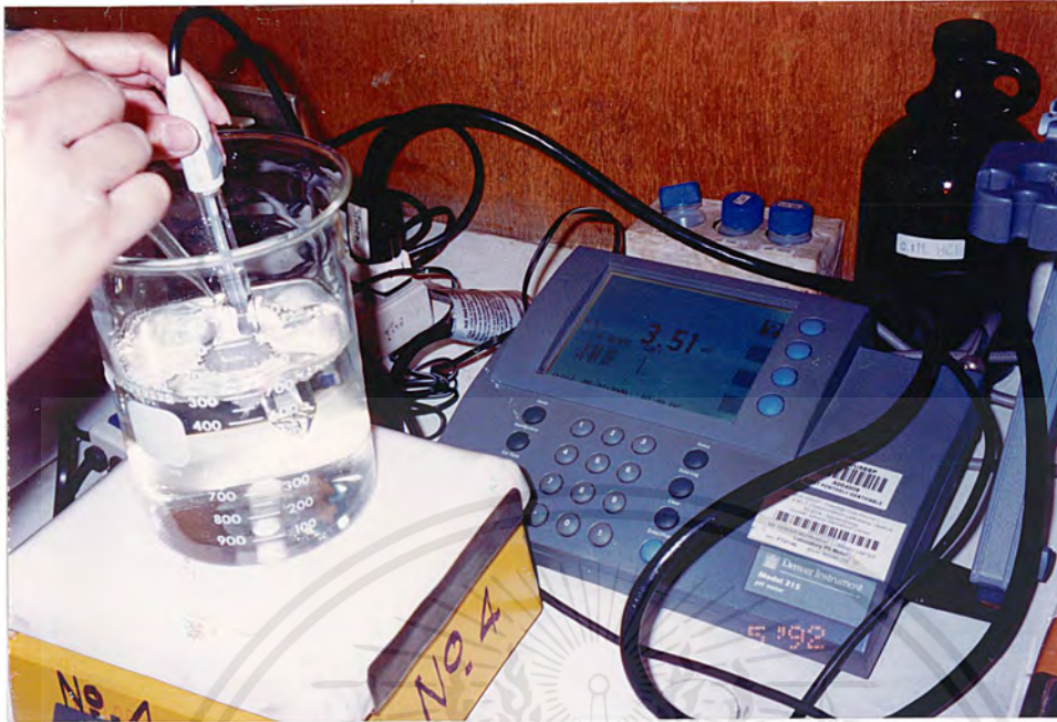
รูปที่ 2 การปรับพีเอชน้ำทิ้งโรงงานแปรรูปไก่ที่ผ่านการกรอง
