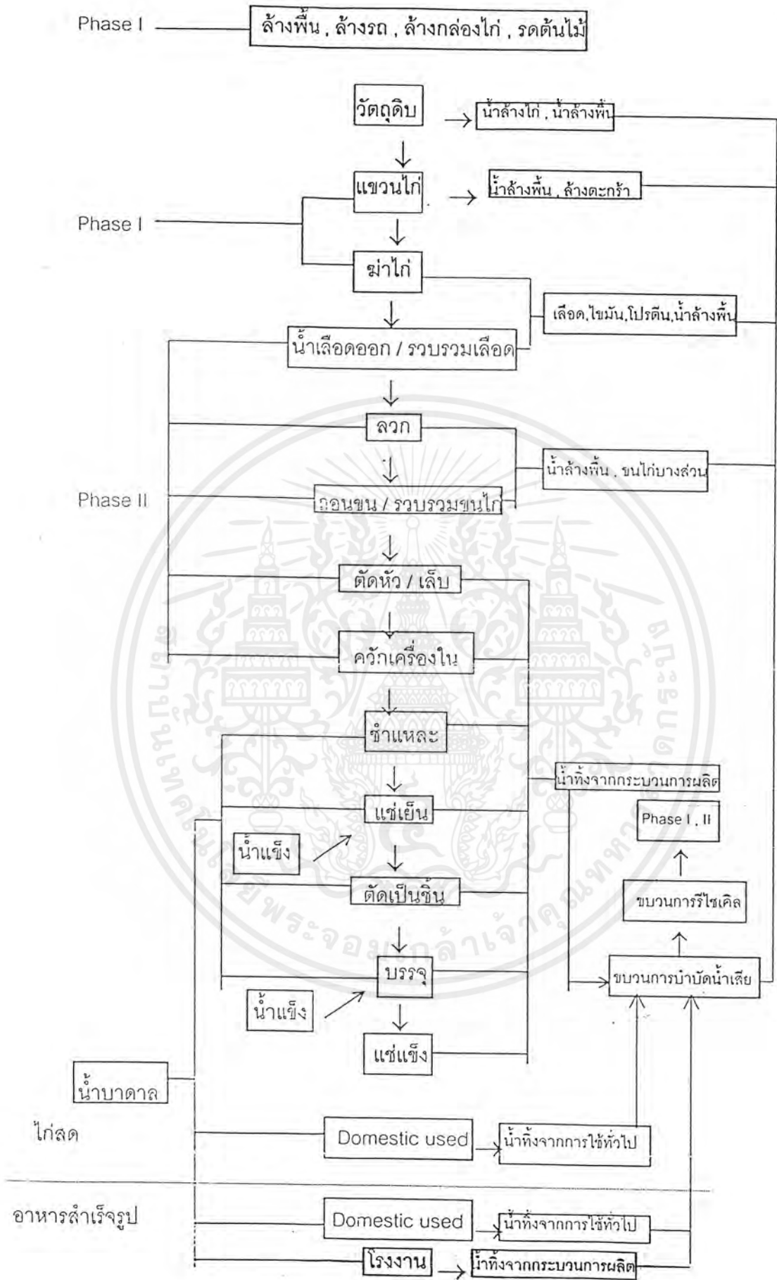
เอกสารนี้เป็น รูปที่ 1 แสดงการใช้ น้ำ / น้ำทิ้งระหว่างขั้นตอนการผลิต ไก่ โดยภาควิชาสิ่งแวดล้อม ภายใต้งานวิจัยโครงการวิจัยนโยบายด้านการค้า ไม่ว่ากรณีใดๆ ทั้งสิ้น อีกทั้งห้ามมิให้ตัดแปลงเนื้อหาและต้องอ้างอิงถึงเจ้าของเอกสารทุกครั้งที่มีการนำไปใช้
