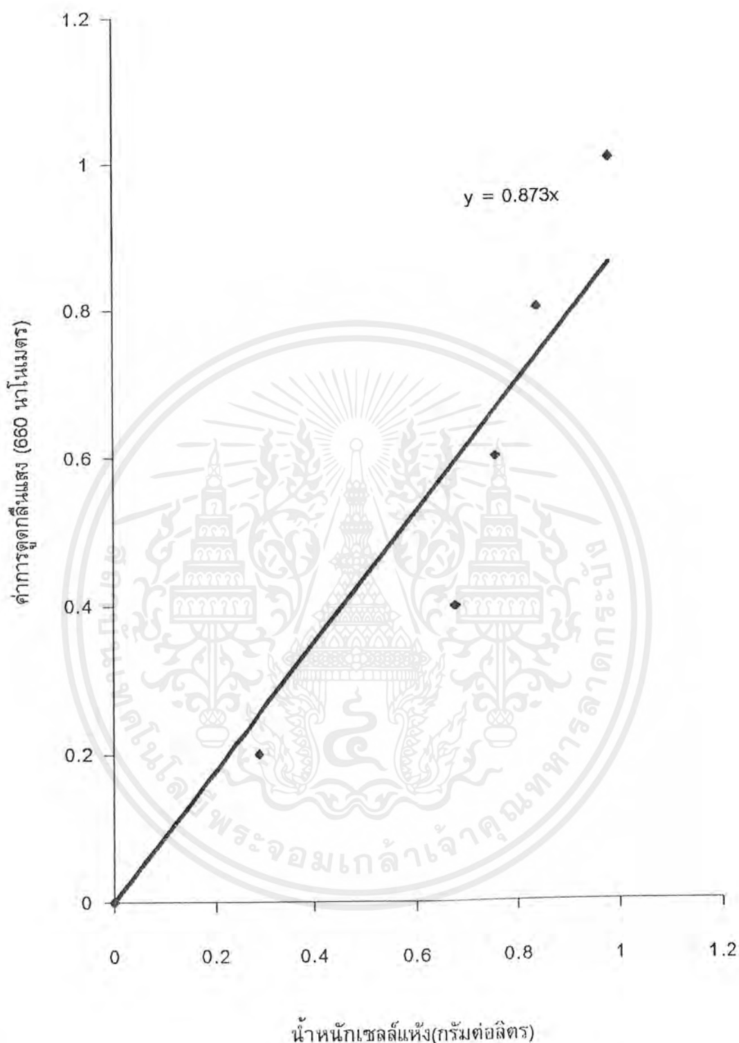
รูปภาคผนวกที่ ค-8 กราฟมาตรฐานน้ำหนักเซลล์แห้งของ Candida tropicalis TISTR 5136 ในน้ำทิ้งโรงงานแปรรูปไก่ที่มีชุดโครสเข้มข้นร้อยละ 2
