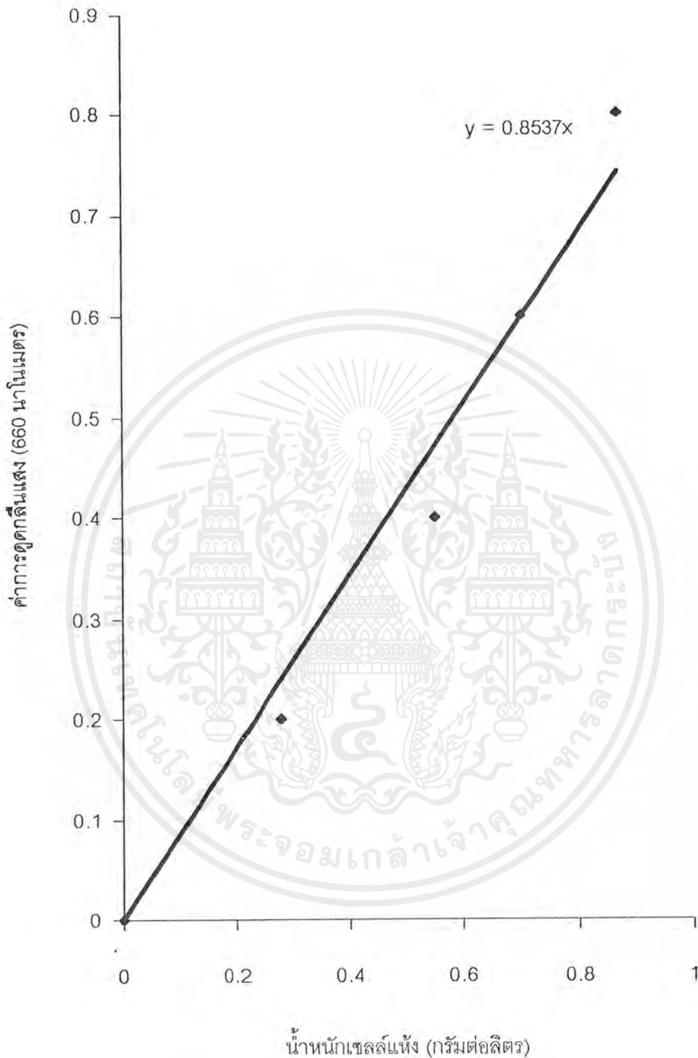
รูปภาคผนวกที่ ค-24 กราฟมาตรฐานน้ำหนักเซลล์แห้งของ Candida tropicalis TISTR 5136 ในน้ำทิ้งโรงงานแปรรูปไก่ ที่มีกลูโคสเข้มข้นร้อยละ 2 กับโพแทสเซียมคลอไรด์เข้มข้นร้อยละ 0.025 และยีสต์สกัดเข้มข้นร้อยละ 0.05
