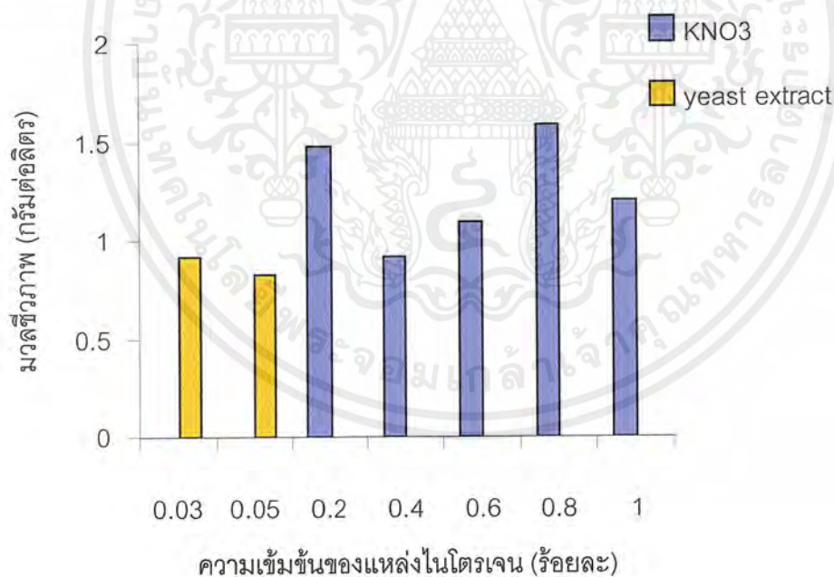
รูปที่ 9 ความสัมพันธ์ระหว่างมวลชีวภาพ ของเชื้อ C. tropicalis TISTR 5136 ในน้ำทิ้งโรงงานแปรรูปไก่ที่มีกลูโคสเข้มข้นร้อยละ 2 โปแทสเซียมคลอไรด์เข้มข้นร้อยละ 0.025 เมื่อมีแหล่งไนโตรเจนที่ความเข้มข้นแตกต่างกัน
