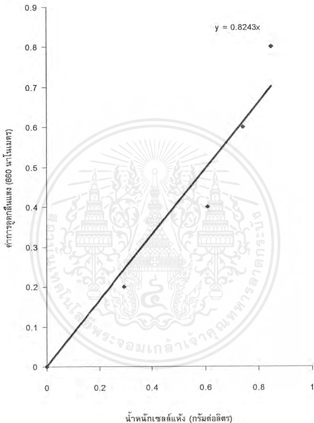
รูปภาคผนวกที่ ค-12 กราฟมาตรฐานน้ำหมักเชสต์แห้งของ Candida tropicalis TISTR 5136 ในน้ำทิ้งโรงงานแปรรูปไก่ที่มีกลูโคสเข้มข้นร้อยละ 2 กับกรดฟอสฟอริกเข้มข้นร้อยละ 0.04
