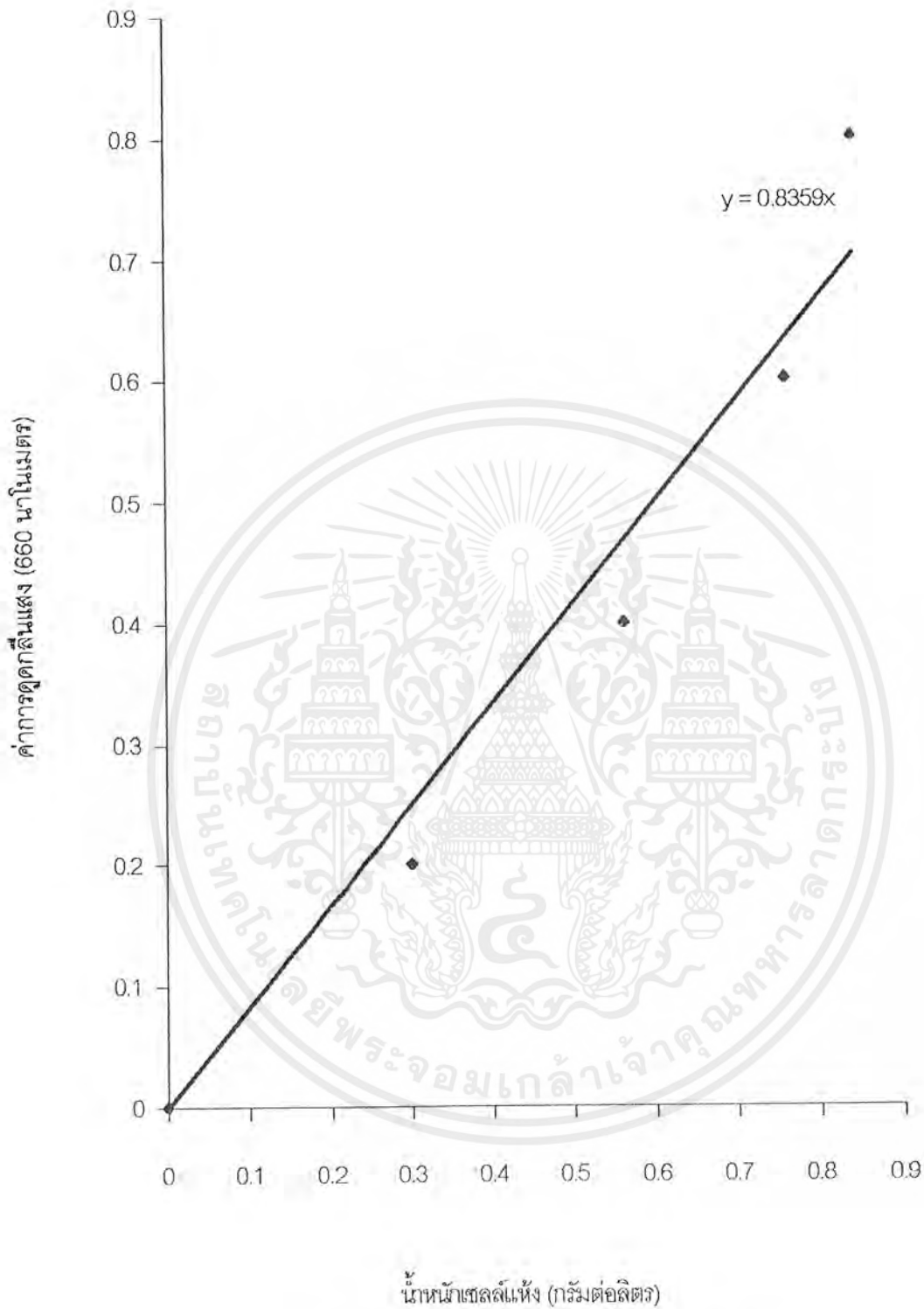
รูปภาคผนวกที่ ก-11 กราฟมาตรฐานน้ำหนักเซลล์แห้งของ Candida tropicalis TISTR 5136 ในน้ำทิ้งโรงงานแปรรูปไก่ที่มีกลูโคสเข้มข้นร้อยละ 2 กับกรดฟอสฟอริกเข้มข้นร้อยละ 0
