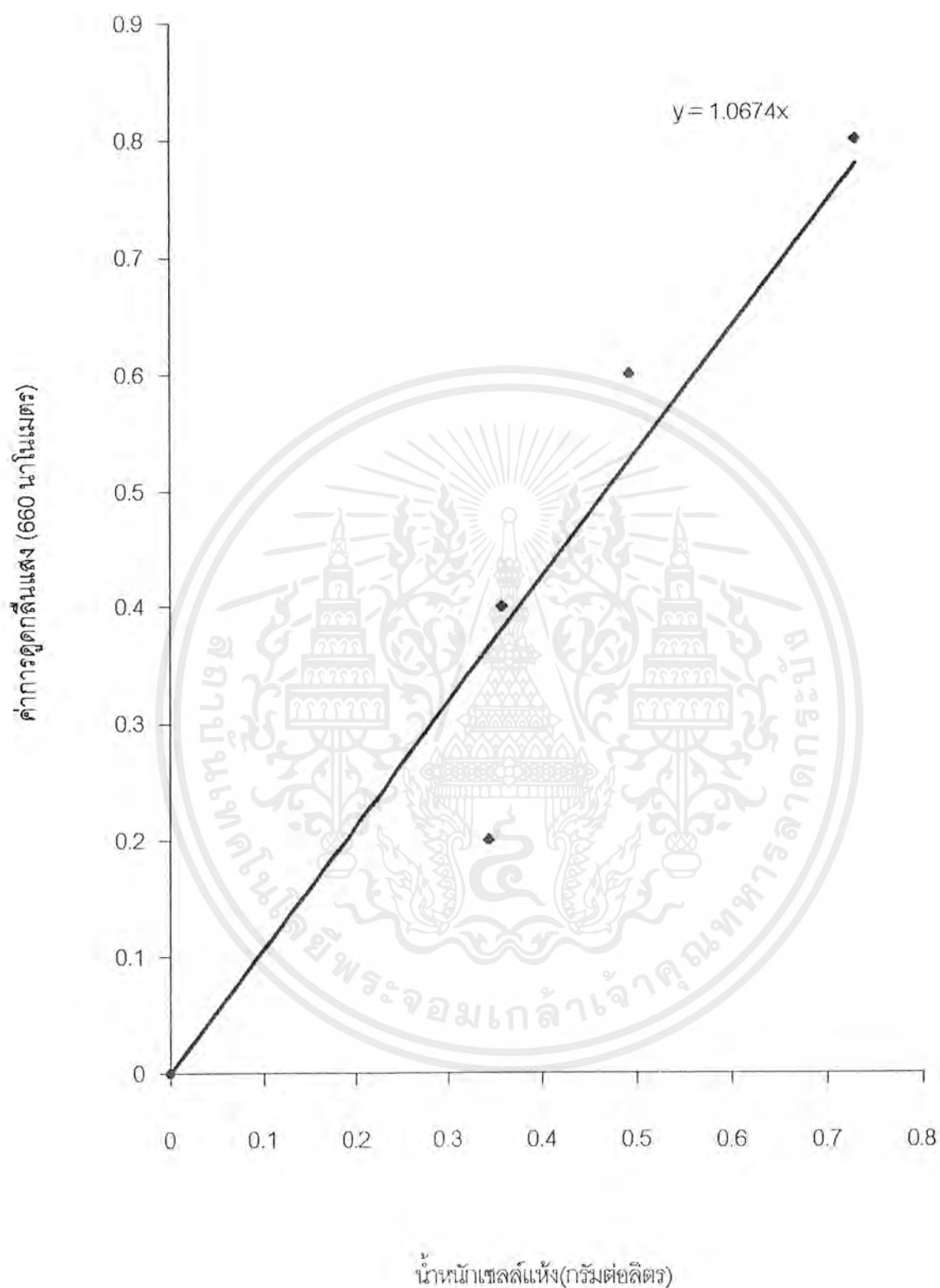
รูปภาคผนวกที่ ค-7 กราฟมาตรฐานน้ำหมักเซลล์แห้งของ Candida tropicalis TISTR 5136 ในน้ำทิ้งโรงงานแปรรูปไก่ที่มีซูโครสเข้มข้นร้อยละ 1
