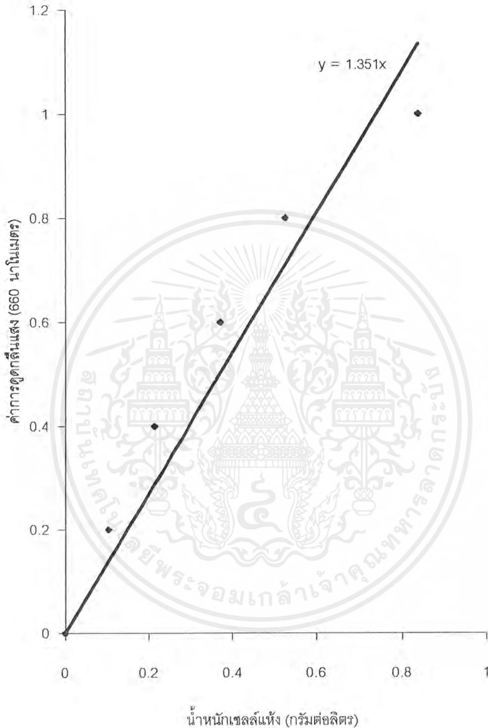
รูปภาคผนวกที่ ค-22 กราฟมาตรฐานน้ำหนักเซลล์แห้งของ Candida tropicalis TISTR 5136 ในน้ำทิ้งโรงงานแปรรูปไก่ ที่มีกลูโคสเข้มข้นร้อยละ 2 กับโพแทสเซียมคลอไรด์เข้มข้นร้อยละ 0.025 และโพแทสเซียมไนเตรดเข้มข้นร้อยละ 1.0
