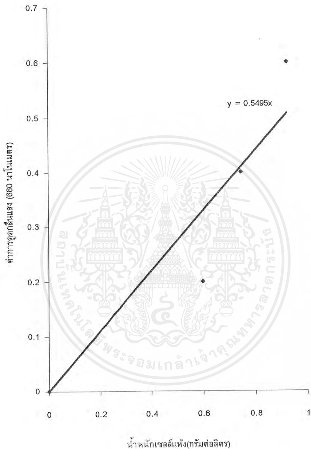
รูปภาคผนวกที่ ค-9 กราฟมาตรฐานน้ำหนักเซลล์แห้งของ Candida tropicalis TISTR 5136 ในน้ำที่โรงงานแปรรูปไก่ที่มีซุโครสเข้มข้นร้อยละ 3
