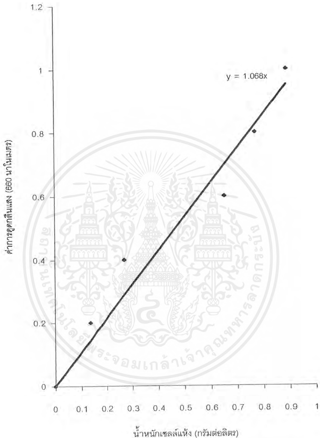
รูปภาคผนวกที่ ค-19 กราฟมาตรฐานน้ำหนักเซลล์แห้งของ Candida tropicalis TISTR 5136 ในน้ำทิ้งโรงงานแปรรูปไก่ ที่มีกลูโคสเข้มข้นร้อยละ 2 กับโพแทสเซียมคลอไรด์เข้มข้นร้อยละ 0.025 และโพแทสเซียมไนเตรตเข้มข้นร้อยละ 0.4
