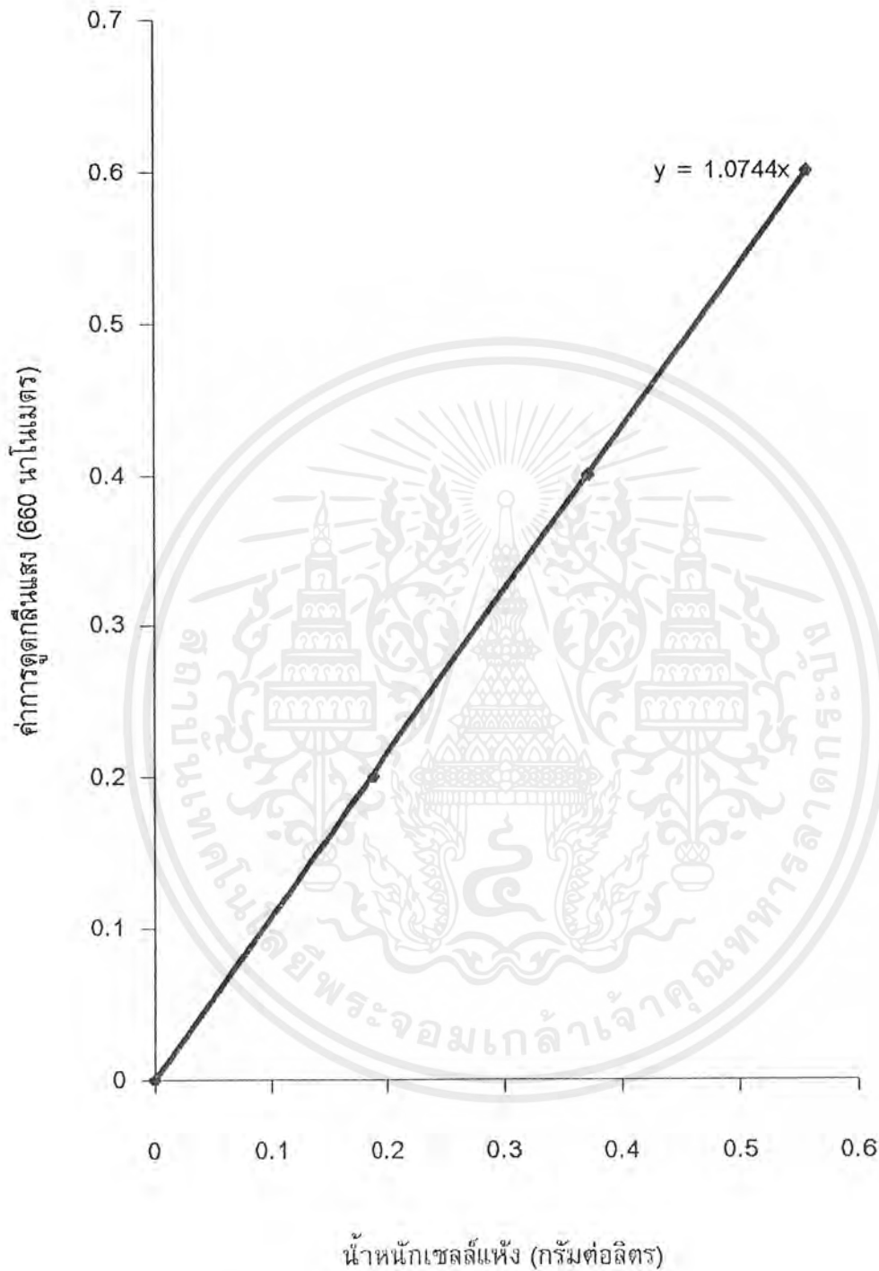
รูปภาคผนวกที่ ค-5 กราฟมาตรฐานน้ำหนักเซลล์แห้งของ Candida tropicalis TISTR 5136 ในน้ำทิ้งโรงงานแปรรูปไก่ที่มีกลูโคสเข้มข้นร้อยละ 3
