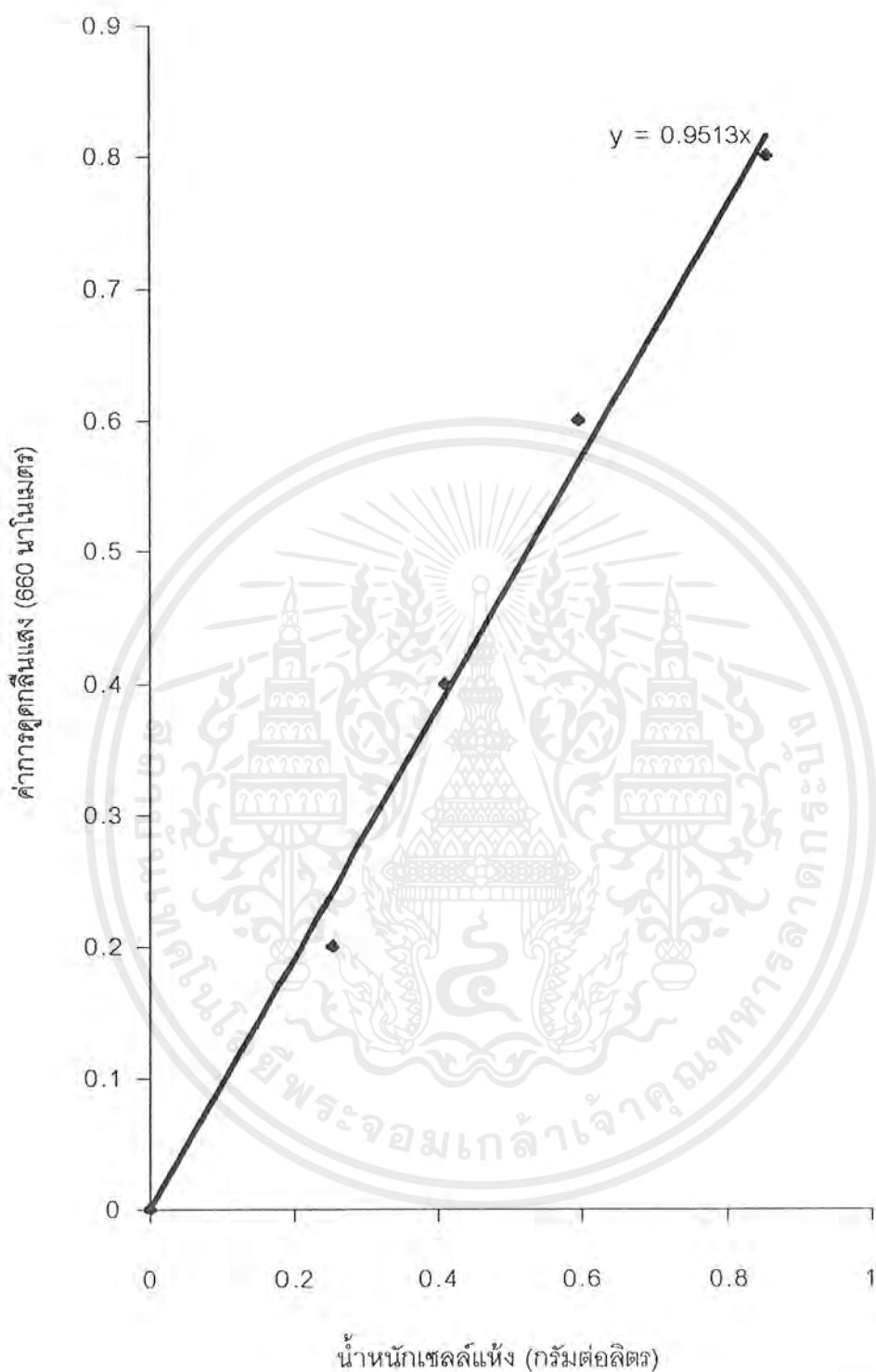
รูปภาคผนวกที่ ค-23 กราฟมาตรฐานน้ำหมักเซลล์แห้งของ Candida tropicalis TISTR 5136 ในน้ำทิ้งโรงงานแปรรูปไก่ ที่มีกลูโคสเข้มข้นร้อยละ 2 กับไพแทลเทียม คลอไรด์เข้มข้นร้อยละ 0.025 และยีสต์สกัดเข้มข้นร้อยละ 0.03
