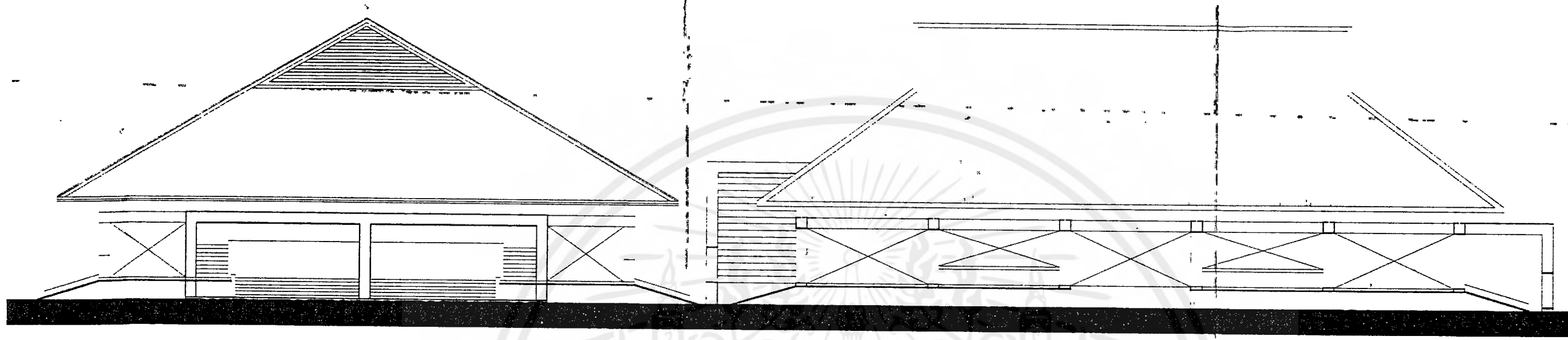
รูปด้านหน้า มาตรฐาน 1 : 125
