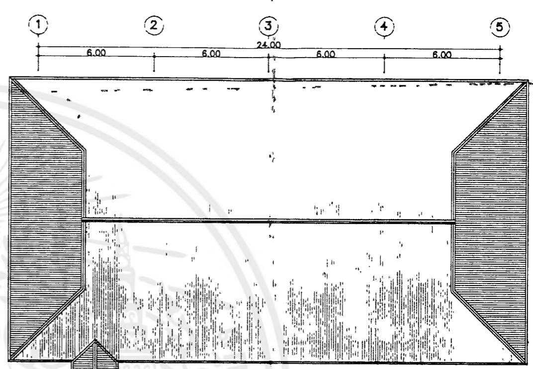
ผังหลังคา มาตรฐาน | 100
