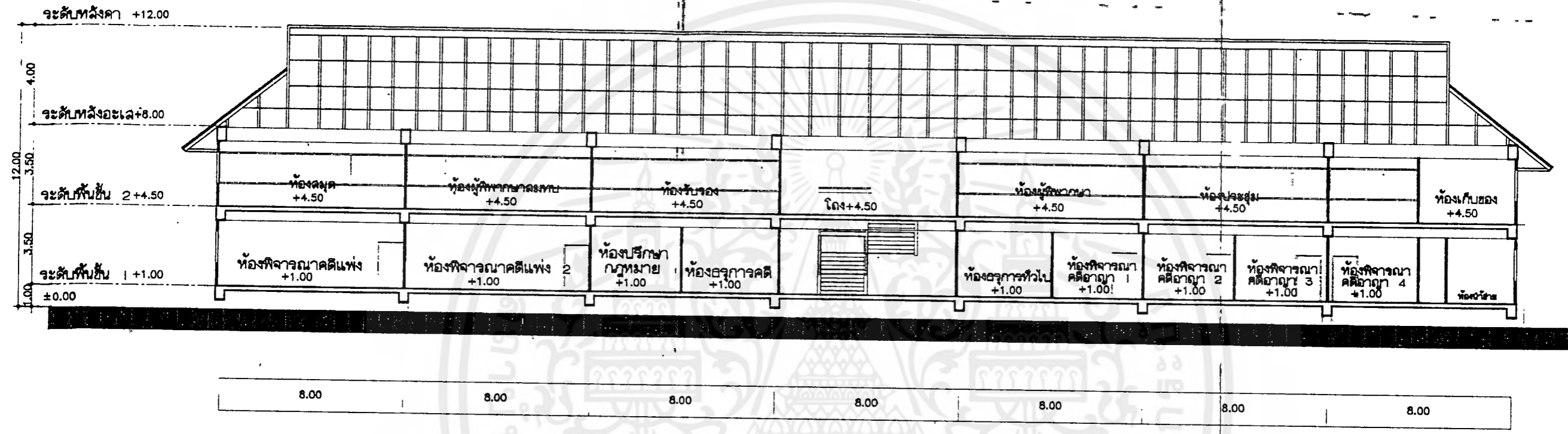
รูปตัดยาว มาตราส่วน 1:200
