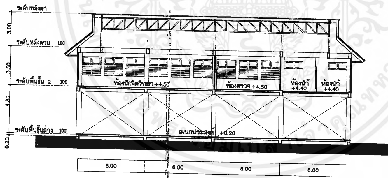
รูปตัด ยาว มาตราส่วน 1:200
