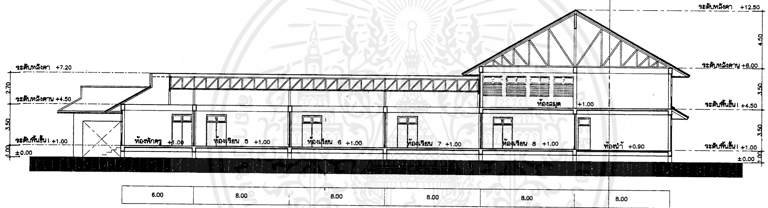
รูปตัด ยาว มาตราส่วน 200
