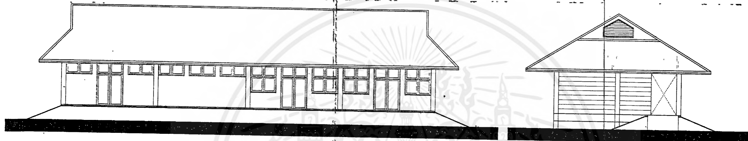
รูปด้านหน้า มาตรฐาน 1 : 150
