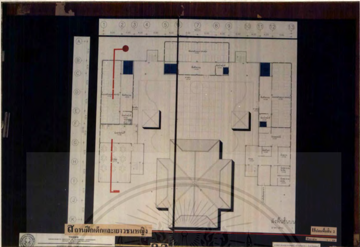
รูปที่ 4.8 1 แสดงแปลนพื้นที่ชั้น 2 สถานฝึกเด็กและเยาวชนหญิง
