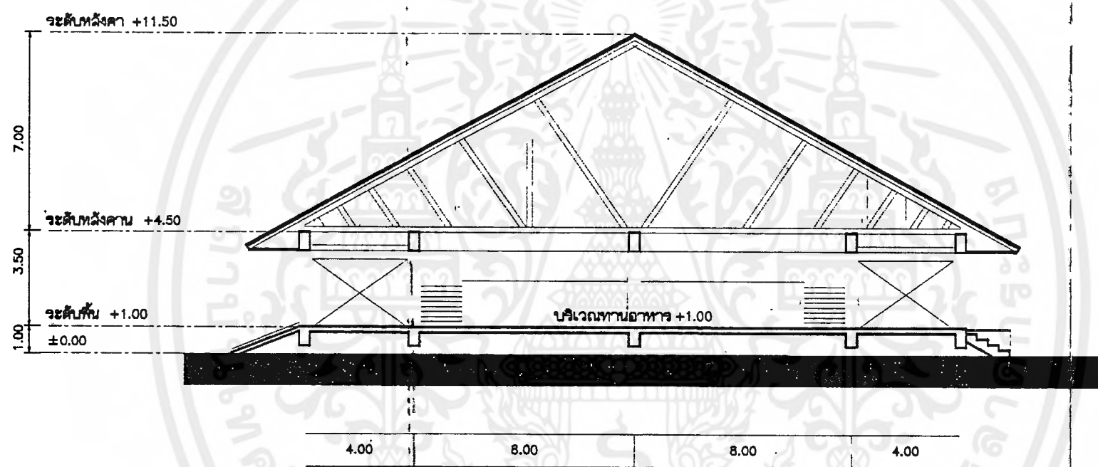
รูปตัด ขวาง มาตราส่วน 1 : 125
