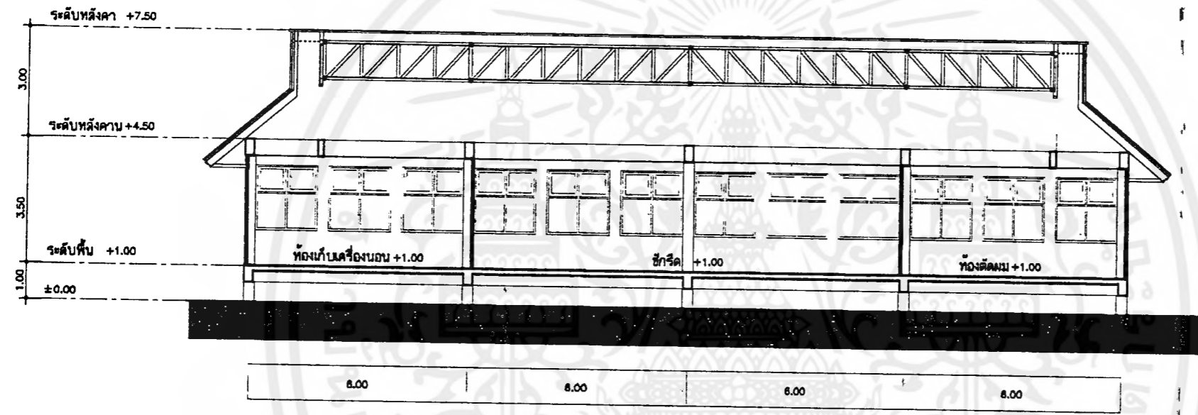
รูปตัด ยาว มาตราส่วน 1 : 150
