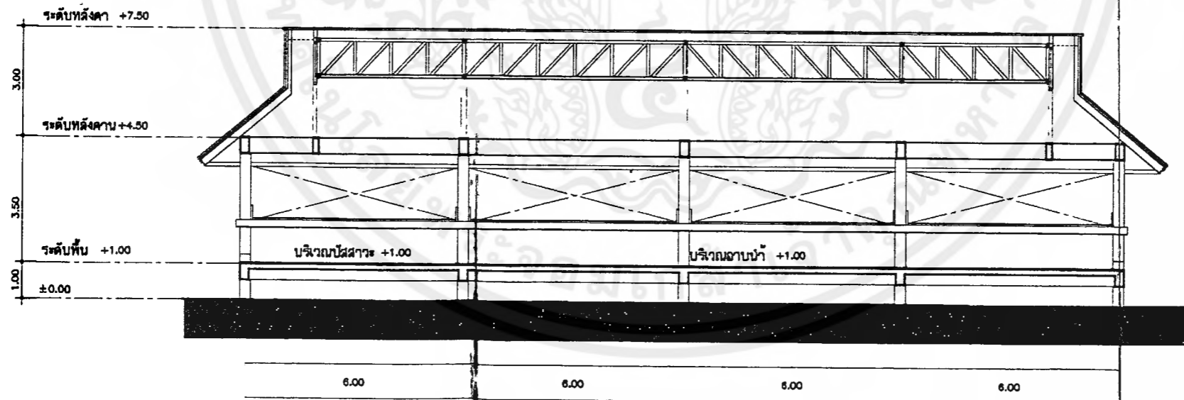
รูปตัด ยาว มาตรฐาน 1 : 150 อานน้ำ ทองสวม
