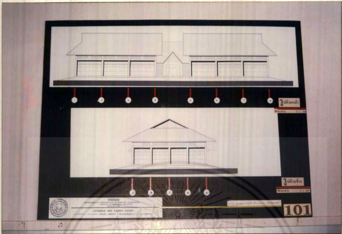
รูปที่ 4.9 5 แสดงรูปด้านหน้า, ด้านข้าง โรงฝึกงานเด็กและเยาวชนชาย
