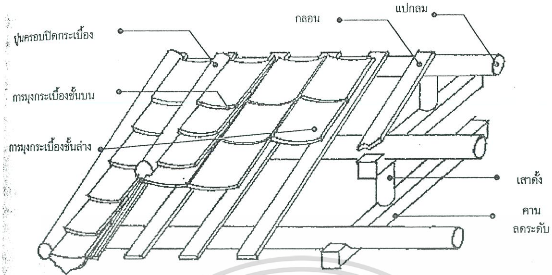
รูปที่ 2.14 แสดงส่วนประกอบของกระเบื้องมุงหลังคา
