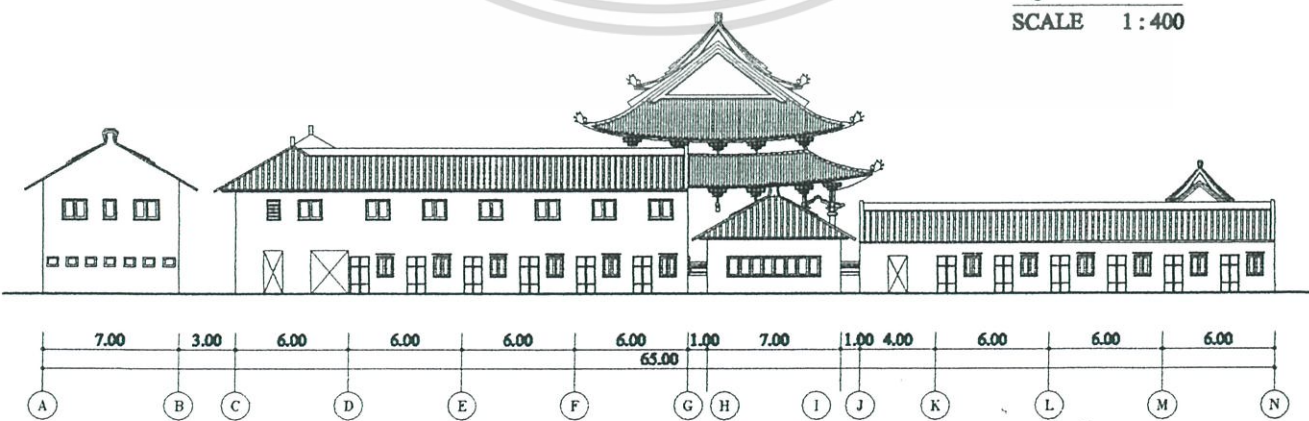
รูปด้าน D SCALE 1:400
