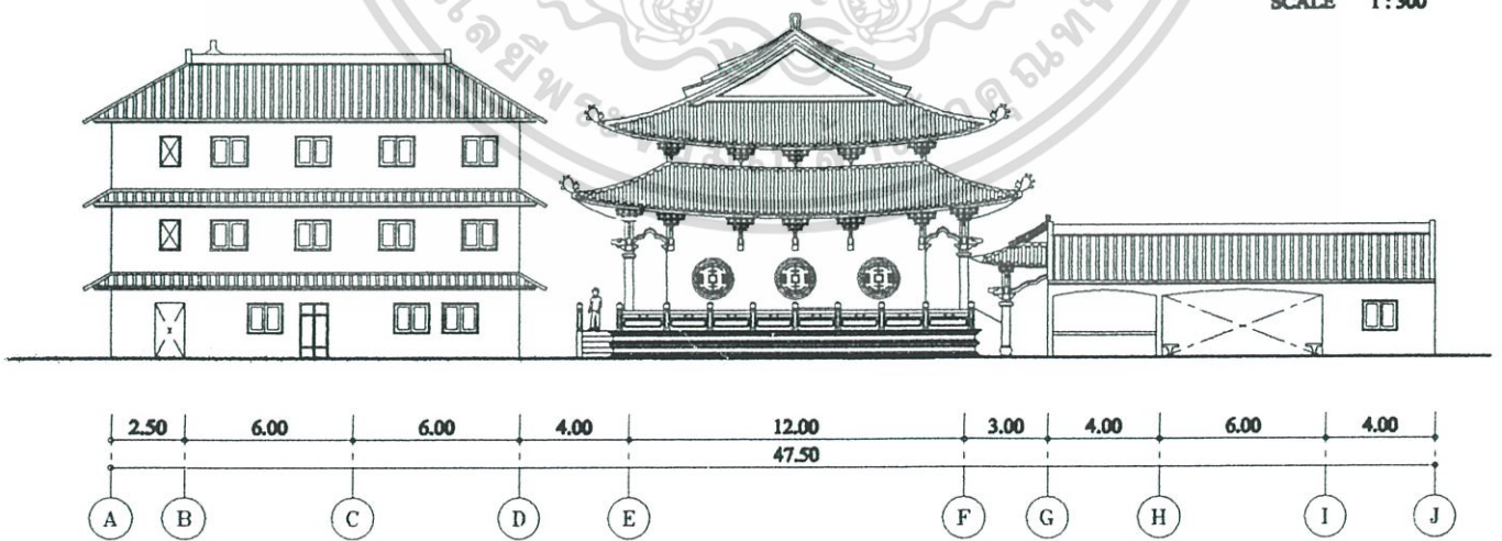
รูปคาน D SCALE 1:300
