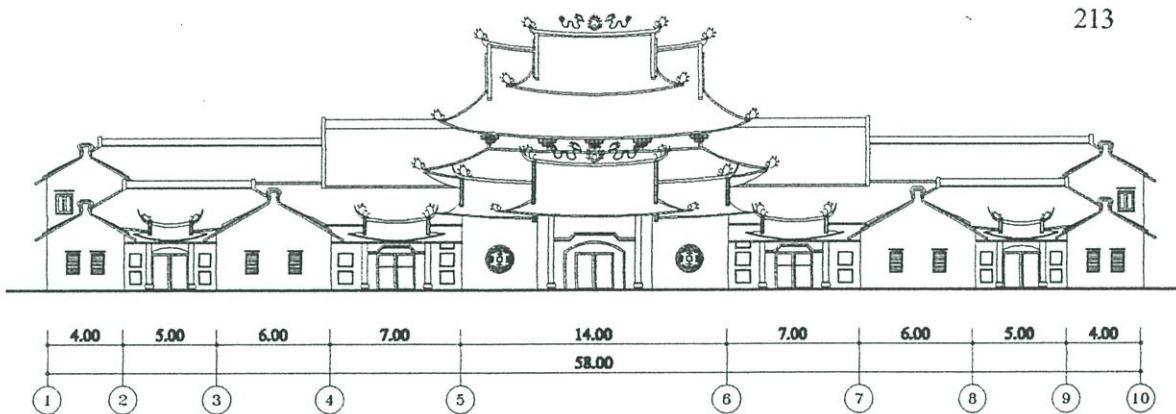
รูปด้าน A SCALE 1:400
