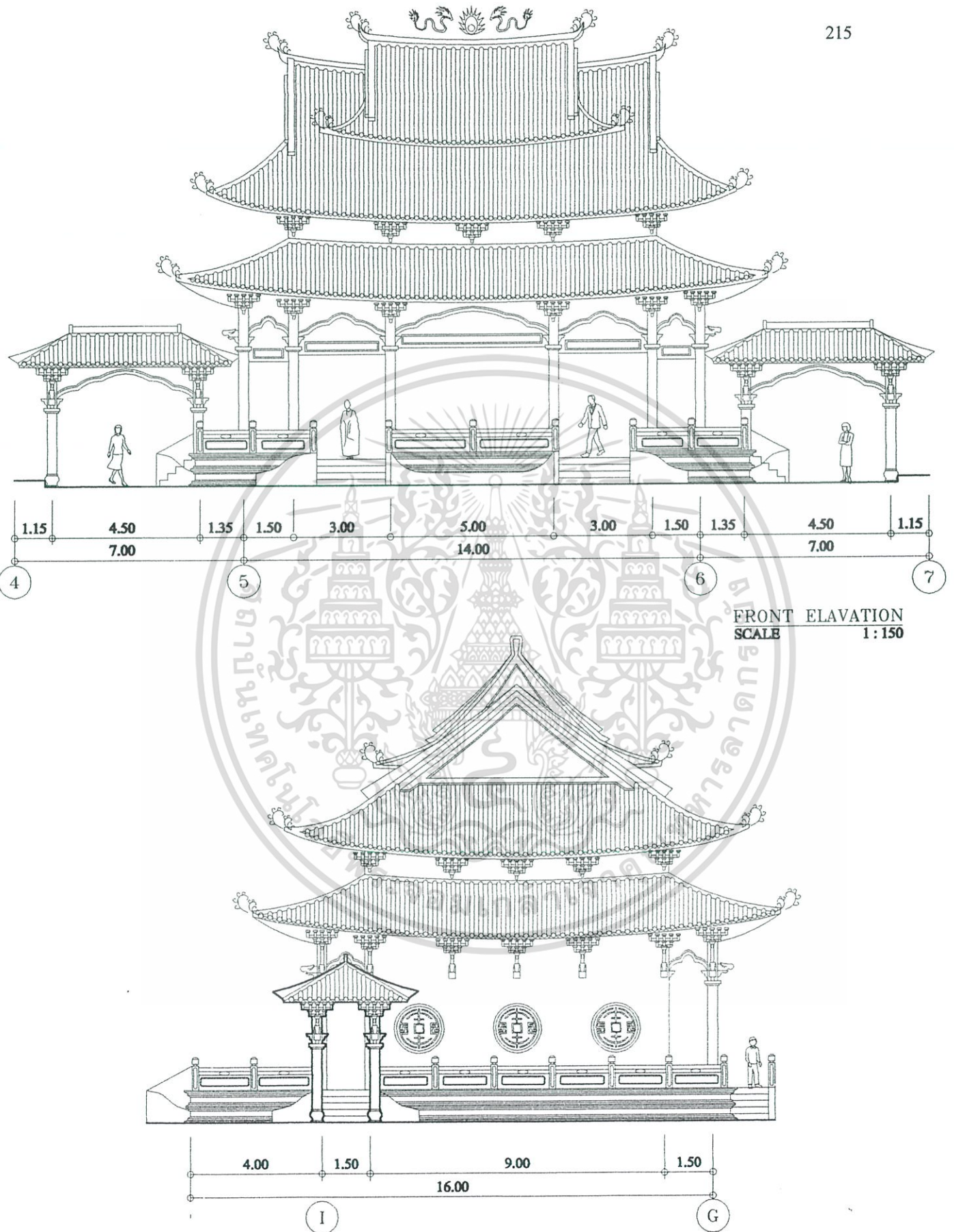
รูปที่ 5.42 แสดงรูปด้านวิหารหลัก (โบสถ์) ของวัดจีนขนาดใหญ่
