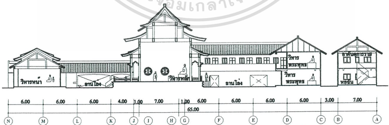
รูปตัด 3 SCALE 1 : 400
