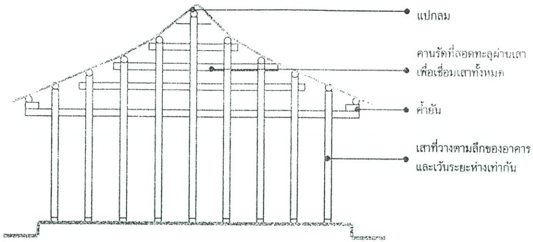
รูปที่ 2.3 แสดงโครงสร้างระบบเสาและคานรัด
