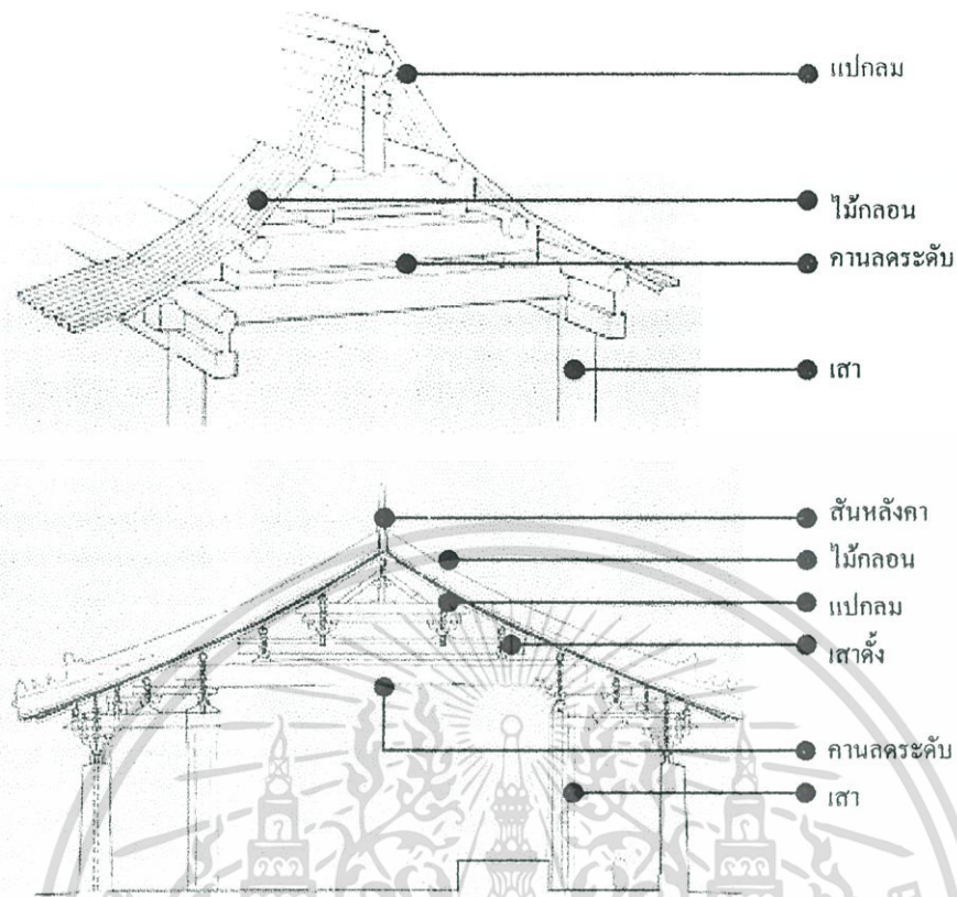
รูปที่ 2.2 แสดงโครงสร้างระบบคานลกระดืบ
