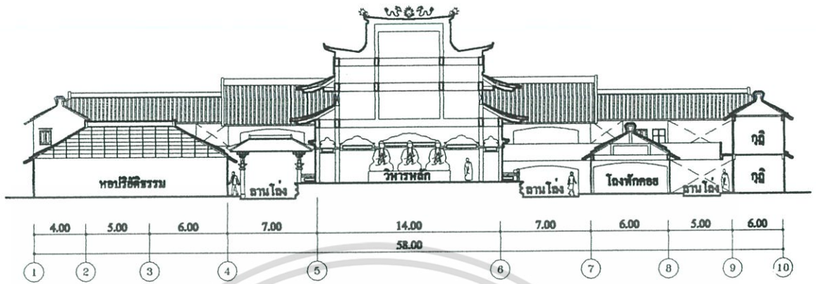
รูปตัด 1 SCALE 1 : 400
