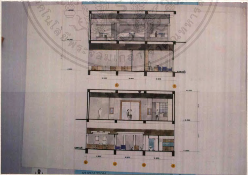
รูปด้าน C - C, D - D
