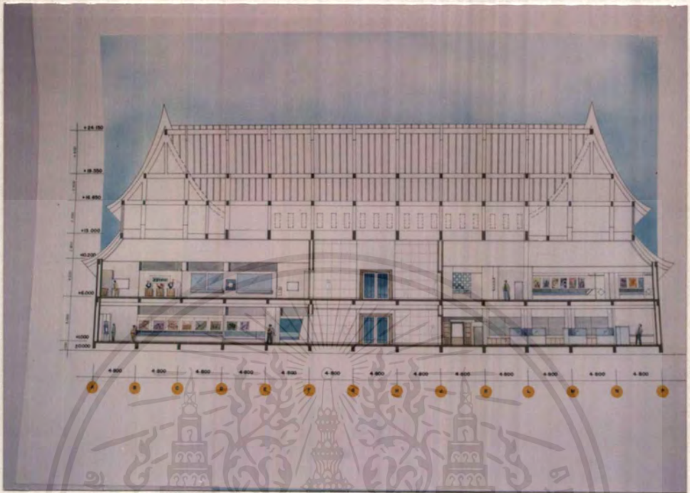
รูปด้าน B - B
