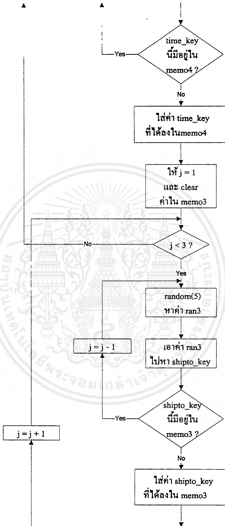
รูปที่ จ-4 แสดง Flow Chart ของโปรแกรมสร้างข้อมูลใน Sale_fact Table
