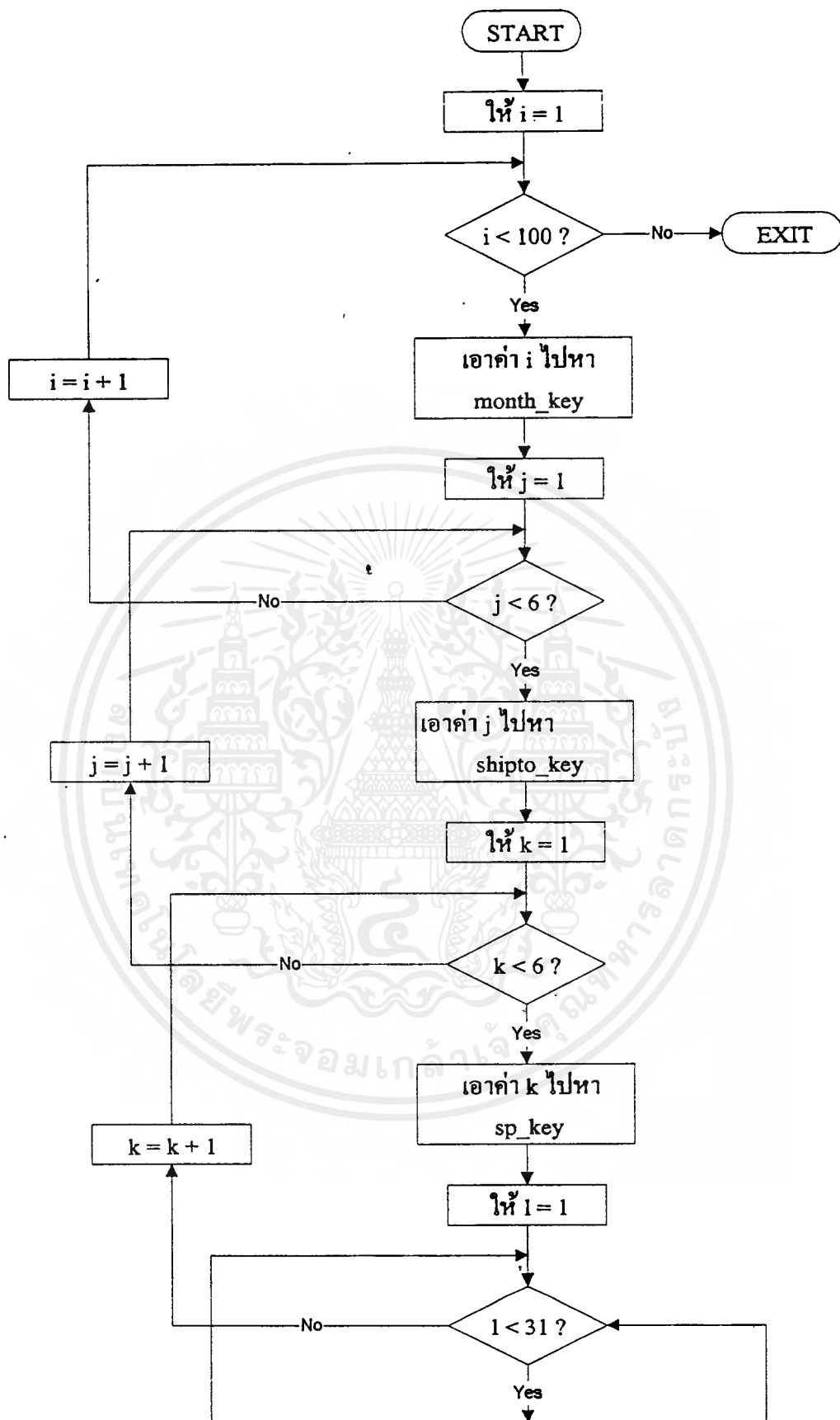
รูปที่ จ-7 แสดง Flow Chart ของโปรแกรมสร้างข้อมูลใน Monthly_fact Table
