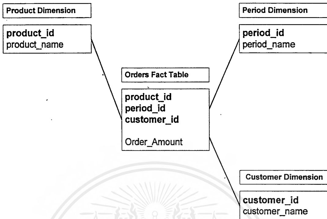
รูปที่ 3-6 แสดง Star Schema ของตัวอย่างการทำ Star Query
