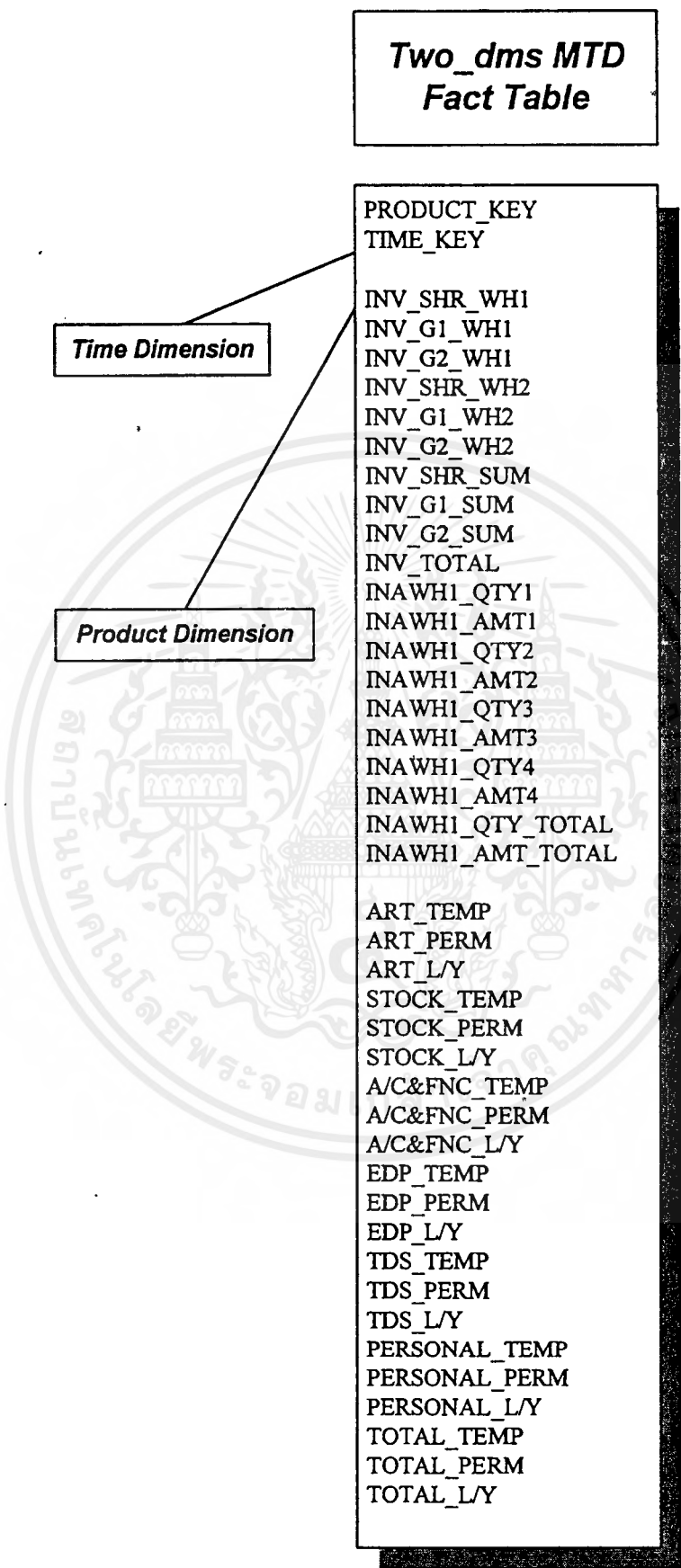
รูปที่ 4-13 แสดง Two Dimension Table ของ MTD
