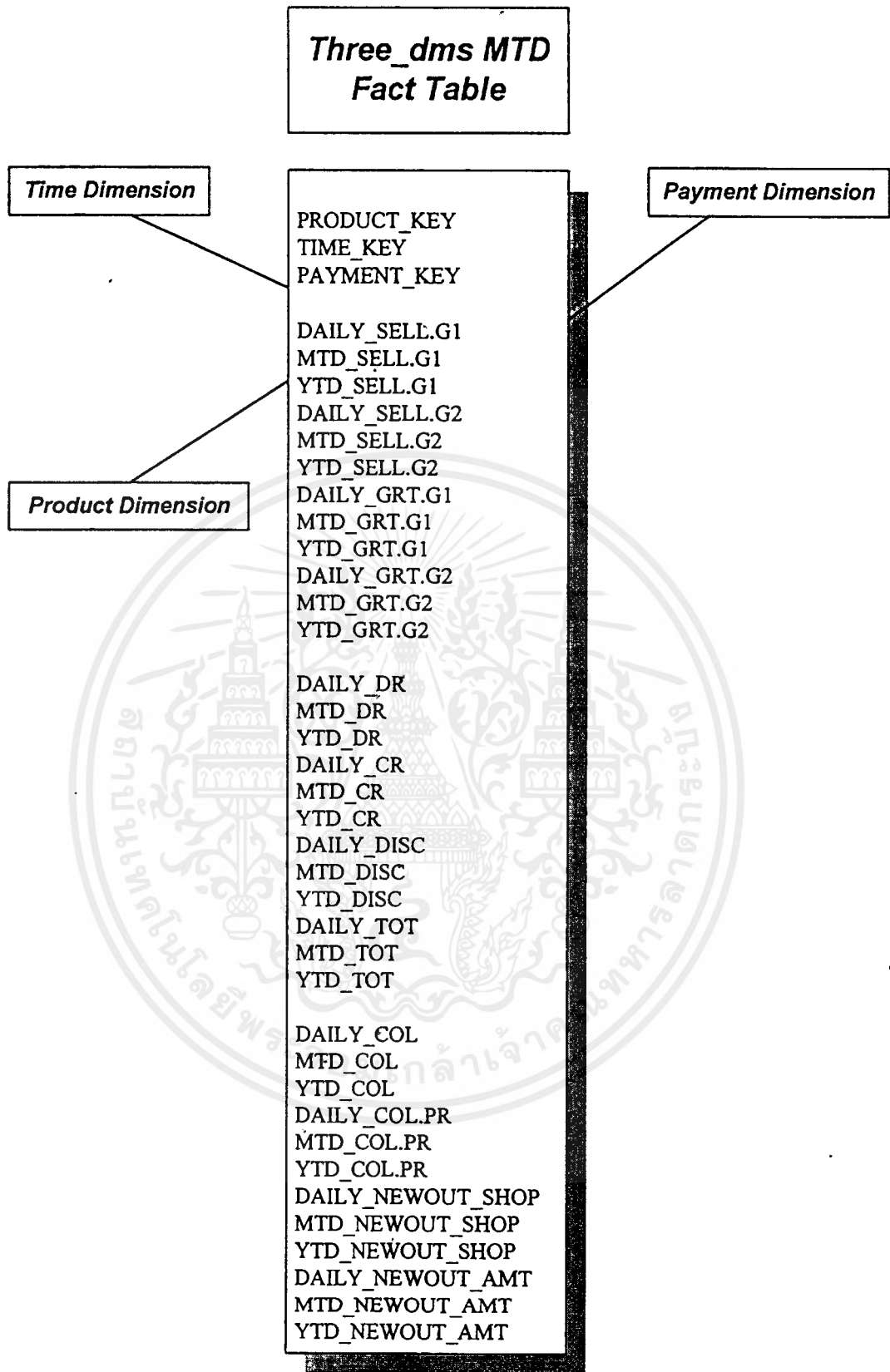
รูปที่ 4-11 แสดง Three Dimension Table ของ MTD
