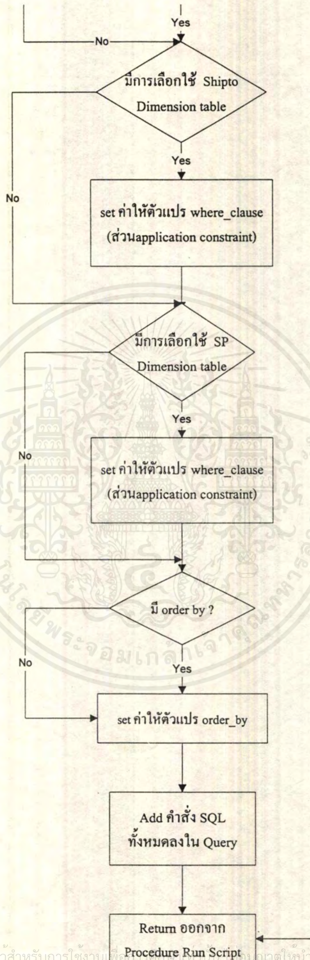
รูปที่ 5.3 แสดง Flow Chart ของ การรับคำสั่งในการ query
