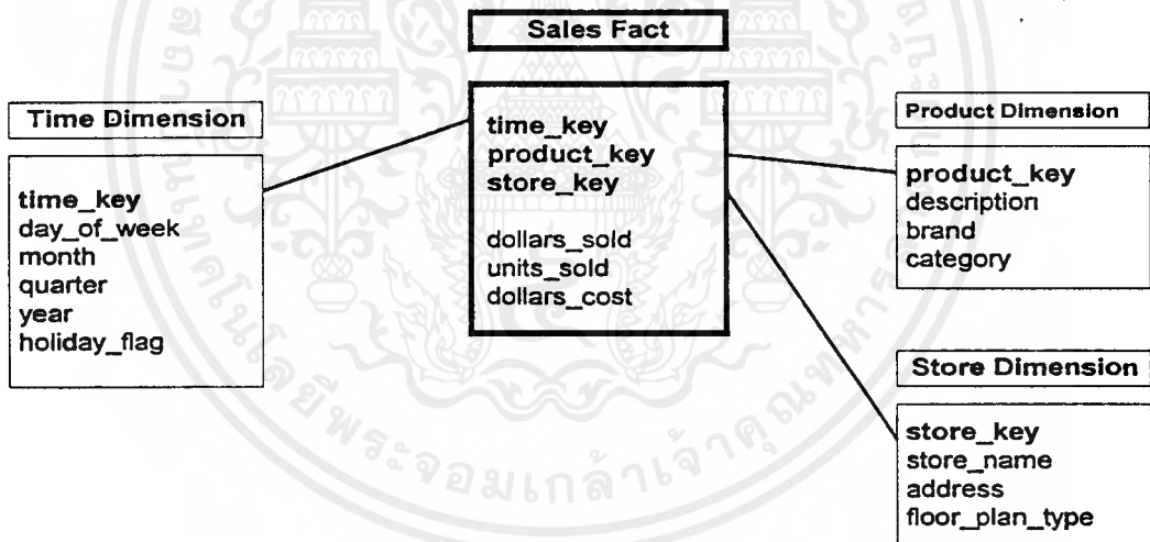
รูปที่ 3-3 แสดงภาพของ STAR JOIN SCHEMA
