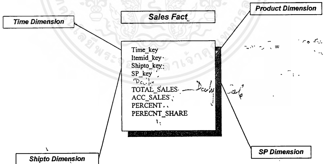
รูปที่ 4-5 แสดง Based_Level Sales Fact Table และ attributes ภายใน table นั้น
