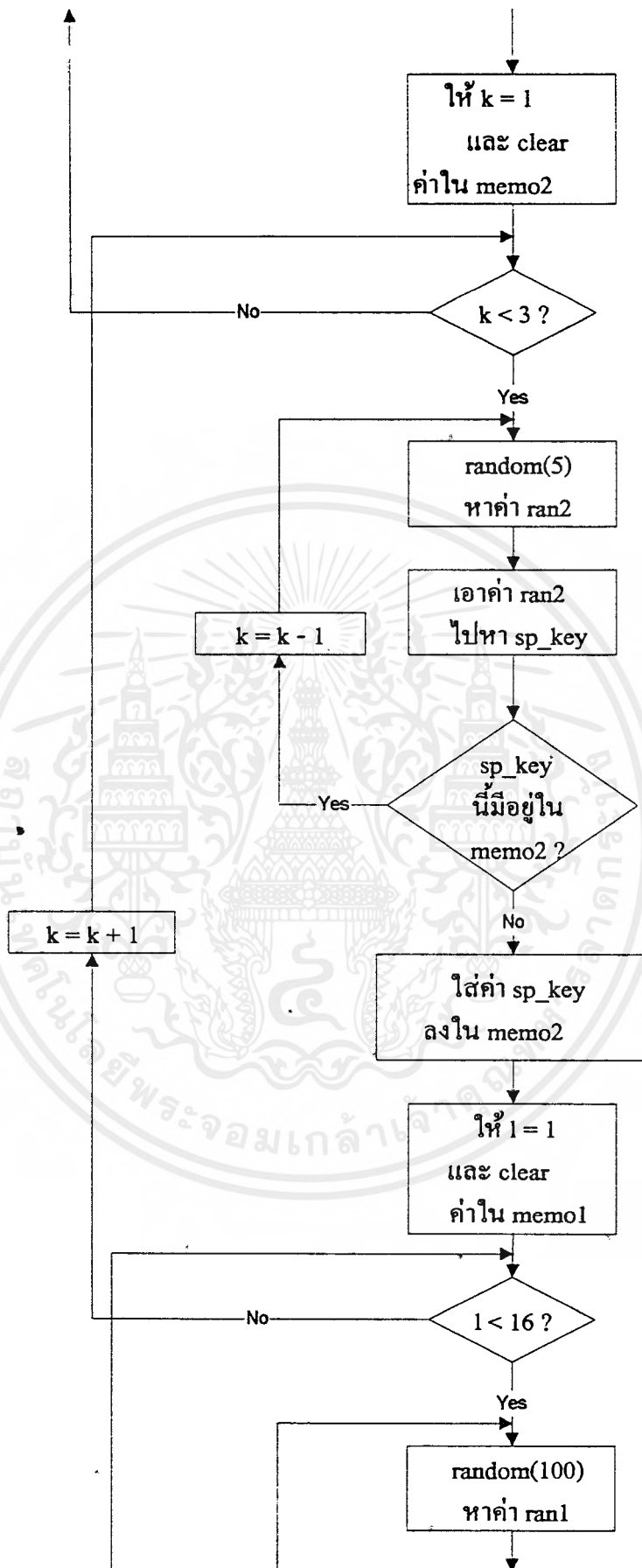
รูปที่ จ-5 แสดง Flow Chart ของโปรแกรมสร้างข้อมูลใน Sale_fact Table
