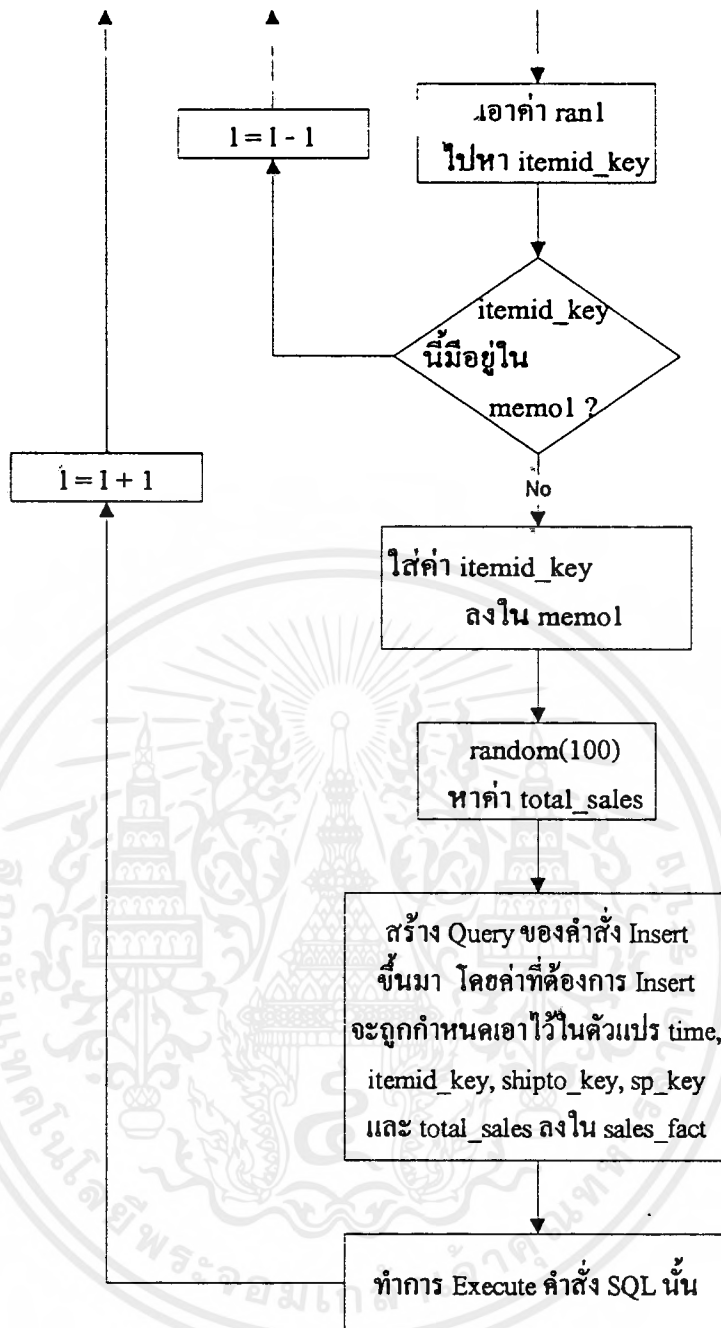
รูปที่ จ-6 แสดง Flow Chart ของโปรแกรมสร้างข้อมูลใน Sale_fact Table
