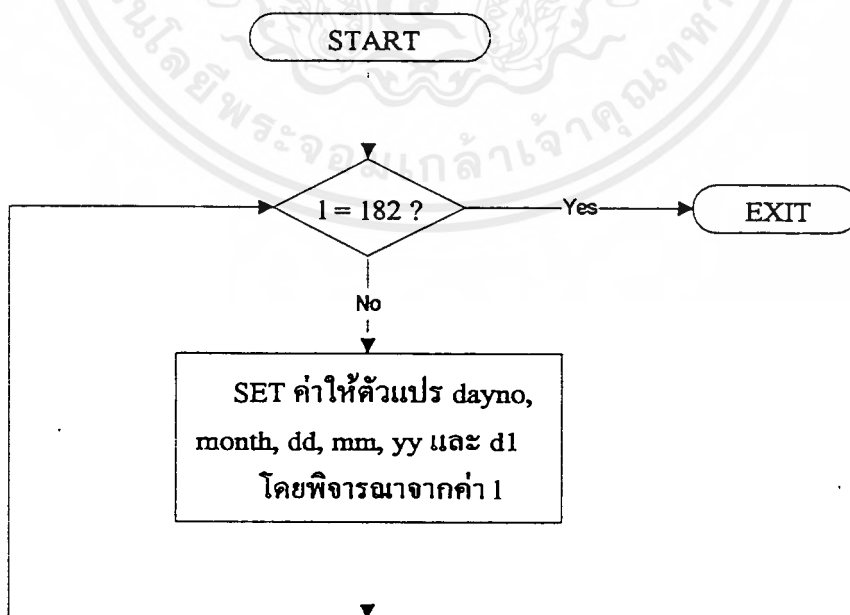
รูปที่ จ-1 แสดง Flow Chart ของโปรแกรมสร้างข้อมูลใน Time Dimension Table
