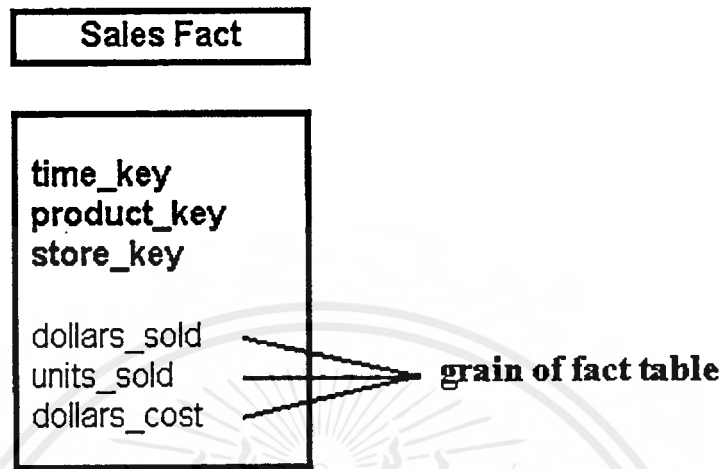
รูปที่ 3-4 แสดง Fact Table และ grain of fact table
