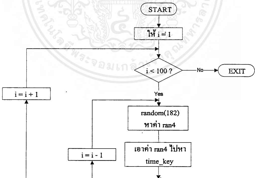
รูปที่ จ-3 แสดง Flow Chart ของโปรแกรมสร้างข้อมูลใน Sale_fact Table
