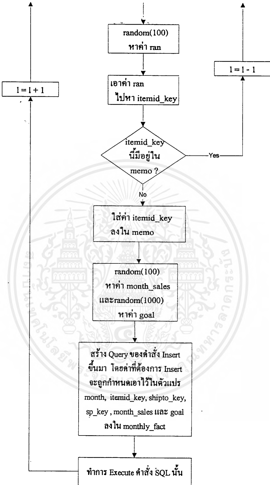
รูปที่ จ-8 แสดง Flow Chart ของโปรแกรมสร้างข้อมูลใน Monthly_fact Table
