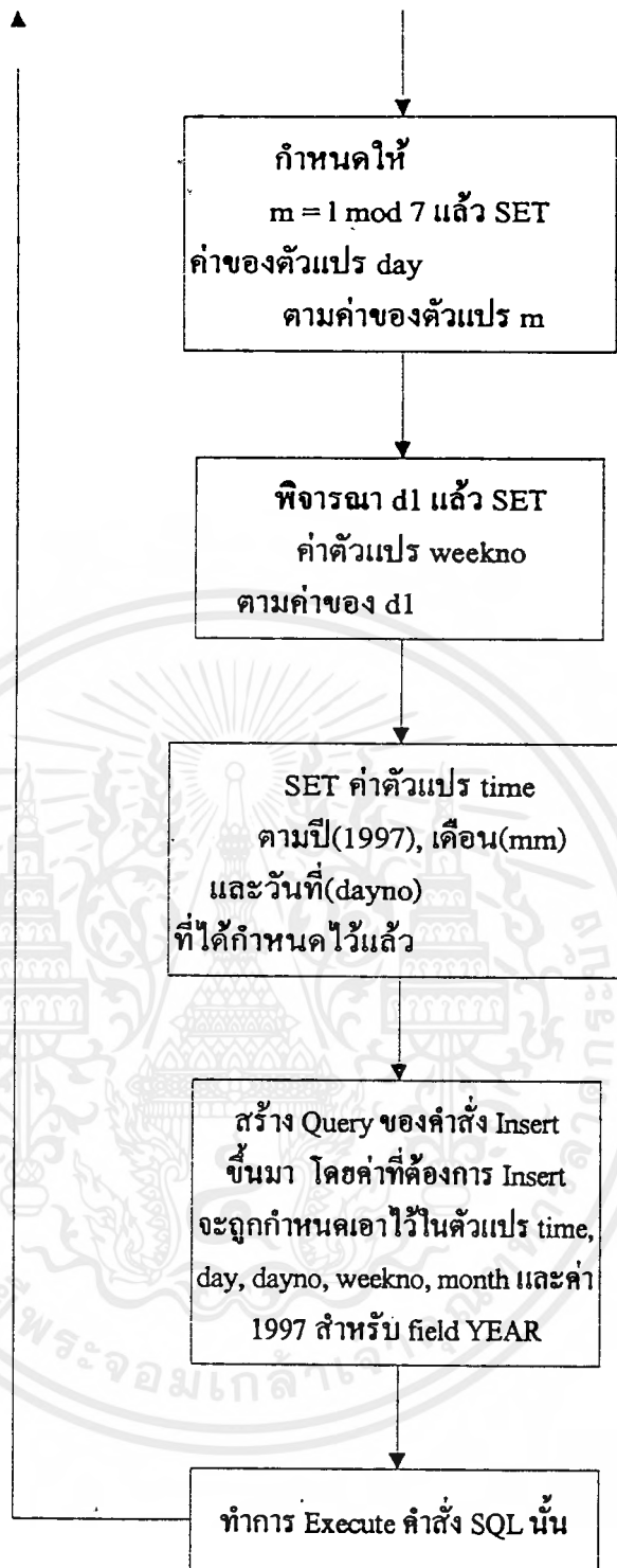
รูปที่ จ-2 แสดง Flow Chart ของโปรแกรมสร้างข้อมูลใน Time Dimension Table
